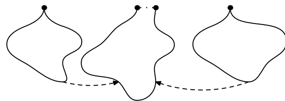
Fig. 3.11: Placement horizontal des sous-arbres : mise à jour des liens (2)
