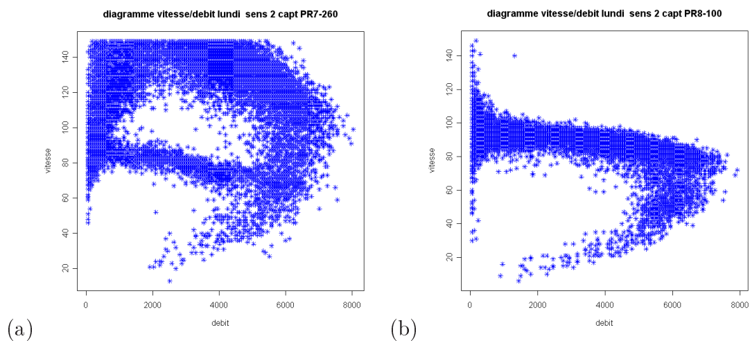
Figure 2.8 – Relation vitesse/débit pour deux capteurs différents, jour similaire, données CORALY . (a) Anomalies apparentes avec vitesses excessives et (b) Profil normal.
