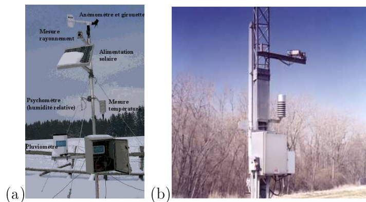
Figure 1.4 – (a) Station météorologique standard. (b) Station météo-routière. [106].
