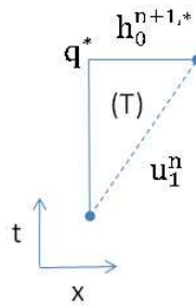
Figure 4.3 – Quantités connues à la fin de l'étape Lagrange.
