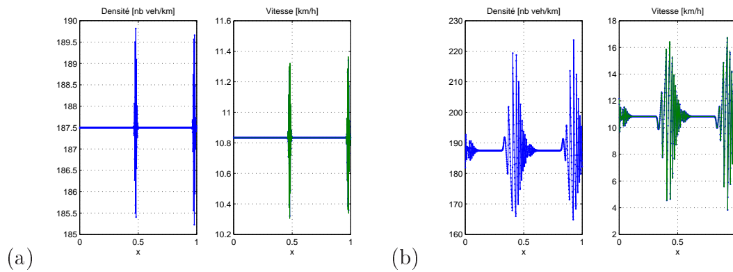
Figure 4.6 – Croissance des instabilités linéaires dans la région dense pour \alpha = 0 et \rho_0 = \frac{1}{2}\rho_M . Profils de densité et vitesse moyenne, (a) au temps t = 0.002 et (b) au temps t = 0.1 .
