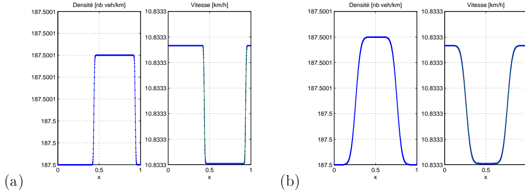
Figure 4.7 – Absence d’instabilités linéaires pour une grande valeur de \rho_0 . Profils de densités et vitesses moyennes, (a) au temps t = 0.002 et (b) au temps t = 0.1 .
