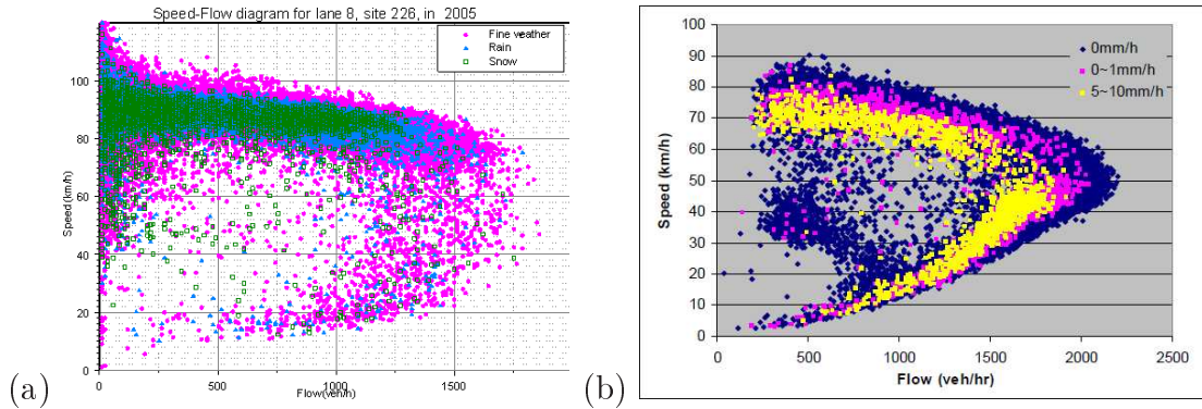
Figure 1.11 – Relation vitesse/débit pour différentes intensités de précipitation. (a) Projet INTRO [78] et (b) données japonaises du réseau MEX [26].
