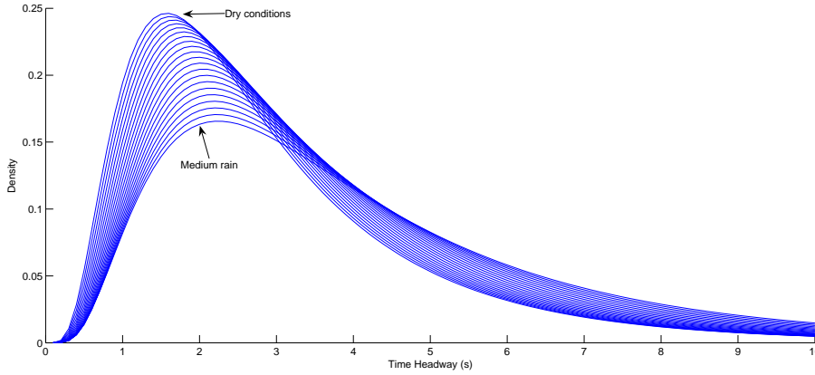
Figure 3.7 – Paramétrage de la distribution des temps inter-véhiculaires.
