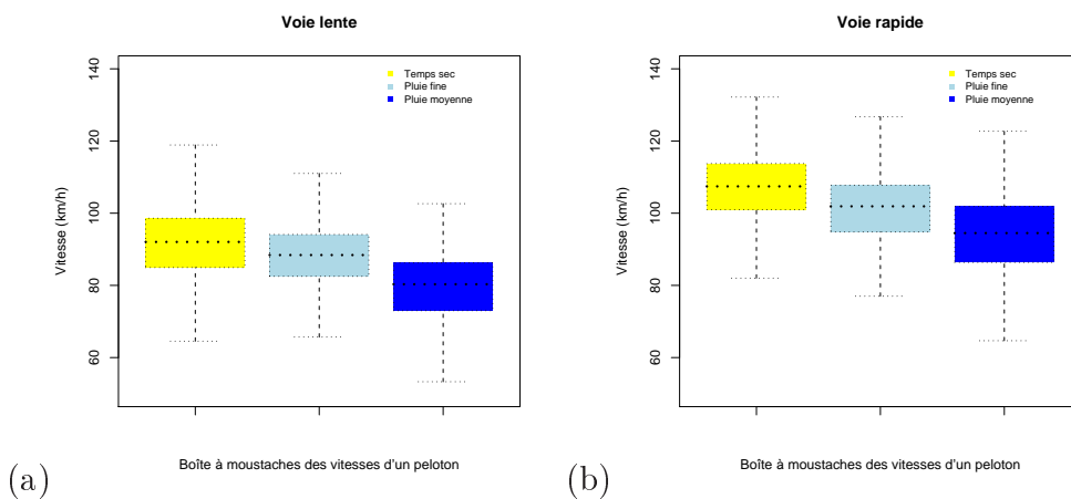
Figure 2.24 – Boîtes à moustaches des vitesses moyennes spatiales des pelotons. Données RN118. (a) voie lente et (b) voie rapide.
