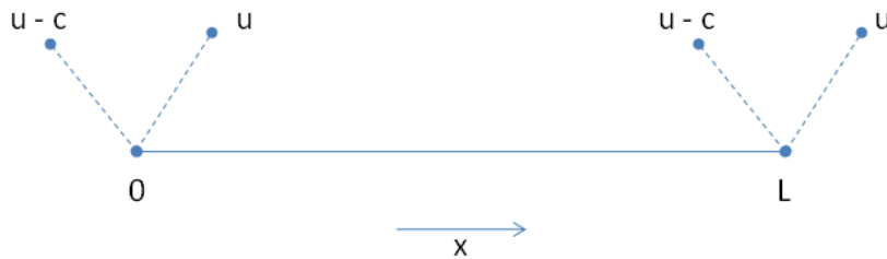
Figure 4.2 – Nature des solutions aux interfaces avec \rho_0 \geq \rho
