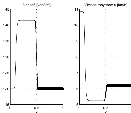
Figure 4.23 – Terme de relaxation faible : profils de densités et vitesses au temps t = 0.015 .
