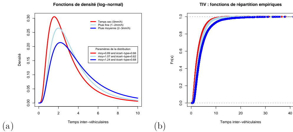
Figure 2.21 – Modélisation des temps inter-véhiculaires sur la RN118 par une loi log-normale, voie lente. (a) fonctions de densité et (b) fonctions de répartition.
