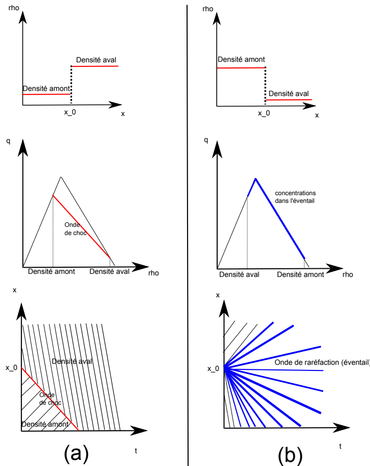
Figure 3.3 – Modèles LWR et discontinuités. (a) cas d'un trafic fluide rencontrant un trafic dense et (b) cas inverse.
