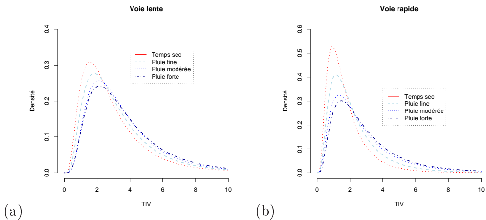
Figure 2.22 – Modélisation log-normale des temps inter-véhiculaires des données suisses (a) voie lente et (b) voie rapide. Données OFROU.
