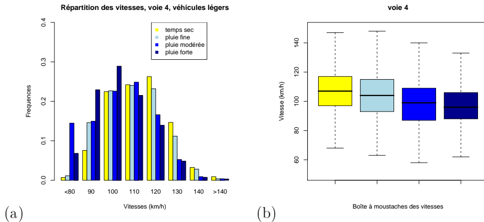
Figure 2.17 – Répartition des vitesses pour les deux directions. (a) histogramme et (b) boîtes à moustaches associées. Données suisses.
