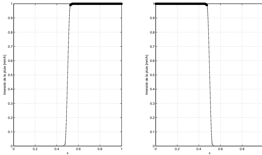
Figure 4.10 – Initialisation d'un créneau de pluie en espace : le front pluvieux est localisé soit sur l'ensemble de la deuxième partie de la section, soit sur la première
