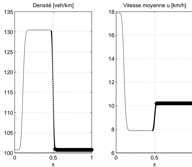
Figure 4.11 – Régime dense : flot de véhicules entrant dans une section pluvieuse. Profils de densités et vitesses moyennes au temps t = 0.015
