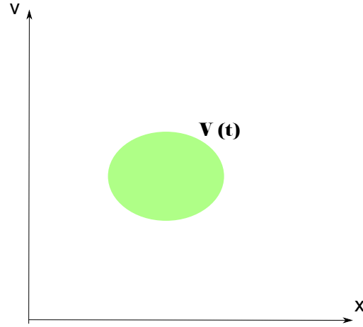
Figure 3.5 – Volume se déplaçant au cours du temps dans l'espace des phases
