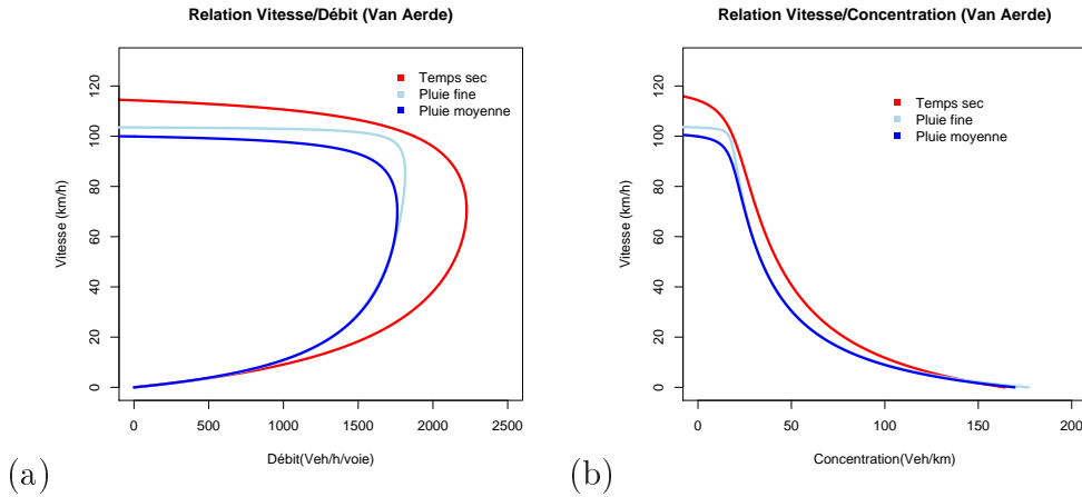
Figure 2.26 – Calibrage du modèle de Van Aerde. Véhicules légers, voie rapide. Données RN118.
