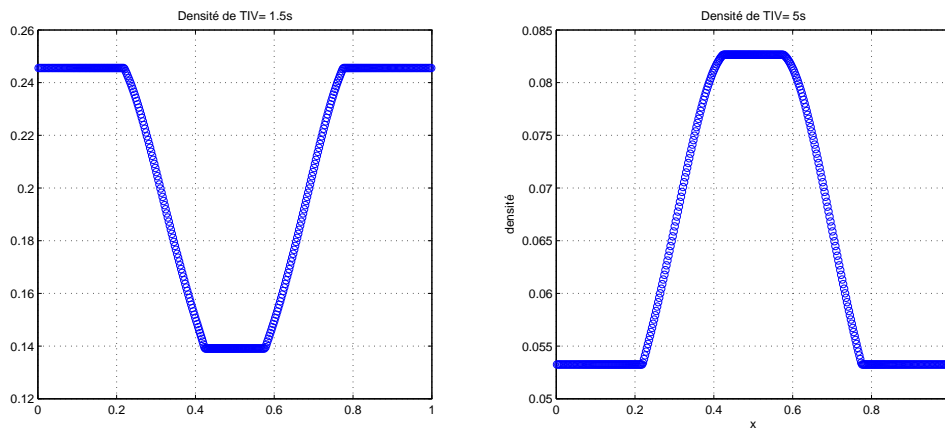
Figure 4.22 – Profils de TIV courts (1.5s) et moyens (5s) sur la section au temps t = 0.015
