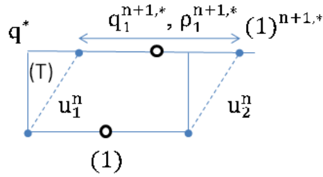
Figure 4.3 – Quantités connues à la fin de l'étape Lagrange.
