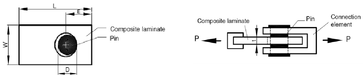
Fig. 3.57 – Paramètres géométriques des assemblages boulonnés [YYL65]
