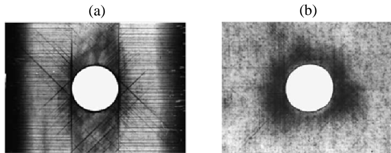
Fig. 2.16 – Radiographies rayons X de stratifiés troués à 95% de la contrainte à rupture [TOU96] : (a) Carbone/époxy – (b) Carbone/PEEK
