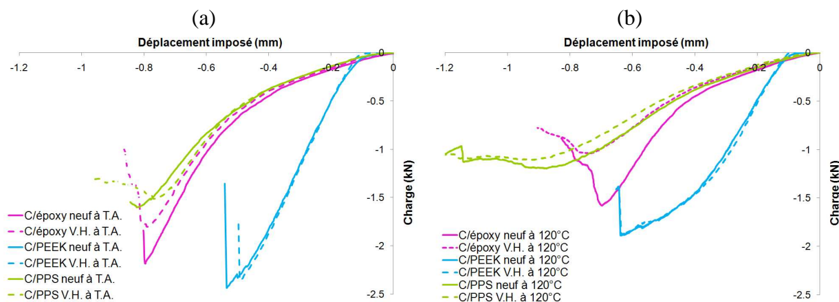
Fig. 3.54 – Influence du V.H. sur la réponse charge-déplacement en Cisaillement InterLaminaire : T.A. – (b) 120°C
