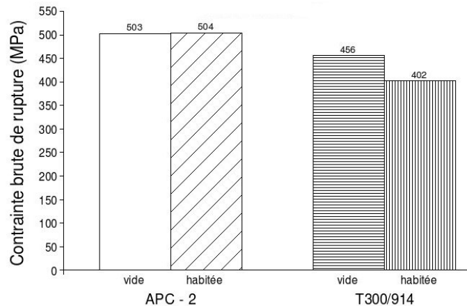
Fig. 3.59 – Influence de la présence d'un boulon sur la traction trouée quasi-isotrope ( \phi_{\text{trou}}=6 mm) [VAU93]
