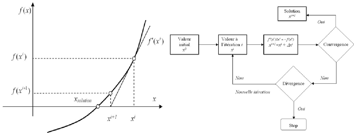
Fig. 4.9 – Méthode de résolution itérative de Newton
