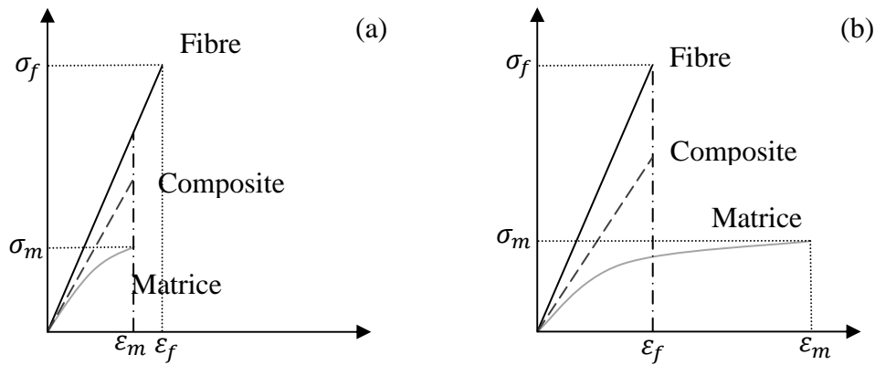
Fig. 1.3 – Courbes schématiques contrainte-déformation des différents constituants d'un composite unidirectionnel sollicité en traction longitudinale : (a) \epsilon_f > \epsilon_m - (b) \epsilon_f < \epsilon_m
