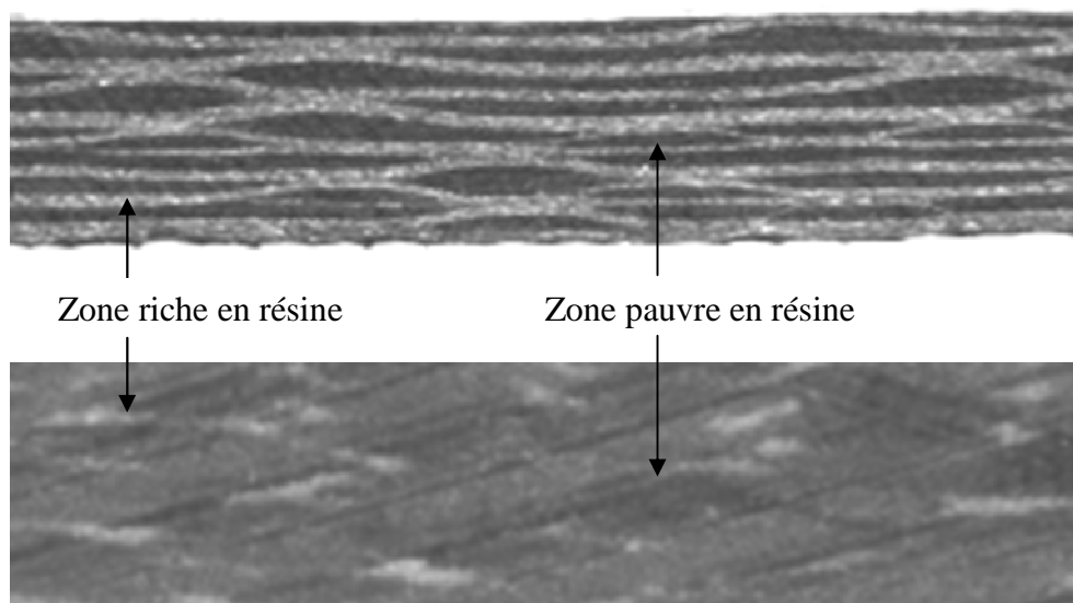
Fig. 3.7 – Coupes dans l'épaisseur de stratifiés tissés quasi-isotrope [0/45/0/45/0/45/0] et à plis orientés [45]_7 - Cas du carbone/PPS
