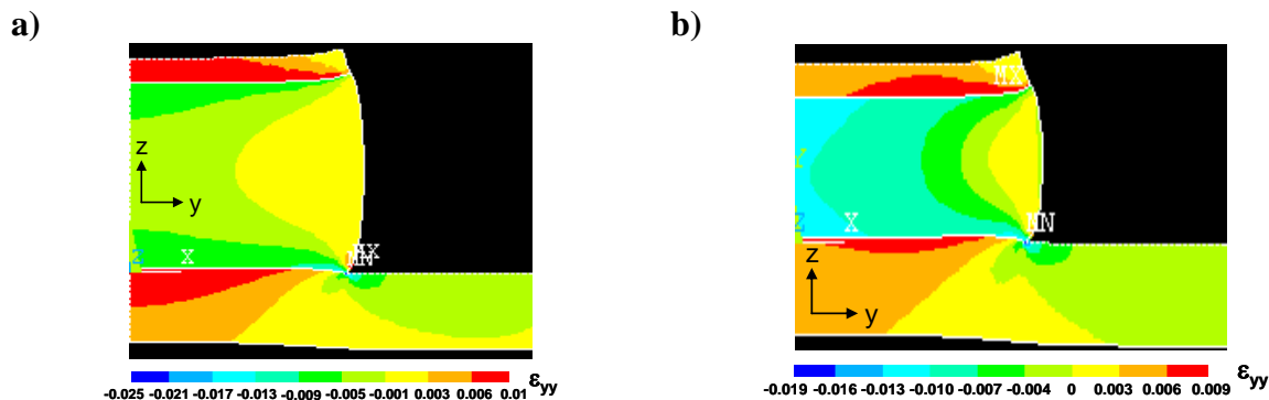
Figure IV.57: Simulations mécaniques par éléments finis 33 de la déformation latérale dans l'empilement Si/SiGe/Si avec une longueur de grille L_g+2L_{sp}=80 nm, un pourcentage en Ge de la couche de SiGe de 40%, une épaisseur de la couche de SOI de 15 nm et de la couche active de Si de 5 nm et des épaisseurs de la couche de SiGe de a) 30 nm et b) 15 nm.
