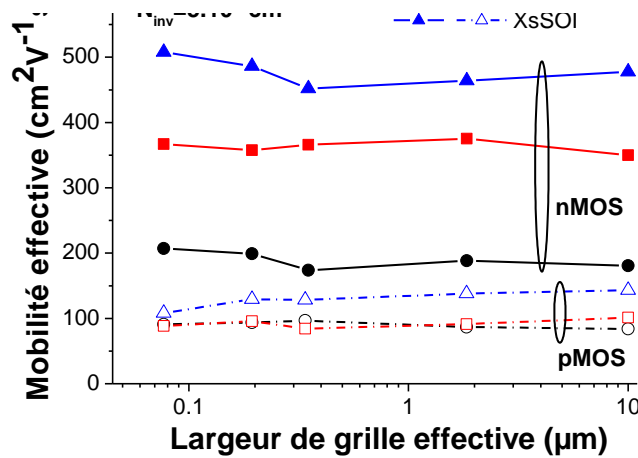
Figure III.58: Mobilité effective en fonction de la largeur de grille effective pour des nMOS et pMOS longs, orientés suivant \langle 110 \rangle , sur SOI, sSOI, XsSOI. La mobilité effective est extraite à densité de charge d'inversion fixée N_{\text{inv}}=5 \times 10^{12} \text{ cm}^{-2} .
