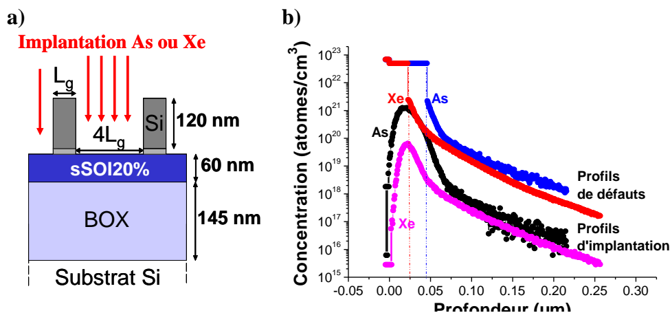
Figure III.31: (a) Schéma des échantillons sSOI obtenus par lithographie e-beam et gravure de l'empilement de grille SiO 2 /Si polycristallin servant de masque pour l'implantation. (b) Simulations C-TRIM des profils d'implantation As et Xe et des profils de défauts.
