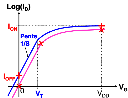
Figure I.2: Caractéristiques I_D(V_G) d'un n-MOSFET.
