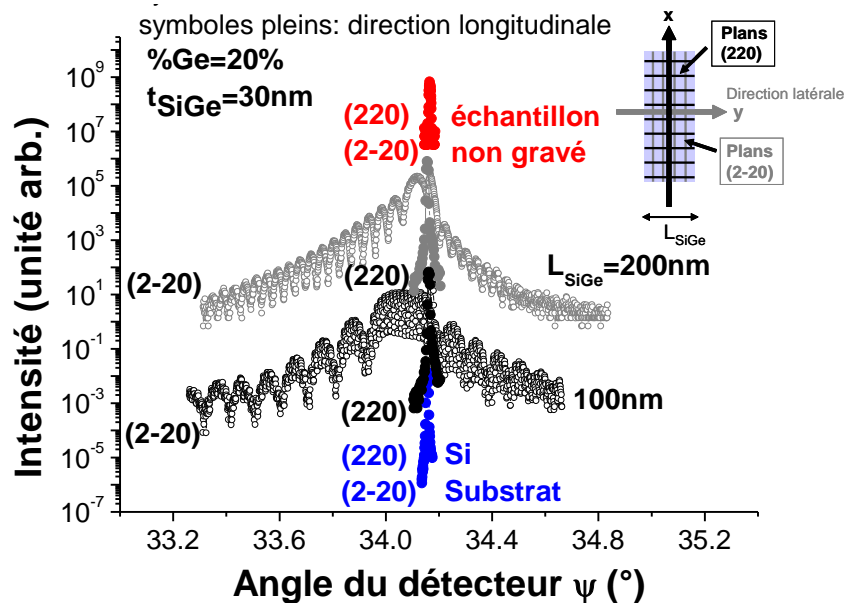
Figure IV.43: Scans radiaux des réflexions (2-20) et (220) d'échantillons d'épaisseur t_{SiGe}=30 nm, de pourcentage en Ge de 20% et de largeurs L_{SiGe}=100 nm et 200 nm. Les pics de Bragg de l'échantillon correspondant non gravé et du substrat de Si sont aussi tracés.
