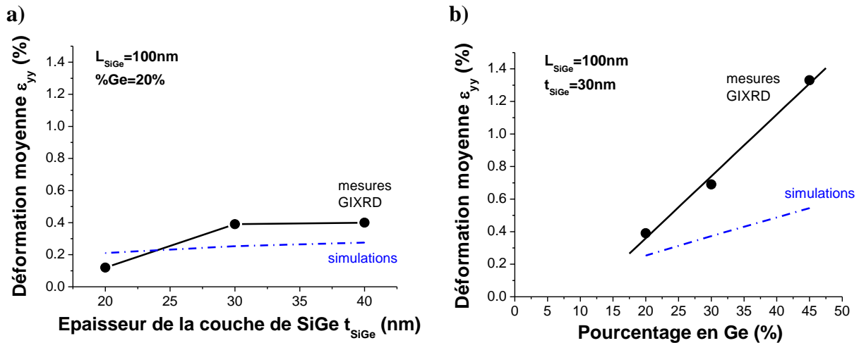
Figure IV.55: Déformation moyenne latérale en fonction a) de l'épaisseur de la couche de SiGe et b) du pourcentage en Ge de la couche de SiGe, d'après les mesures GIXRD et les simulations mécaniques par éléments finis. Pour les simulations, l'épaisseur de surgravure est t_{grav}=0 nm, l'épaisseur de la couche active de Si est t_{Si}=15 nm et l'épaisseur de la couche de SOI est t_{SOI}=15 nm.
