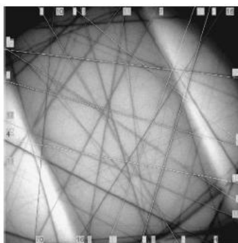
Figure II.4: Figure CBED expérimentale obtenue dans la direction cristallographique <230> de silicium non déformé, avec en superposition les lignes de HOLZ calculées [Armigliato03].
