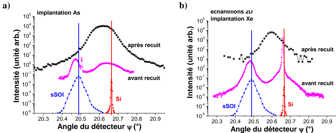
Figure III.37: Scans radiaux dans le plan des réflexions (220) pour les échantillons non gravés implantés a) à l'As avant et après recuit et b) au Xe avant et après recuit. Les pics de Bragg du sSOI et du substrat ont aussi été tracés pour référence. Les conditions expérimentales sont similaires à celles de la figure III.32.
