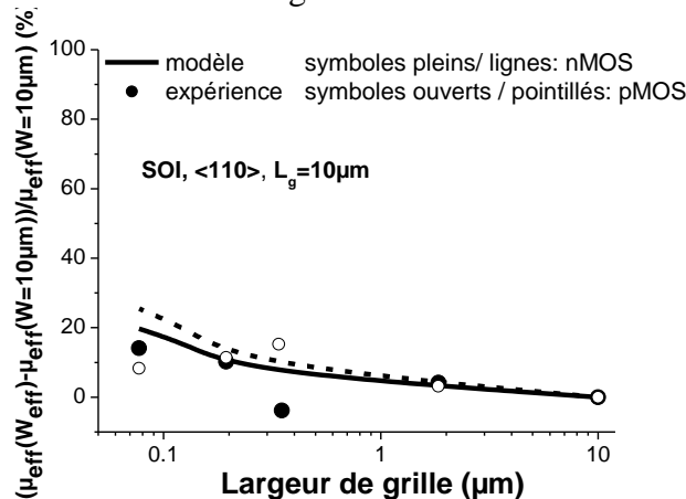
Figure III.59: Mobilité effective normalisée pour des nMOS et pMOS sur SOI orientés \langle 110 \rangle (de longueur de grille L_g=10 \mu\text{m} ) en fonction de la largeur de grille. Les symboles correspondent aux mesures de transport et les lignes au calcul réalisé à partir des mesures de déformation GIXRD et du modèle piézoélectrique.
