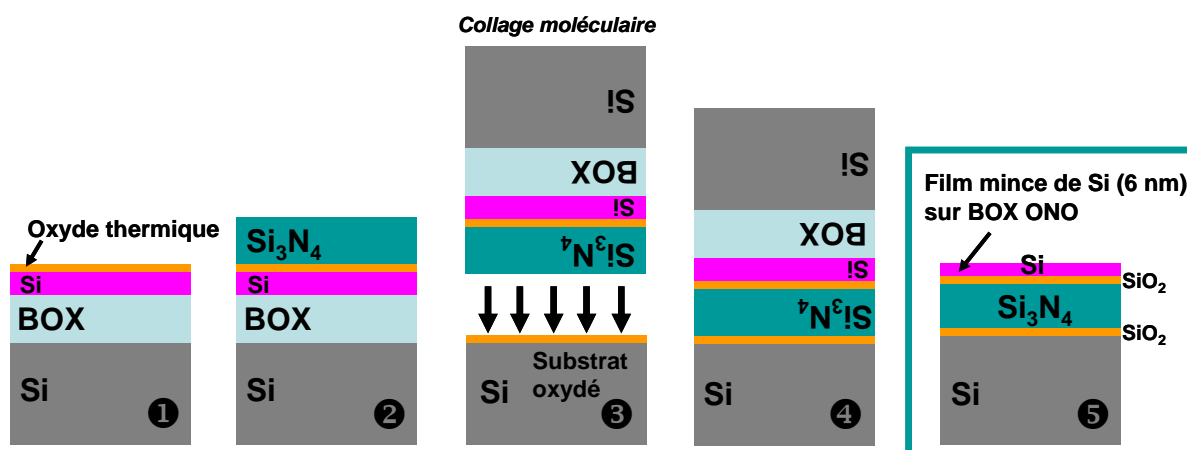
Figure IV.22: Schéma du procédé de fabrication de structures SOI avec un oxyde enterré ONO.
