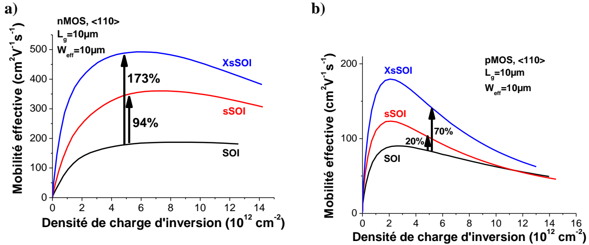
Figure III.53: Mobilité effective en fonction de la densité de charge d'inversion pour des a) nMOS et b) pMOS longs ( L_g=10\ \mu\text{m} ) et larges ( W_{\text{eff}}=10\ \mu\text{m} ), orientés \langle 110 \rangle , sur SOI, sSOI ou XsSOI.
