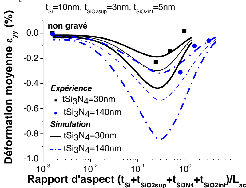
Figure IV.35: Déformation latérale moyenne \varepsilon_{yy} expérimentale et simulée dans la couche active de Si pour des épaisseurs de nitrure de 30 nm et 140 nm en fonction du rapport d'aspect de l'empilement gravé (en considérant une incertitude de \pm 35\% sur la contrainte intrinsèque et de \pm 25\% sur le module d'Young).
