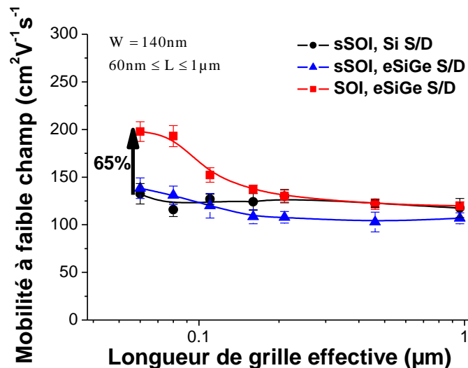
Figure IV.16: Mobilité à faible champ en fonction de la longueur de grille effective pour des pMOS sur sSOI ou sur SOI avec des S/D eSiGe ou en Si, avec une largeur de zone active de 140 nm. Les extractions ont été réalisées à V_D=50 \text{ mV} .
