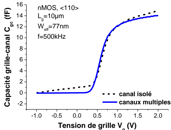
Figure III.48: Capacité grille-canal C_{gc} en fonction de la tension de grille pour des nMOS orientés \langle 110 \rangle , longs et étroits ( L_g=10\ \mu\text{m} , W_{\text{eff}}=77\ \text{nm} ), sur substrats SOI. C_{gc} a été extraite à une fréquence f=500\ \text{kHz} pour un canal isolé et pour des canaux multiples en parallèle (puis divisé par le nombre de canaux) afin de s'affranchir des effets de capacités parasites.
