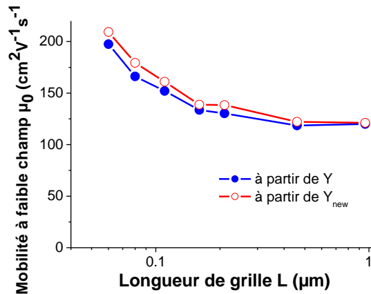
Figure IV.15: Mobilité à faible champ en fonction de la longueur effective, extraite à partir de la fonction Y ou de la fonction Y_{new} , pour des pMOS sur SOI avec des S/D eSiGe.
