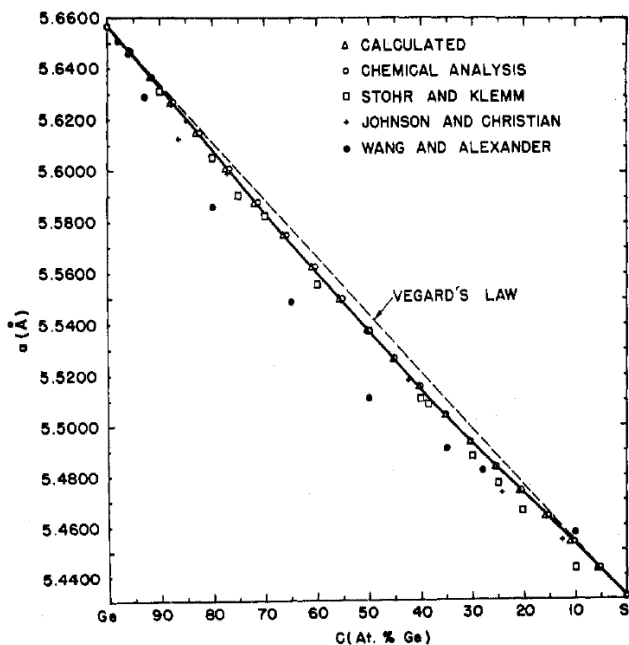
Figure I.13. Variation du paramètre de maille de l'alliage SiGe en fonction de sa composition en Ge [Dismukes64]. La loi de Végard est présentée en pointillés. L'autre droite représente la déviation par rapport à cette loi.
