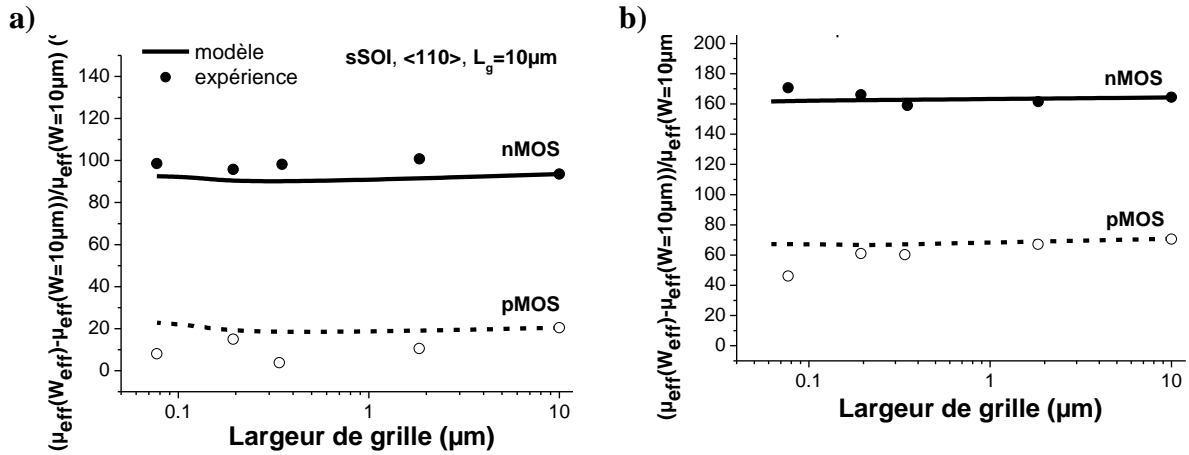
Figure III.60: Mobilité effective normalisée pour des nMOS et pMOS sur a) sSOI et b) XsSOI, orientés <110> (de longueur de grille L g =10 µm) en fonction de la largeur de grille. Les symboles correspondent aux mesures de transport et les lignes au calcul réalisé à partir des mesures de déformation GIXRD et du modèle piézoélectrique.
