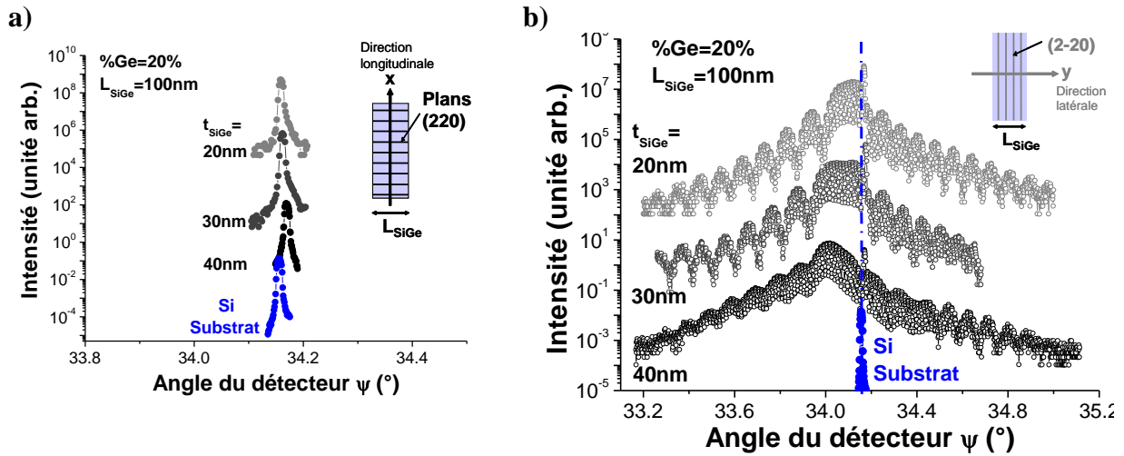
Figure IV.40: Scans radiaux des réflexions (220) (a) et (2-20) (b) d'échantillons d'épaisseur t_{SiGe}=20,30,40 nm, de largeur L_{SiGe}=100 nm et avec un pourcentage en Ge de 20%.
