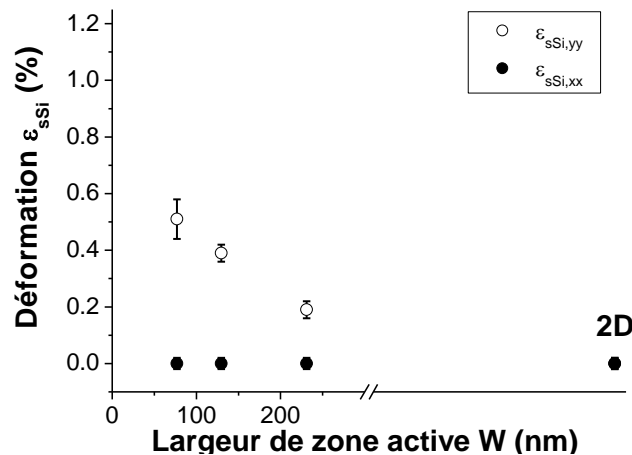
Figure III.28: Déformation dans le plan mesurée en fonction de la largeur W des lignes de SOI, dans les directions longitudinale (symboles pleins) et latérale (symboles ouverts), pour des lignes de SOI non contraintes recouvertes de TiN.
