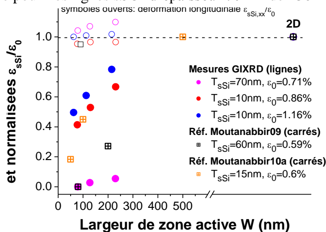
Figure III.18: Déformations longitudinales et latérales moyennes et normalisées par \epsilon_0 (mesurée expérimentalement), dans des lignes et des carrés de sSOI en fonction de la largeur W . Les mesures GIXRD de cette étude sont comparées à celles de [Moutanab09] et [Moutanab10a].
