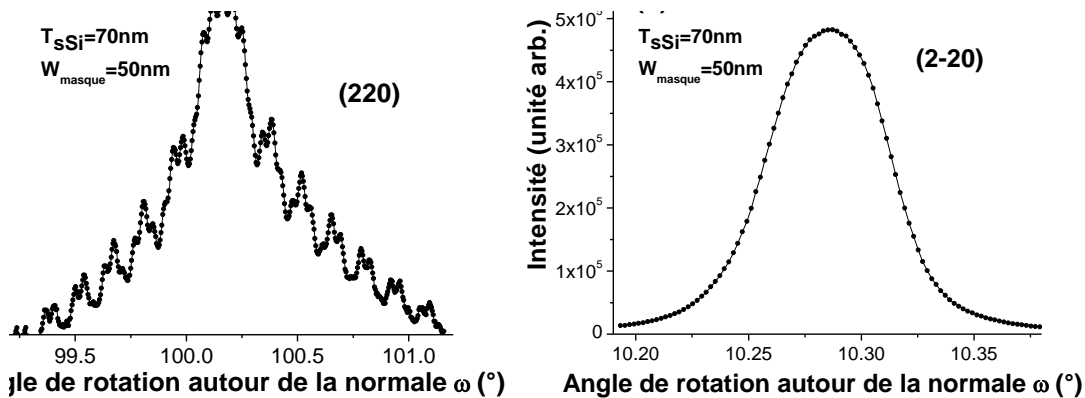
Figure III.6: Scans transverses dans le plan des réflexions (a) (220) et (b) (2-20) pour des lignes de sSOI d'épaisseur 70 nm et de largeur W_{masque}=50 nm.
