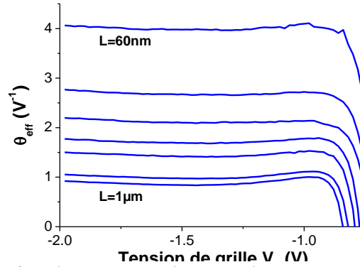
Figure IV.12: Fonction \theta_{\text{eff}} en fonction de la tension de grille pour les différentes longueurs de grille effectives, pour des pMOS sur SOI avec des S/D eSiGe.
