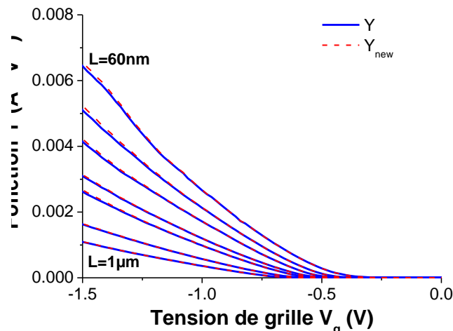
Figure IV.14: Fonction Y et Y_{new} en fonction de la tension de grille pour les différentes longueurs de grille effectives, pour des pMOS sur SOI avec des S/D eSiGe.
