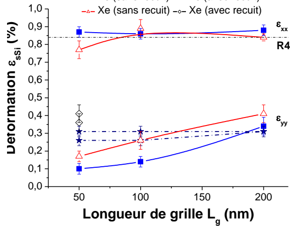
Figure III.41: Déformations dans le plan calculées à partir des données des figures III.38 et III.39 pour les régions sous l'empilement de grille en fonction de la largeur de celui-ci dans les directions longitudinale ( \epsilon_{xx} ) et latérale ( \epsilon_{yy} ) pour des implantations à l'As et au Xe avec et sans recuit.
