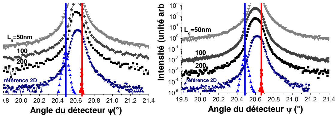
Figure III.38: Scans radiaux dans le plan des réflexions a) (220) le long des lignes et b) (2-20) perpendiculairement aux lignes pour des échantillons implantés à l'As et recuits de différentes largeurs de ligne L_g (50, 100 et 200 nm). Les scans d'échantillons implantés et recuits non gravés, d'échantillons sSOI 2D et du substrat sont tracés comme référence. Les conditions expérimentales sont celles de la figure III.32.
