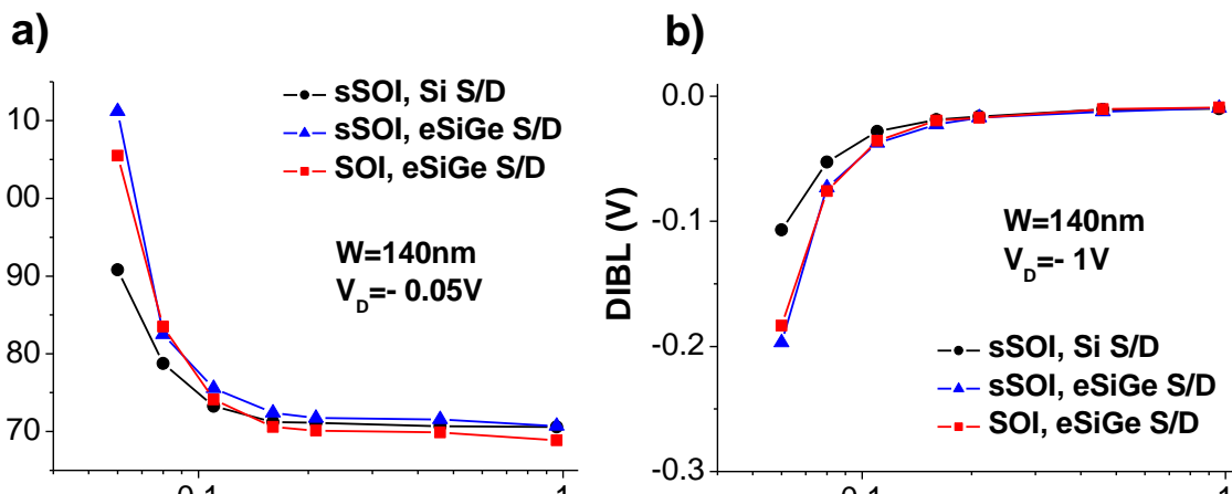
Figure IV.4: a) Pente sous le seuil et b) DIBL en fonction de la longueur de grille effective pour une largeur de zone active de 140 nm.
