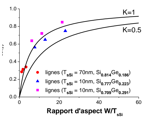
Figure III.26: Ratio \langle \sigma_{sSi,yy} \rangle / \sigma_0 moyen en fonction du rapport d'aspect W / T_{sSi} des lignes contraintes obtenues par gravure à partir des échantillons de référence R1, R2 et R3. Les traits pleins correspondent à une approximation analytique [Loubens03] avec deux rigidités différentes du substrat K=1 et 0.5 (cf. équation III.6).
