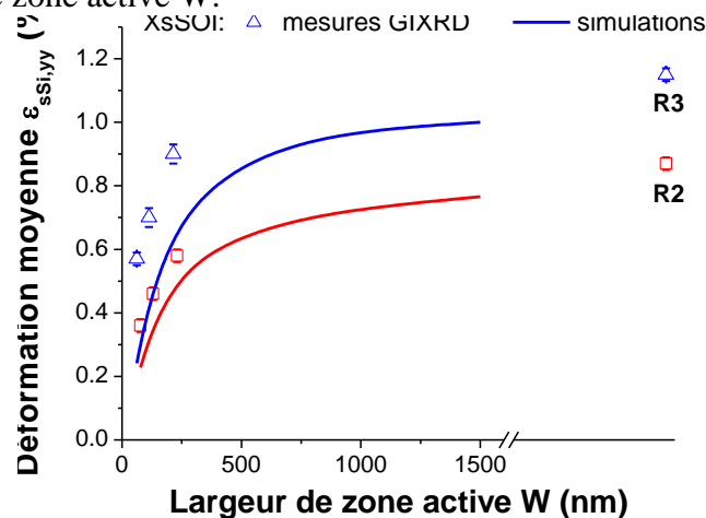
Figure III.25: Comparaison entre les valeurs mesurées et les valeurs obtenues à partir des simulations mécaniques par éléments finis des déformations moyennes dans le plan dans la direction transverse en fonction de la largeur W des lignes de SOI contraint. Les lignes de SOI correspondent aux références R2 (sSOI) et R3 (XsSOI) d'épaisseur de couche active de 10 nm.
