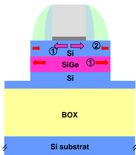
Figure IV.42: Mécanismes de transfert de contrainte dans une structure STS à base de SiGe enterré. Le mécanisme 1 est la relaxation par les bords de la contrainte intrinsèque en compression du SiGe, qui induit une contrainte en tension dans la couche active de Si. Le mécanisme 2 est la relaxation de la contrainte en tension de la couche active de Si par les bords.
