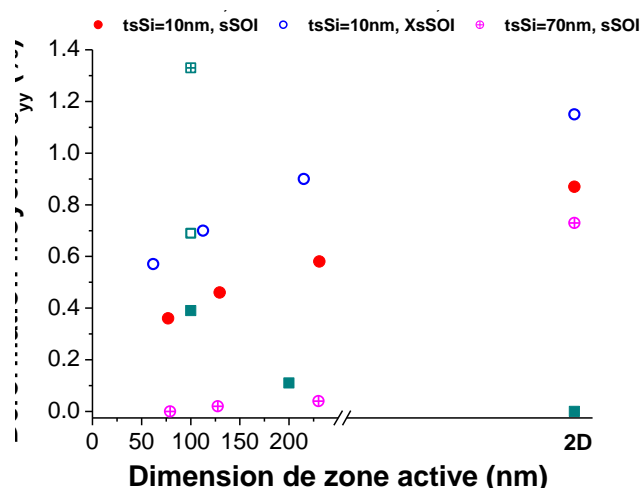
Figure IV.59: Comparaison des structures sSOI et STS à base de SiGe. Pour les structures STS, la déformation moyenne est la déformation moyenne dans l'empilement Si/SiGe/Si. Pour les structures sSOI, la déformation moyenne est la déformation moyenne dans la couche active de Si. L'épaisseur de la couche active de Si dans le cas des structures STS est 15 nm et celle de la couche de SOI 15 nm.
