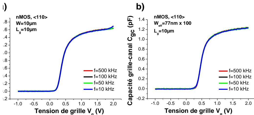
Figure III.49: Influence de la fréquence de mesure sur la capacité grille-canal de nMOS longs ( L_g=10\ \mu\text{m} ), a) larges ( W=10\ \mu\text{m} ) ou b) étroits ( W_{\text{eff}}=77\ \text{nm} ).
