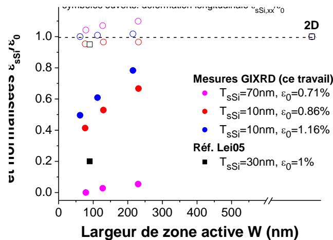
Figure III.17: Déformations longitudinales et latérales moyennes dans des lignes sSOI en fonction de la largeur W . Les valeurs ont été normalisées par la moyenne \epsilon_0 sur l'épaisseur du film de la déformation dans le plan \epsilon_{xx}=\epsilon_{yy} des échantillons 2D, mesurée expérimentalement. Les mesures GIXRD de cette étude sont comparées à celles de [Lei05].
