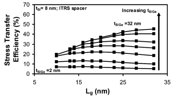
Figure IV.48: Efficacité du transfert de contrainte STE pour une épaisseur de Si fixée et une épaisseur de SiGe variable. La largeur de l'espaceur est fixée à 1.1 \times L_g , comme spécifié par l'ITRS. D'après [Fiorenza08].
