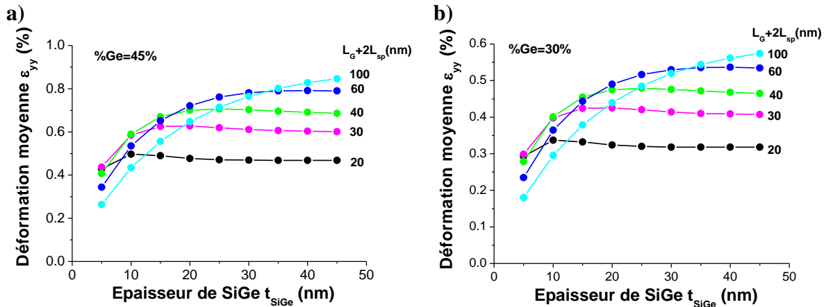
Figure IV.54: Déformation moyenne latérale dans la couche active de Si en fonction de l'épaisseur de la couche de SiGe, pour différents longueurs de grille et pour un pourcentage en Ge de la couche de SiGe de a) 45% et b) 30%. L'épaisseur de surgravure est t_{grav}=5 nm, l'épaisseur de la couche active de Si est t_{Si}=5 nm et l'épaisseur de la couche de SOI est t_{SOI}=15 nm.
