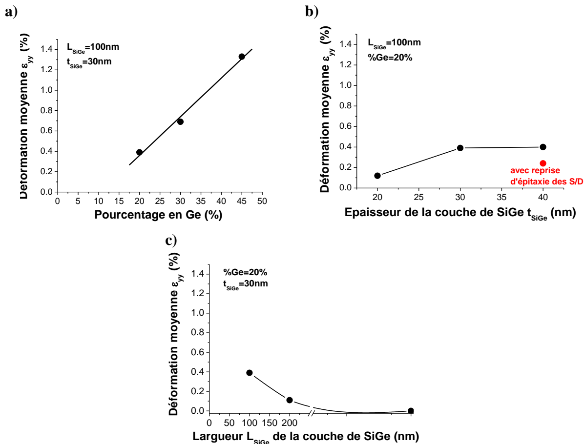
Figure IV.46: Déformation latérale moyenne \varepsilon_{yy} dans l'empilement Si/SiGe/Si en fonction a) du pourcentage en Ge de la couche de SiGe, b) de l'épaisseur de la couche de SiGe, c) de la largeur de la couche de SiGe.
