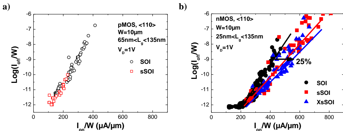
Figure III.54: Compromis I_{\text{on}}/I_{\text{off}} (à V_D=1\text{V} ) pour des a) pMOS et b) nMOS larges et courts, orientés \langle 110 \rangle , sur substrats SOI, sSOI et XsSOI.
