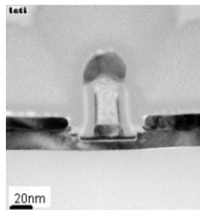
Figure III.44: Image TEM d'un n-MOSFET FDSOI de longueur de grille 25 nm sur un substrat SOI non contraint, avec un canal orienté dans la direction \langle 110 \rangle . L'empilement de grille est HfO 2 /TiN. Les épaisseurs de la couche de Si active et de l'oxyde enterré sont respectivement T_{\text{Si}}=9 \text{ nm} et T_{\text{BOX}}=145 \text{ nm} .
