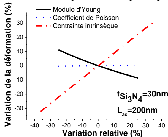
Figure IV.33: Impact des constantes élastiques du nitrure sur la déformation latérale ( \varepsilon_{yy} ) moyenne dans la couche active de Si.
