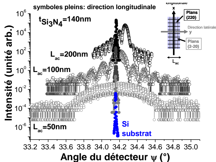
Figure IV.28: Scans radiaux des pics de Bragg correspondant aux réflexions (220) et (2-20) des couches supérieures de Si active de différentes largeurs L_{\text{ac}}=50, 100, 200 nm et du substrat de silicium pour des structures avec un nitrure enterré de 140 nm d'épaisseur. Seulement un pic de substrat a été représenté, car il est toujours mesuré à la même position pour chaque échantillon. Insert : Plans cristallographiques mesurés en GIXRD et directions correspondantes pour la mesure des déformations.
