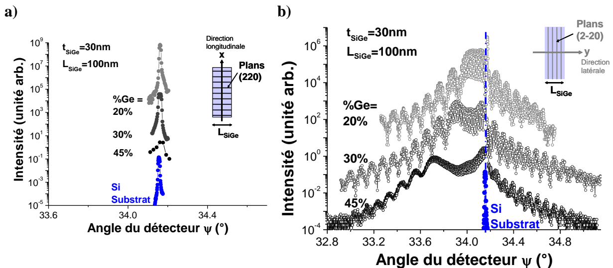
Figure IV.41: Scans radiaux des réflexions (220) (a) et (2-20) (b) d'échantillons d'épaisseur t_{SiGe}=30 nm, de largeur L_{SiGe}=100 nm et avec des pourcentages en Ge de 20%, 30% et 45%.
