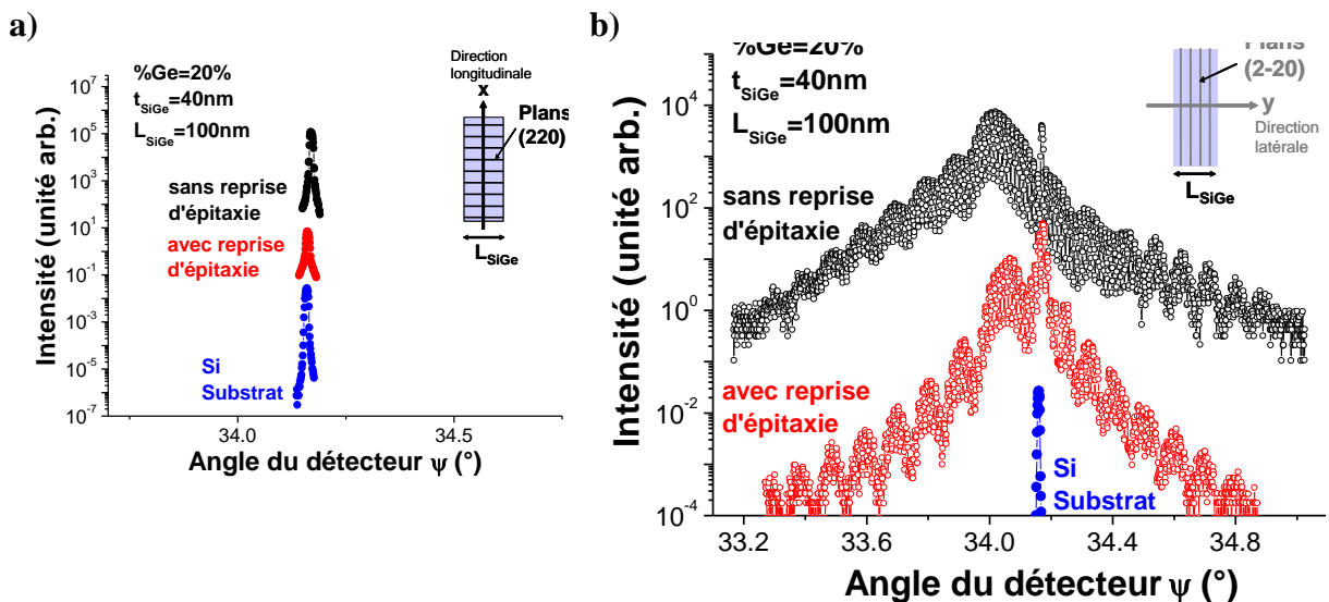
Figure IV.45: Scans radiaux des réflexions (220) (a) et (2-20) (b) d'échantillons d'épaisseur t_{SiGe}=40 nm, de largeur L_{SiGe}=100 nm et avec des pourcentages en Ge de 20%. La figure compare les pics de Bragg de deux échantillons avec et sans reprise d'épitaxie.
