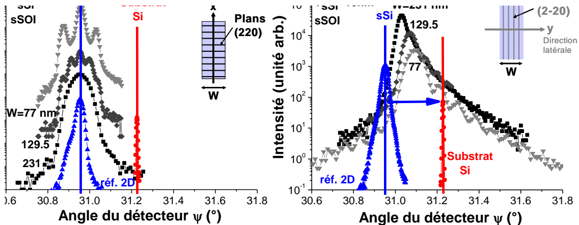
Figure III.12: Scans radiaux dans le plan des réflexions (220) et (2-20) le long (a) et perpendiculairement à la direction des lignes (b) pour des lignes de sSOI d'épaisseur 10 nm et de différentes largeurs W. Les conditions expérimentales sont les mêmes que celles de la figure III.11.
