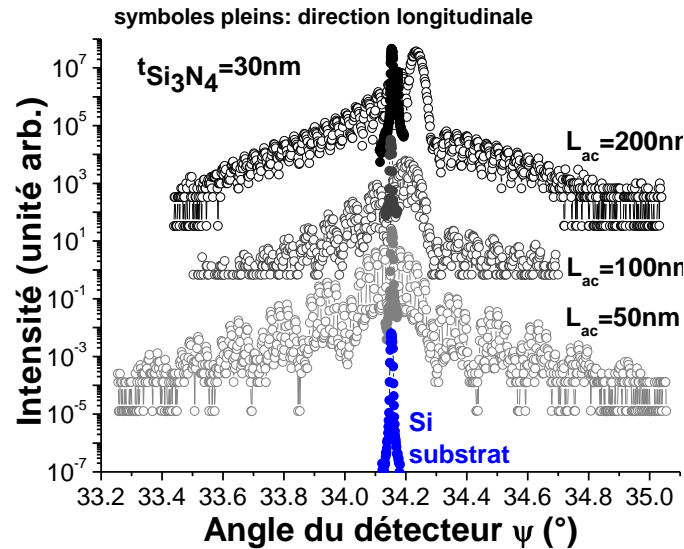
Figure IV.29: Scans radiaux des pics de Bragg correspondant aux réflexions (220) et (2-20) des couches supérieures de Si active de différentes largeurs L_{ac}=50,100,200 nm et du substrat de silicium pour des structures avec un nitrure enterré de 30 nm d'épaisseur. Seulement un pic de substrat a été représenté, car il est toujours mesuré à la même position pour chaque échantillon.
