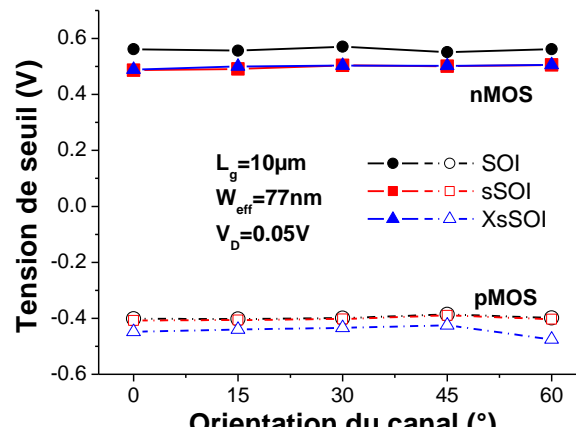
Figure III.61: Tension de seuil en fonction de l'orientation du canal pour des n- et p-MOS longs et étroits sur substrats SOI, sSOI et XsSOI. La tension de seuil est extraite à faible courant de drain (V D =50 mV).
