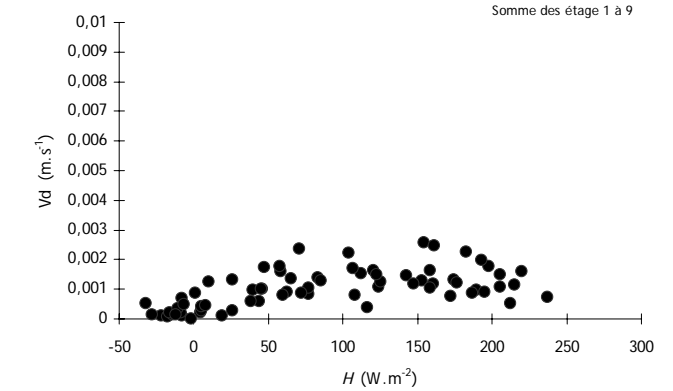
Figure annexe.19: Vd en fonction de H , Landes 2, étages 5 à 9 et somme des étages 1 à 9
