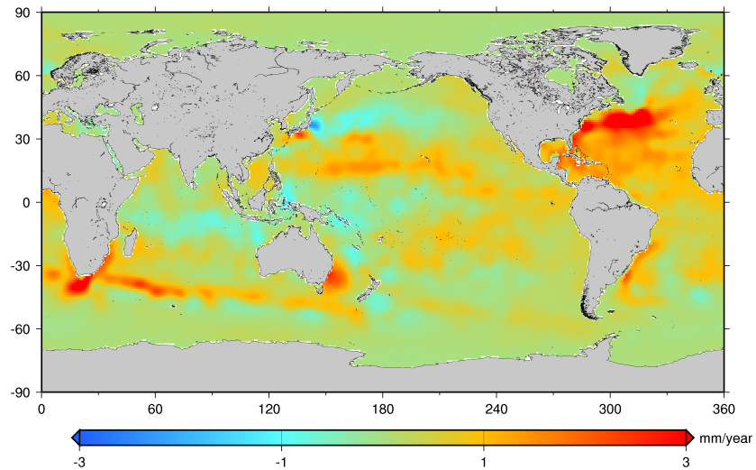
FIG. 5.12 – Cartographie des taux de variation du niveau de la mer thermostérique entre 1955 et 2008 d’après les données de Levitus et al. [2009]
