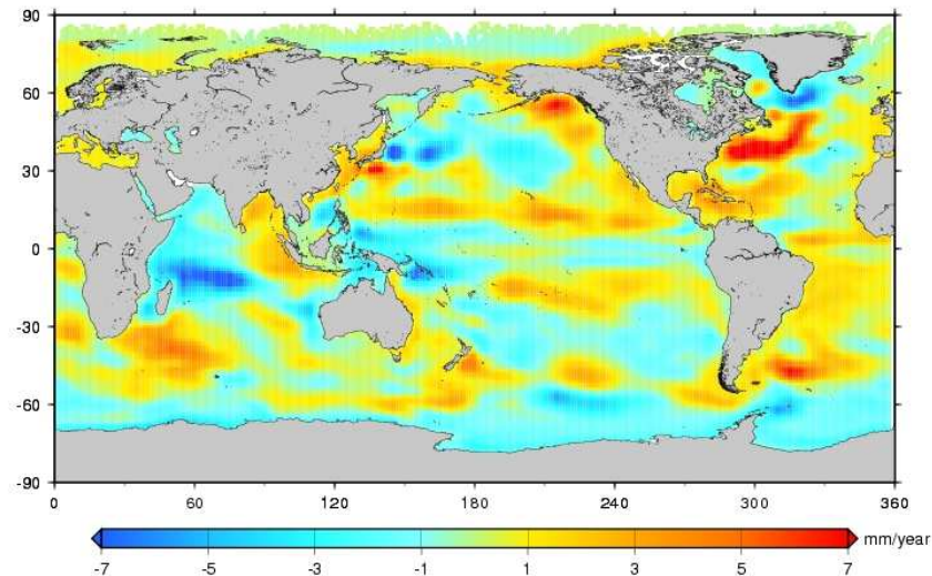
FIG. 5.8 – Cartographie des taux de variation du niveau de la mer reconstruit entre 1950 et 2003 (d'après Llovel et al. [2009] ).
