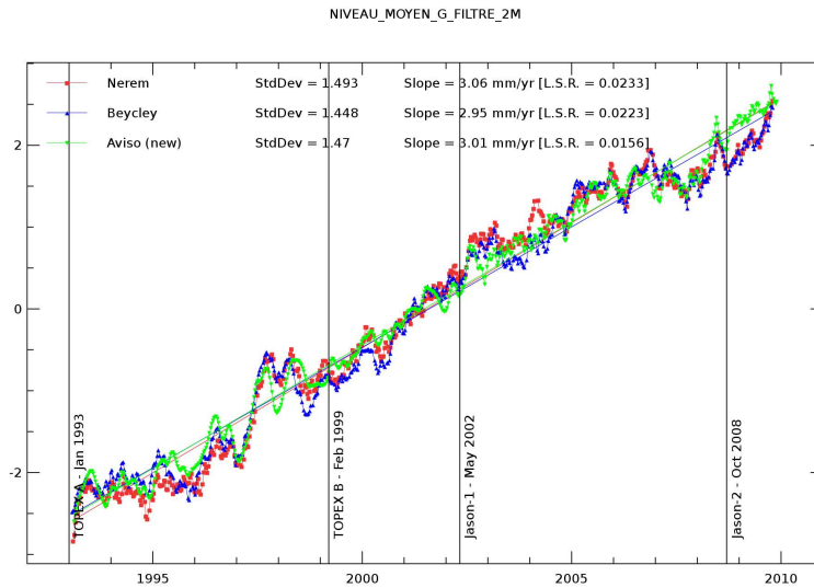
FIG. 2.7 – Variations du niveau moyen global de la mer sur la période 1993-2009 pour différents produits fournis par les groupes de recherche de l'Université du Colorado (courbe rouge, Nerem et al. [2006]), GSFC/NASA (courbe bleue, Beckley et al. [2010]) et CLS (courbe verte, Ablain et al. [2009]).
