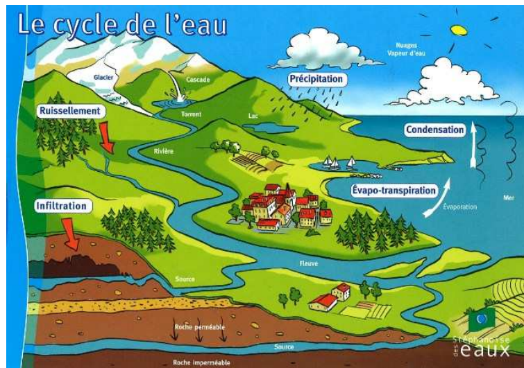
FIG. 4.8 – Cycle global de l'eau
