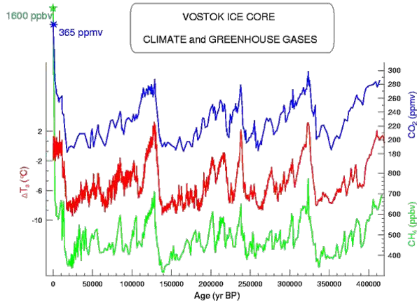
FIG. 2.2 – Evolutions au cours des derniers 450 000 ans de la teneur en CO_2 (courbe bleue), en CH_4 (courbe verte) et de la température (par rapport à la moyenne, courbe rouge) en Antarctique déduites de l'analyse des carottes glaciaires de Vostok ( Petit et al. [1999]; Raynaud et al. [2005]) et EPICA ( community members [2004])
