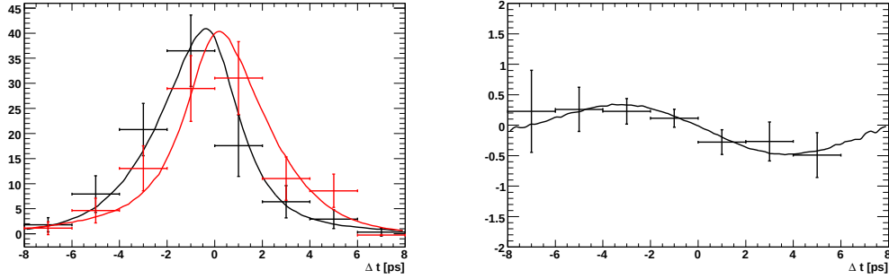
Figure 0.1: sPlots pour \Delta t côté signal. A gauche sont montrées les distributions du temps propre \Delta t pour des mésons B côté signal (étiquetés comme B^0 en noir et des mésons B étiqueté comme \bar{B}^0 en rouge). La figure de droite montre l'asymétrie dépendant du temps.
