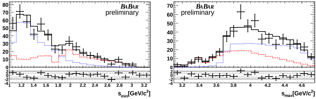
Figure 0.3: Projections du résultat de l'ajustement sur les axes du plan de Dalitz( s_{\min} à gauche et s_{\max} à droite). Les données sont indiquées avec leurs barres d'erreur. La ligne rouge tireté (pointillée bleue) correspond au signal (bruit de fond) et la ligne noire correspond au modèle total.
