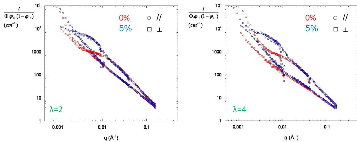
Figure 5.30 – Comparaison des signaux DNPA d’une matrice de 430 \text{ kg.mol}^{-1} non chargée avec un nanocomposite chargé à 5\% \text{ v/v} . Aux q intermédiaires, les signaux se superposent : les chaînes se déforment de la même manière.
