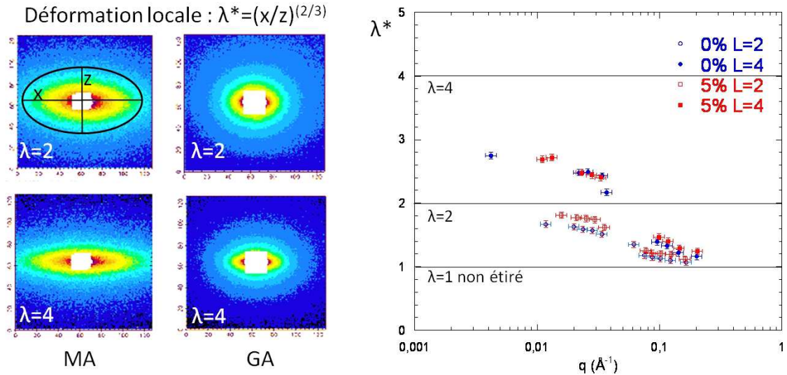
Figure 5.28 – Mesure de la déformation locale \lambda^* à partir des axes de l'ellipse (à gauche). A droite, \lambda^* = f(q) pour les nanocomposites de masse 315 \text{ kg.mol}^{-1} à 0% et 5%v/v en silice.
