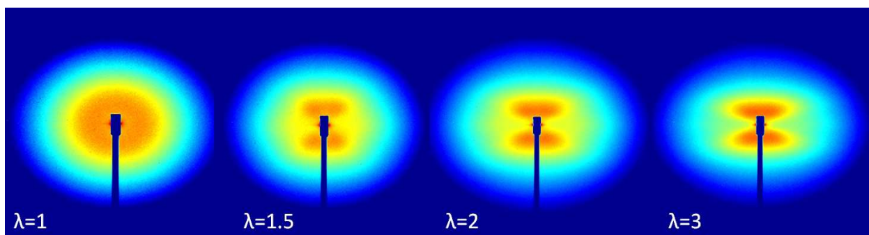
Figure 5.16 – Figures 2D obtenues par DXPA pour un nanocomposite Nissan/PMMA 15%v/v à différents taux d'élongation. De gauche à droite, \lambda = 1 , \lambda = 1.5 , \lambda = 2 , \lambda = 3 . La gamme de vecteur de diffusion q est 0.0021\text{\AA}^{-1} < q < 0.034\text{\AA}^{-1} dans la direction parallèle et 0.0008\text{\AA}^{-1} < q < 0.03\text{\AA}^{-1} dans la direction perpendiculaire ( ID02-ESRF ).
