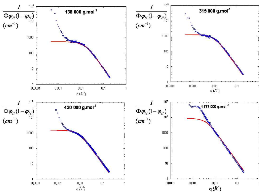
Figure 4.5 – Spectres DNPA (en bleu) des matrices non chargées en fonction de la masse molaire (de 138 à 1777 \text{kg.mol}^{-1} ). Le trait plein rouge correspond à la modélisation par la fonction de Debye.
