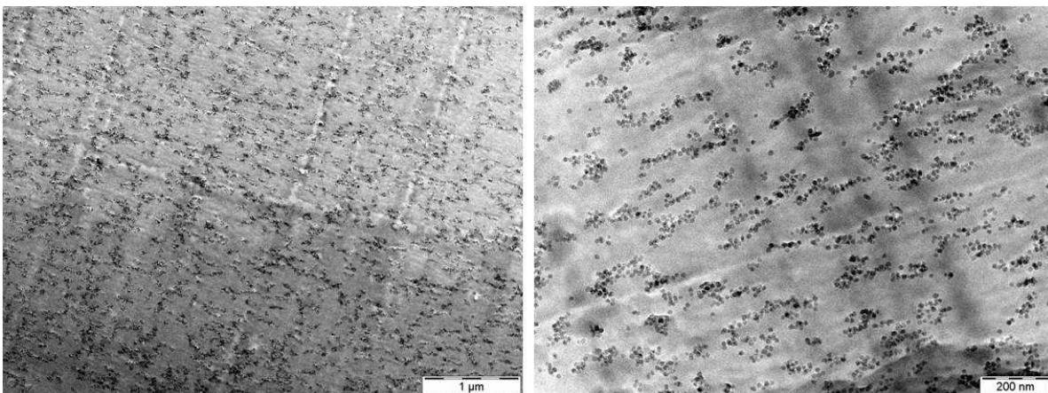
Figure 2.20 – Clichés MET du systèmes Ludox LS/PS 5%v/v : à gauche faible grossissement, à droite fort grossissement.
