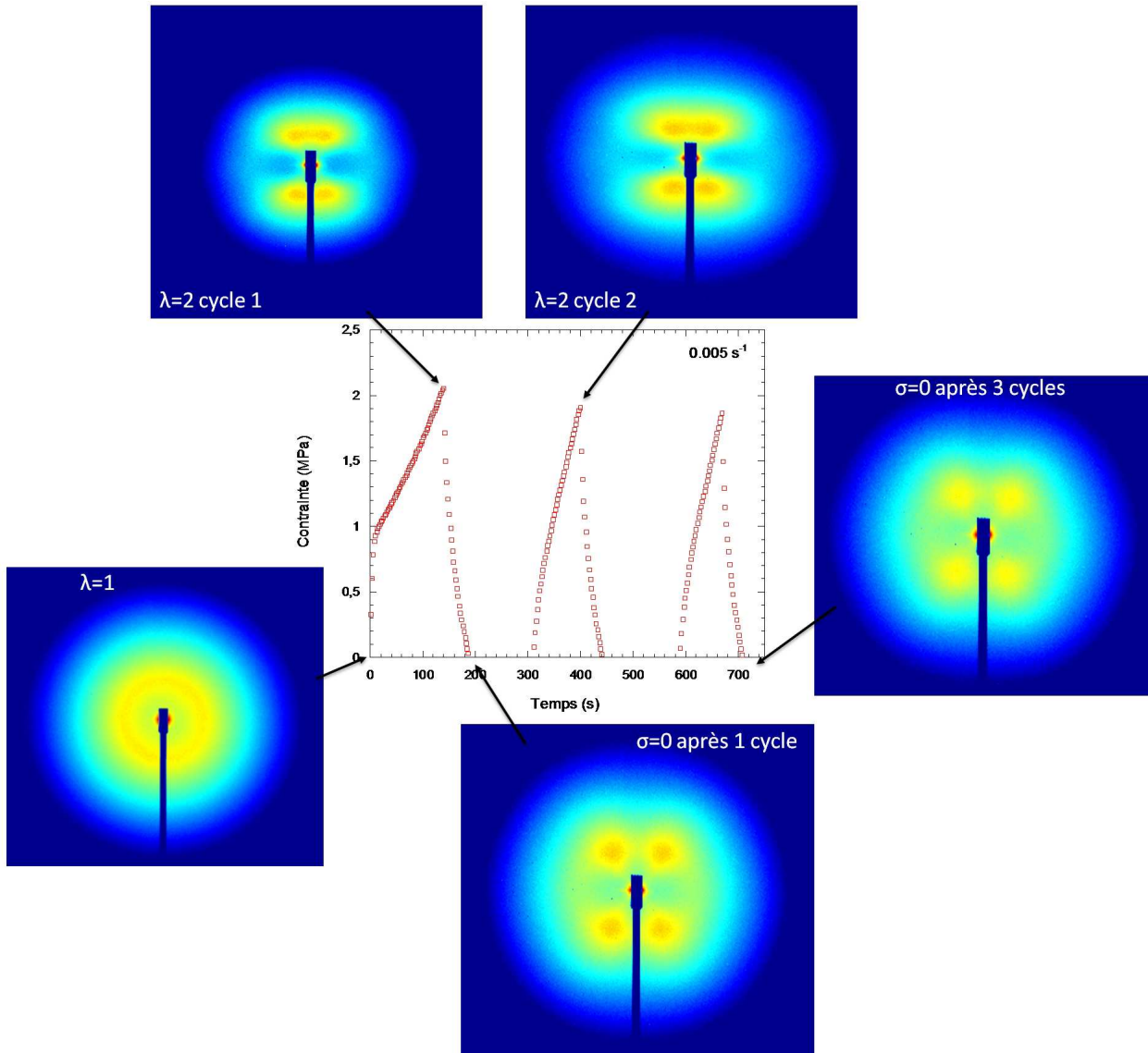
Figure 5.23 – Figures de diffraction 2D au cours de cycles de déformation du nanocomposite Nissan/PMMA 20%. Les mesures DXPA ont été effectuées à cinq instants : \lambda = 1 (état non étiré), \lambda = 2 , retour à contrainte nulle, \lambda = 2 du deuxième cycle et retour à contrainte nulle à la fin du troisième cycle. La déformation est appliquée verticalement avec un gradient de vitesse de 0.005 \text{ s}^{-1} à T_g + 20^\circ\text{C} ( ID02-ESRF ).
