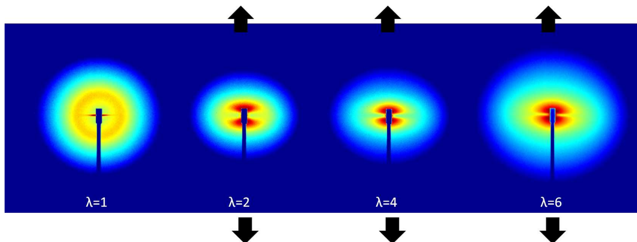
Figure 5.14 – Figures de diffusion 2D obtenues en DXPA pour des nanocomposites Nissan/PS 15%v/v. De gauche à droite le taux d'élongation augmente : \lambda = 1, \lambda = 2, \lambda = 4, \lambda = 6 . Les flèches noires représentent le sens de l'étirement. Ces figures correspondent à une configuration donnée (10m et 10keV). La gamme de vecteur de diffusion q est 0.0021\text{Å}^{-1} < q < 0.034\text{Å}^{-1} dans la direction parallèle et 0.0008\text{Å}^{-1} < q < 0.03\text{Å}^{-1} dans la direction perpendiculaire ( ID02-ESRF ).
