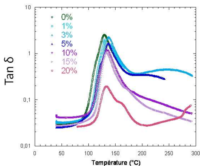
Figure 3.6 – Facteur de perte \tan \delta pour les nanocomposites Nissan/PS pour différentes fractions volumiques (de 0% à 20%v/v).
