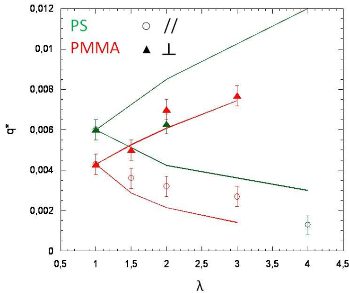
Figure 5.18 – Evolution de la position du pic en fonction du taux d'élongation dans les deux directions de l'étirement pour les nanocomposites Nissan/PS 15% et Nissan/PMMA 15%v/v . Les traits pleins correspondent à l'évolution si la déformation est affine.
