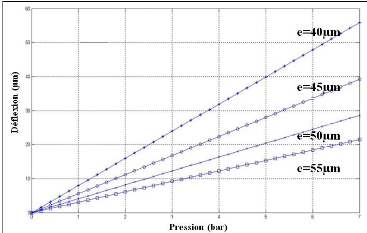
Fig II. 17. Variation de la déflexion maximale du centre d'une membrane (circulaire de diamètre d=2800\mu\text{m} ) en fonction de la pression pour différentes épaisseurs
