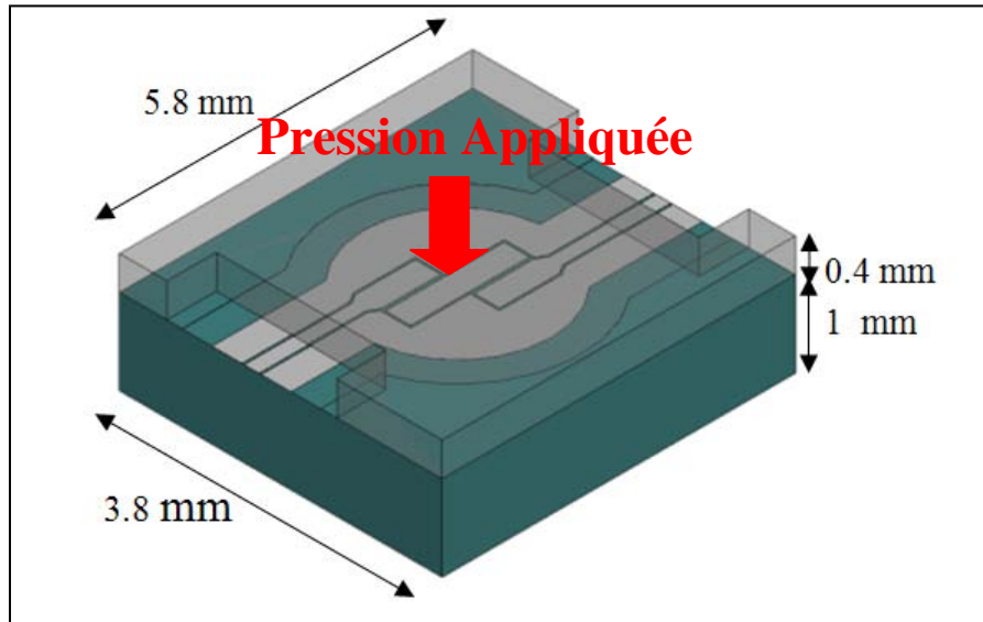
Fig II. 14. Premier prototype du capteur à transduction EM
