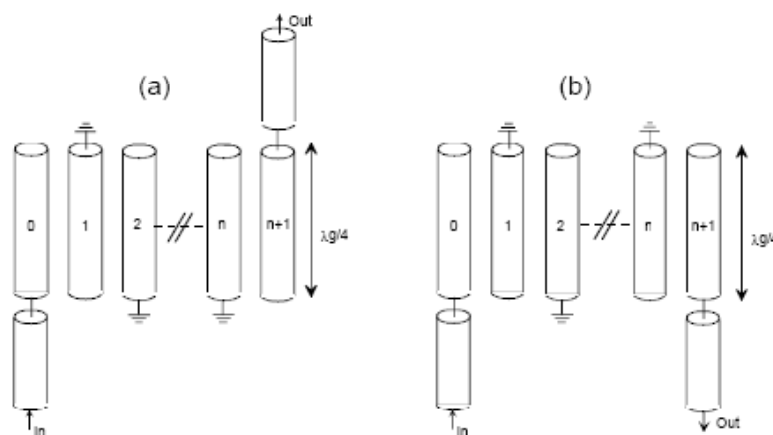
Fig E. 7. Filtres interdigités en lignes de transmissions idéales
