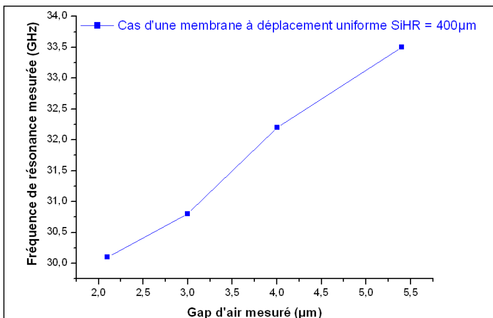
Fig III. 33. Résultats de mesure pour une membrane à déplacement uniforme (SiHR=400 \mu\text{m} )
