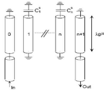
Fig E. 6. Filtre combine en ligne de transmission idéale
