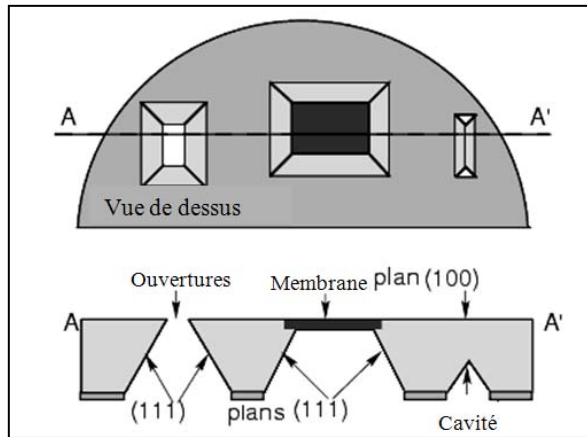
Fig III. 20. Profil de gravure humide KOH du silicium
