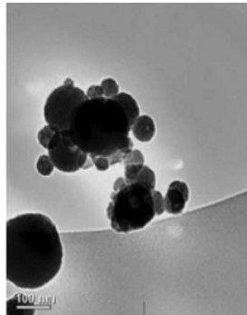
Figure 22. Image TEM de nanoparticules d'Al/Fe 2 O 3 auto-assemblées par force électrostatique
