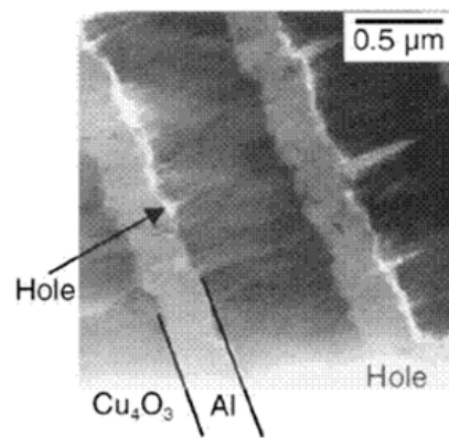
Figure 15. Multicouches Cu_4O_3/Al réalisées par PVD - observation au TEM [92]
