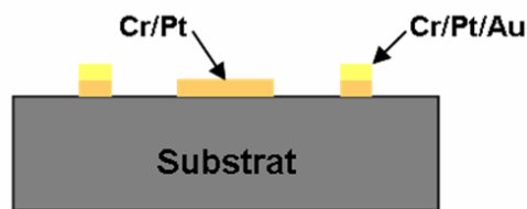
Figure 63. Gravure de l'or - Résistances en serpentins constituées de Cr/Pt/Au
