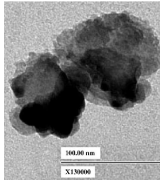
Figure 13. Nanoparticules d'aluminium recouvertes d'une couche mince de SnO 2 déposée par ALD
