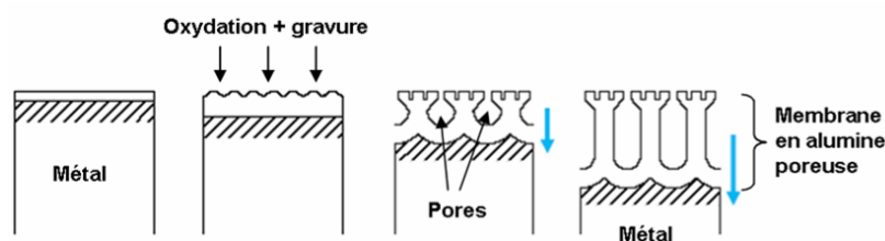
Figure 16. Principe du procédé d'anodisation [114]
