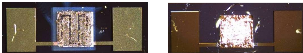
Figure 70. Micro initiateur après initiation de la nanothermite sous forme de (a) : nanofils. (b) : multicouches
