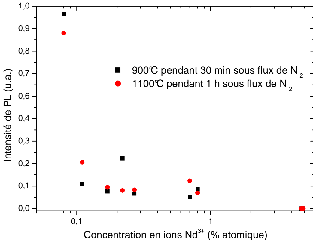
Figure III.25 : Evolution de l'intégrale du pic à 0,92 \mu\text{m} de la PL des échantillons contenant un excès de Si de 7,5% atomique en fonction de la concentration en Nd 3+ .
