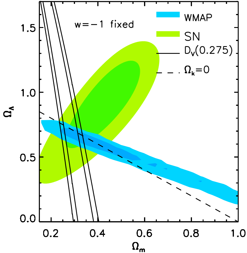
FIG. 1.4 – Combinaison des contraintes sur les paramètres (\Omega_m, \Omega_\Lambda) du modèle \Lambda CDM issues de la mesure de la distance luminosité des SN Ia (Union supernovae [195]), du CMB (WMAP5) et des BAO (SDSS - release 7). Les ellipses des contraintes associées des trois types de mesures sont orientées d'une façon très différente : l'association des trois observations permet donc de mesurer les paramètres (\Omega_m, \Omega_\Lambda) beaucoup plus précisément qu'avec chacune des méthodes séparément. La figure provient de [212].
