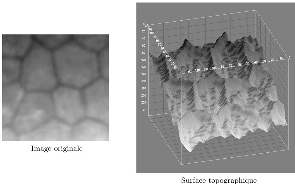
FIG. 5.1 – Image de taille 128 \times 128 de cellules d’endothélium cornéen humain représentée en 256 niveaux de gris et sa surface topographique.
