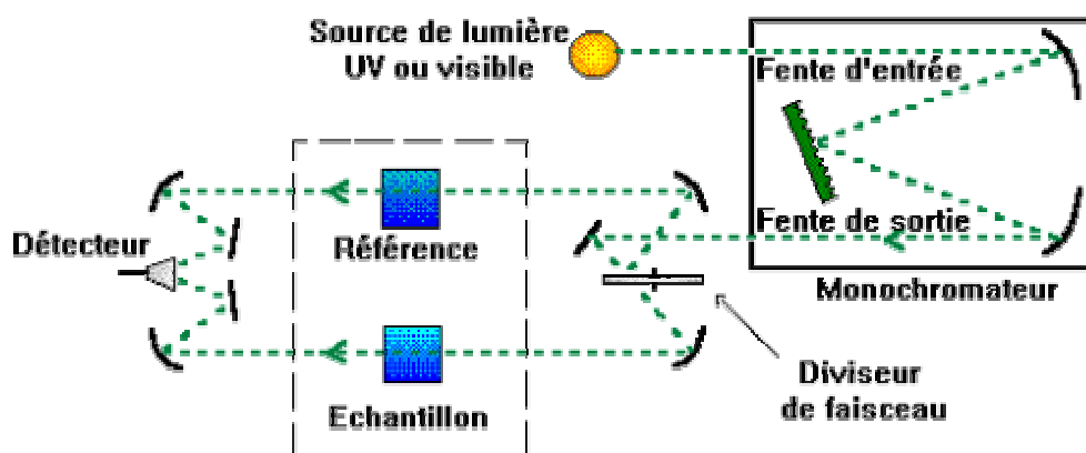
Figure 9 : Principe de fonctionnement d'un spectromètre UV-visible
