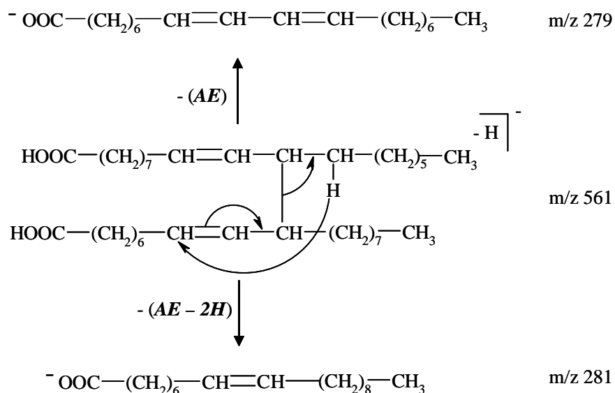
Figure 30 : Mécanisme de réarrangement à six centres permettant l'obtention des ions à m/z 279 et m/z 281 à partir d'une molécule issue d'une addition radicalaire suivie d'une élimination (RAE)
