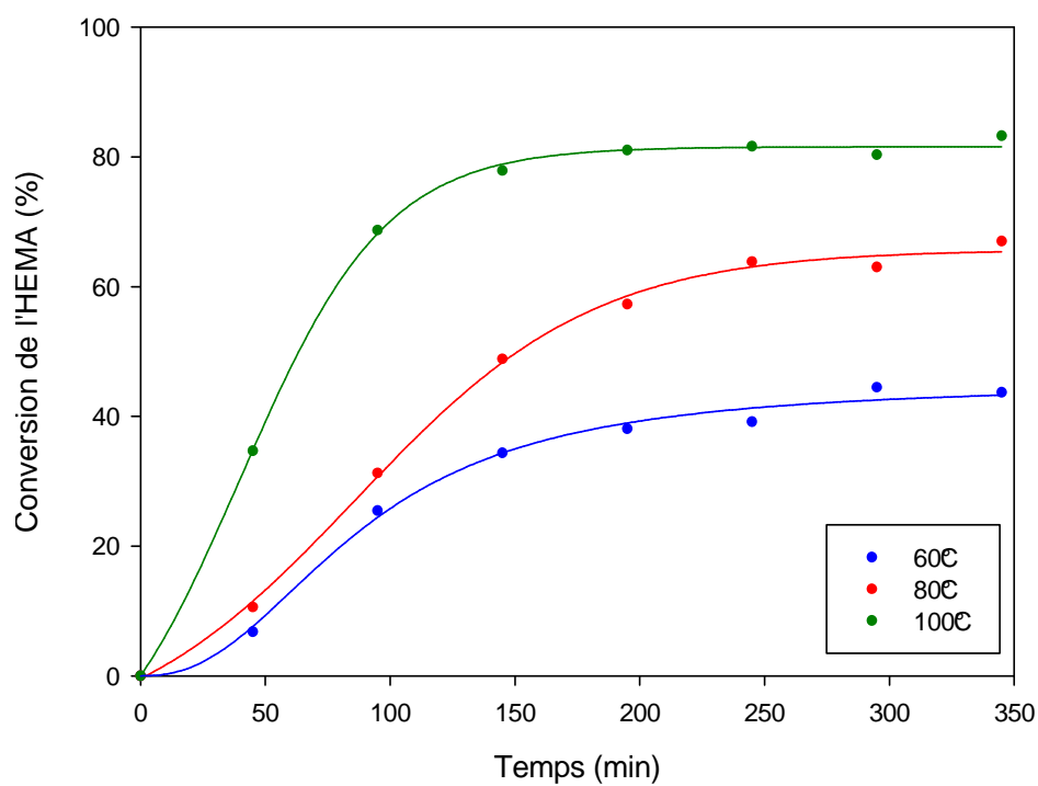
Figure 24 : Influence de la température sur la polymérisation de l'HEMA
