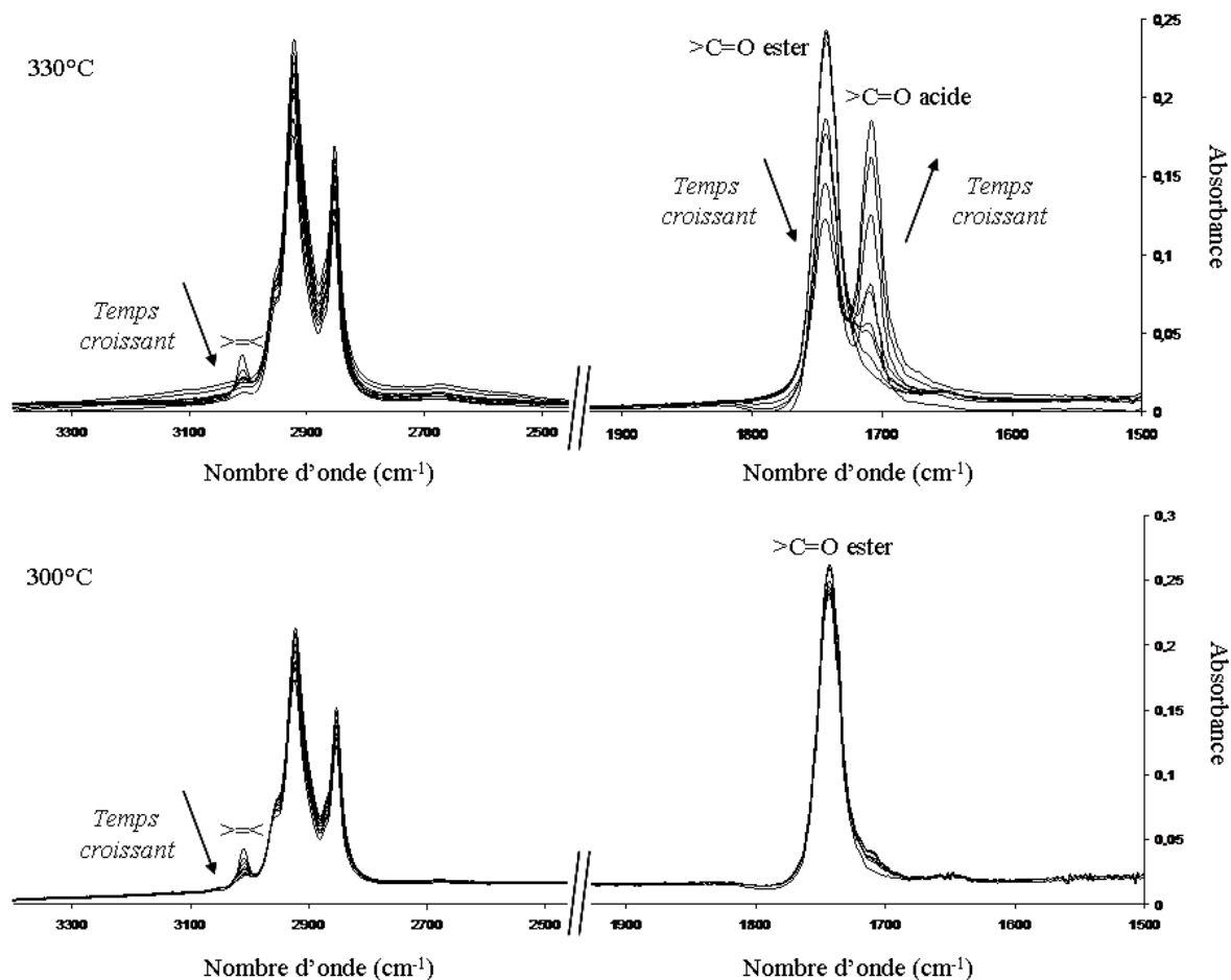
Figure 9 : Evolution des spectres infra-rouge d'huiles de lin standolisées à 300°C et 330°C
