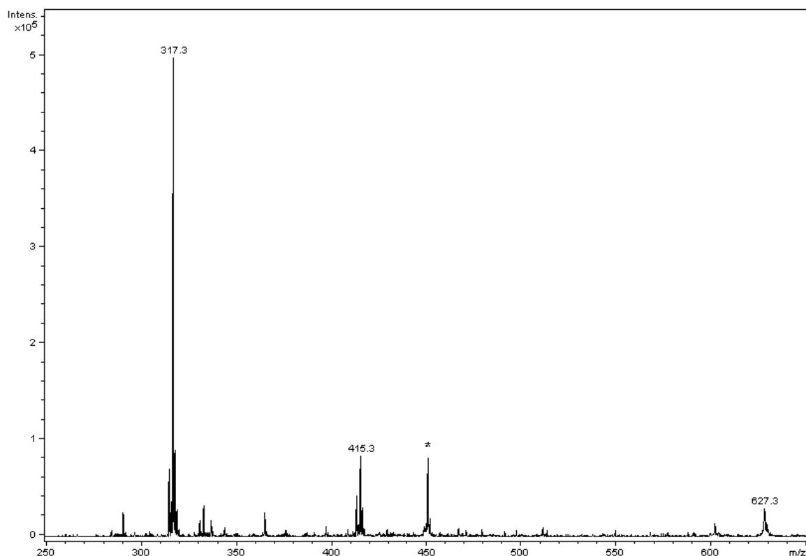
Figure 3 : Spectre MS du mélange réactionnel (OE + AM) (* : contaminant)
