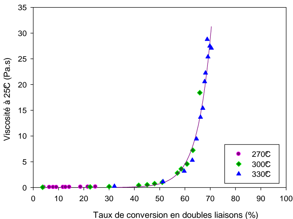
Figure 10 : Evolution de la viscosité des huiles standolisées à différentes températures en fonction de la conversion en doubles liaisons
