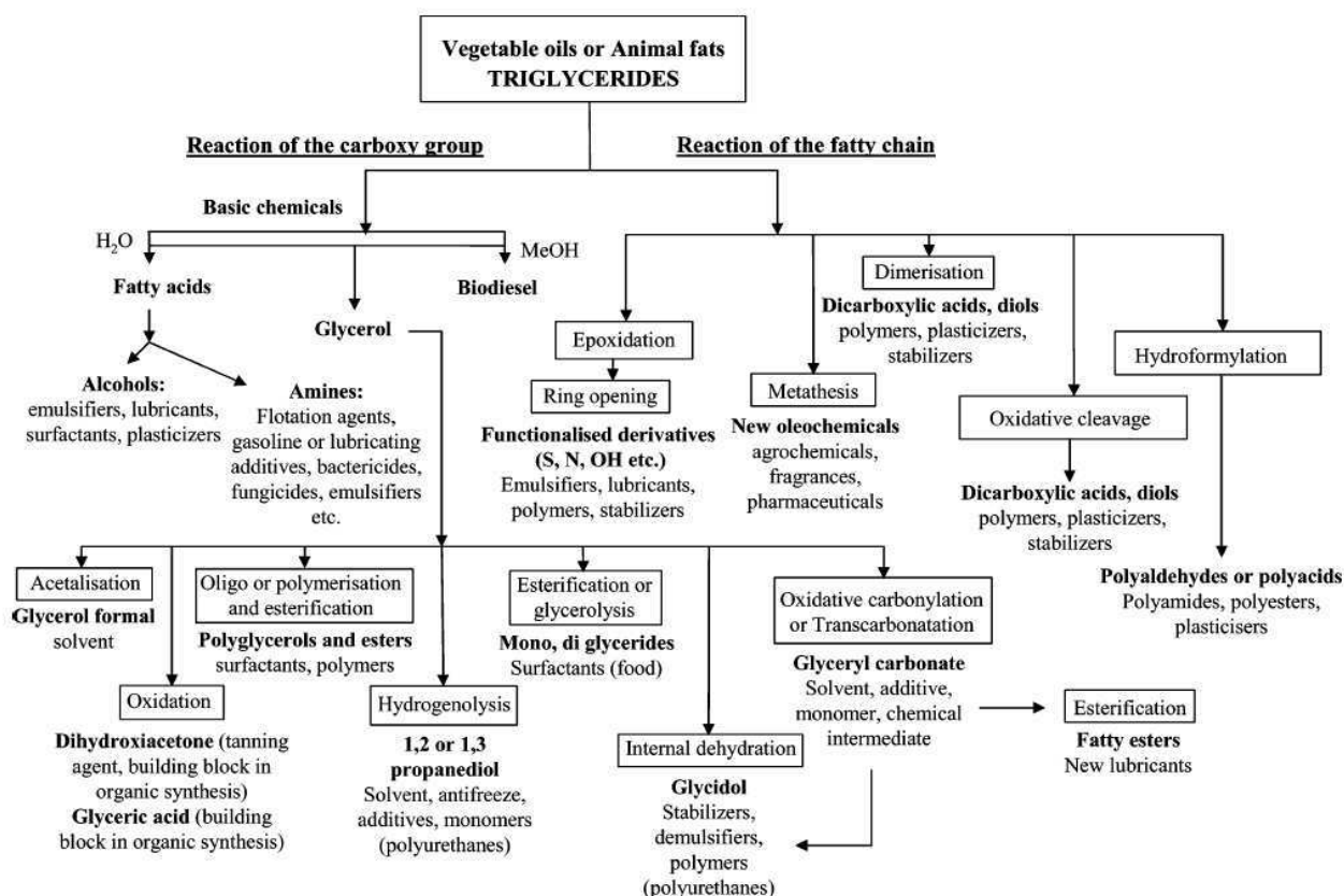
Figure 40 : Récapitulatif des différentes modifications chimiques pouvant être réalisées sur les huiles végétales 70
