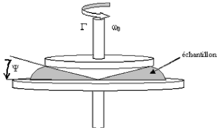
Figure 8 : Géométrie plan-cône
