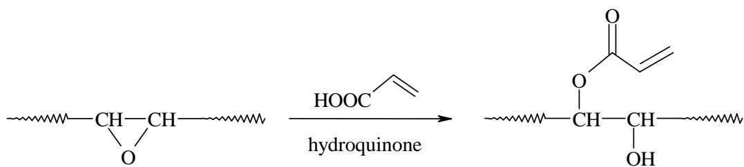
Figure 36 : Acrylation des huiles époxydées
