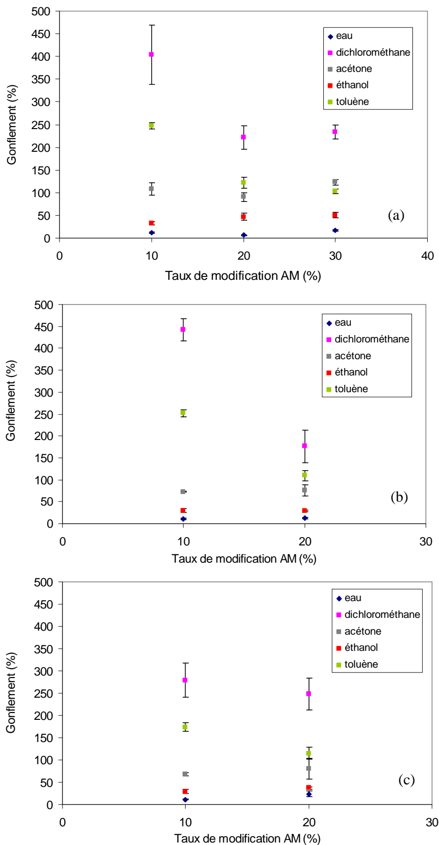
Figure 17 : Evolution du gonflement des matériaux standolisés à 30 % (a), 40 % (b) et 50% (c) et modifiés à différents taux de modification
