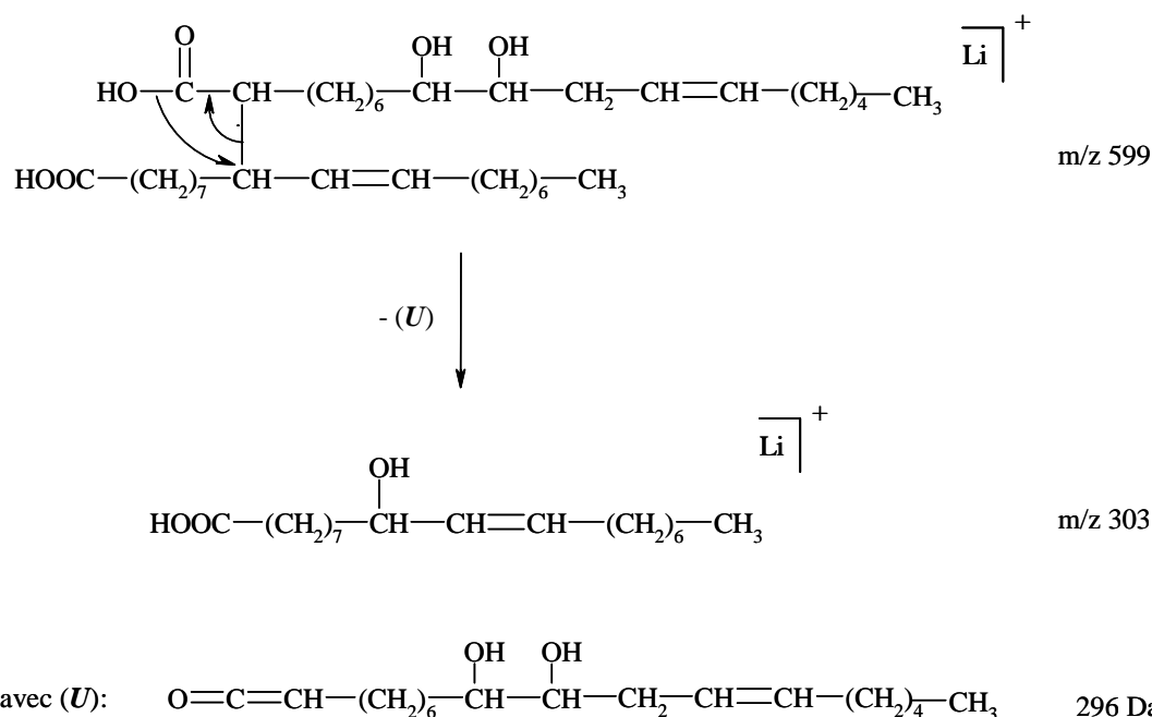
Figure 41 : Mécanisme de réarrangement à quatre centres permettant d'obtenir l'ion à m/z 303 à partir d'une espèce issue d'un couplage en \alpha de la fonction acide carboxylique
