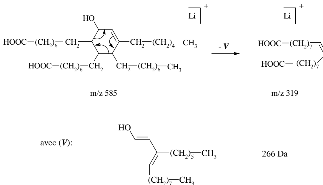
Figure 45 : Mécanisme d'obtention de l'ion à m/z 319
