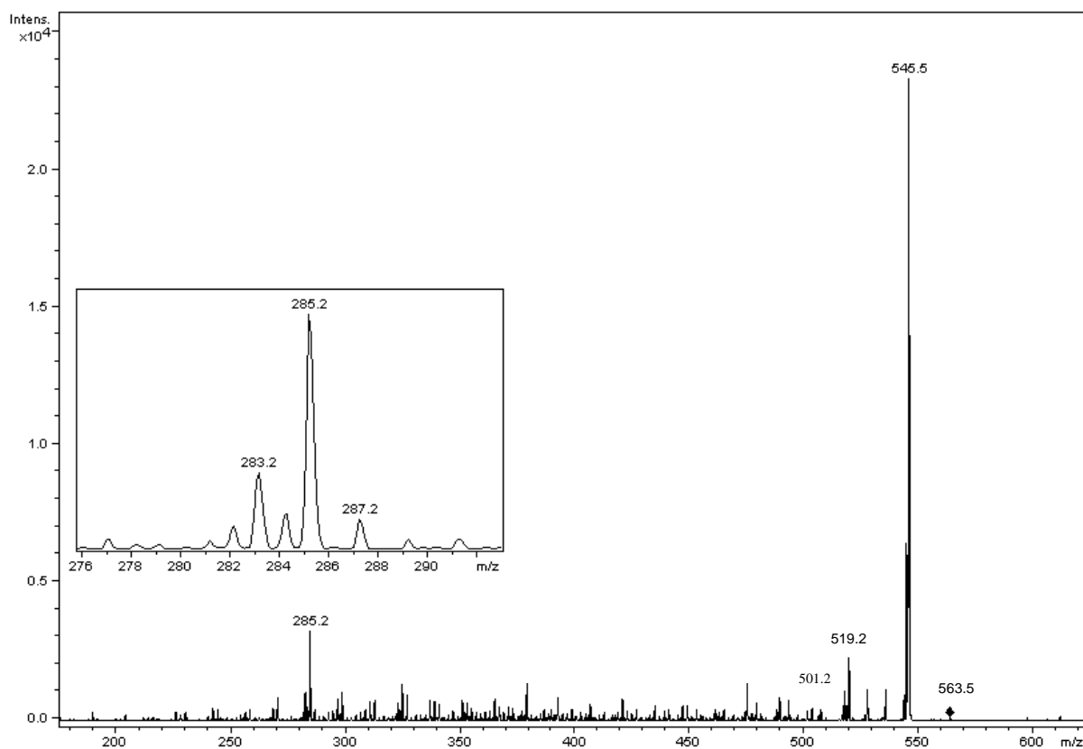
Figure 48 : Spectre MS 2 de l'ion à m/z 563
