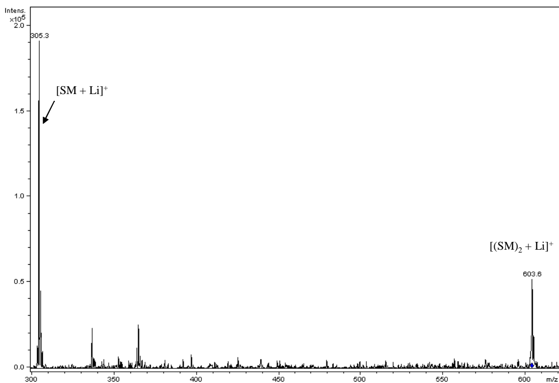
Figure 24 : Spectre MS du stéarate de méthyle après chauffage
