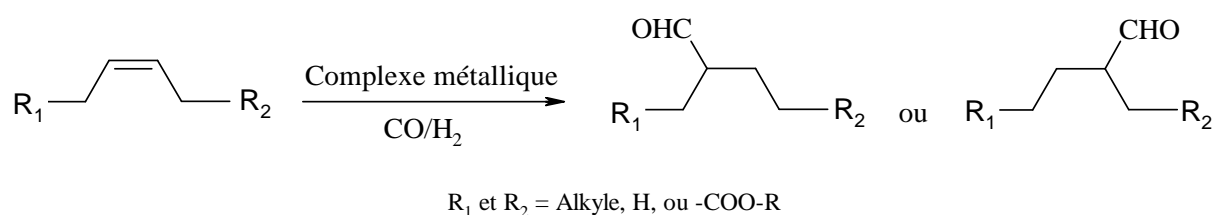
Figure 16 : Réaction d'hydroformylation sur les insaturations des huiles végétales
