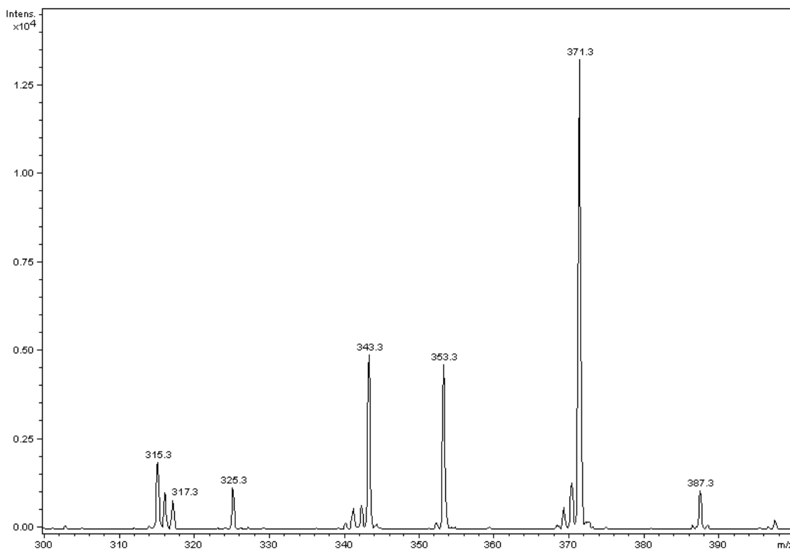
Figure 4 : Spectre MS^2 de l'ion à m/z 415
