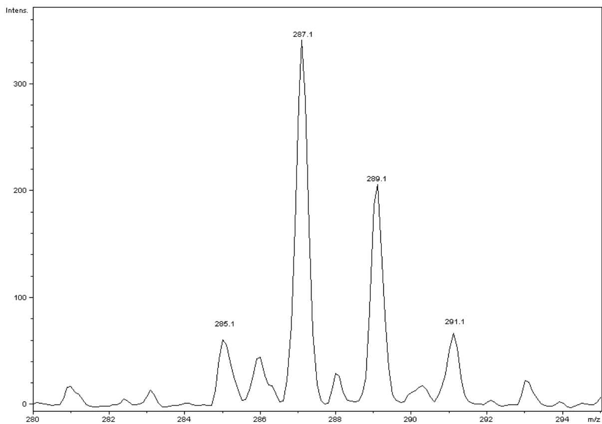
Figure 54 : Spectre MS^2 de l'ion à m/z 569
