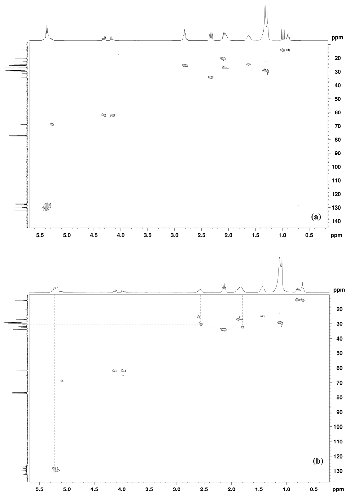
Figure 16 : Comparaison des spectres HMQC avant (a) et après (b) chauffage de l'huile de lin
