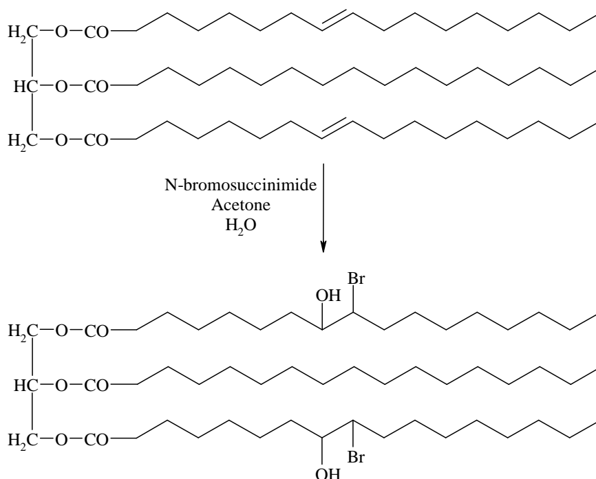
Figure 20 : Hydroxybromation des triglycérides
