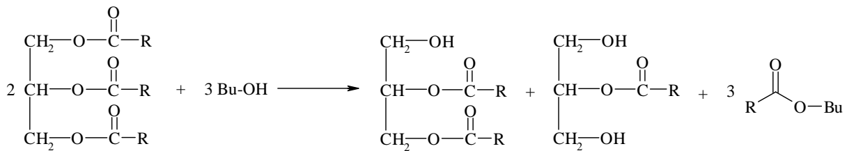
Figure 27 : Transestérification des triglycérides
