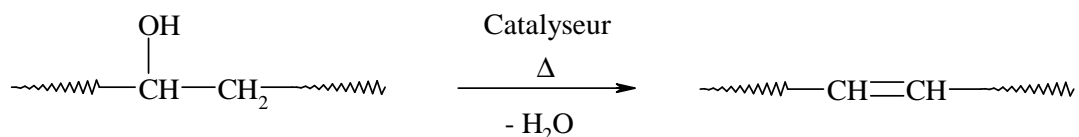
Figure 31 : Déshydratation des triglycérides
