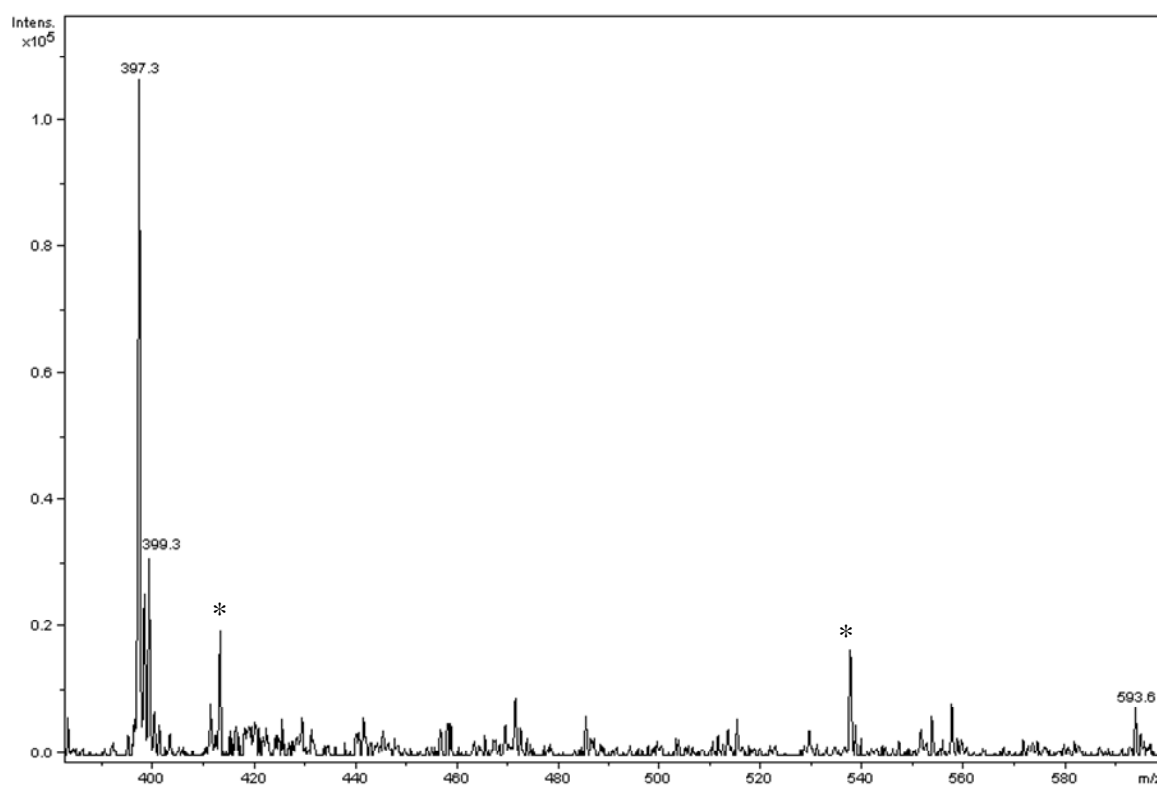
Figure 7 : Spectre MS du mélange réactionnel LM + AM (* : contaminants)
