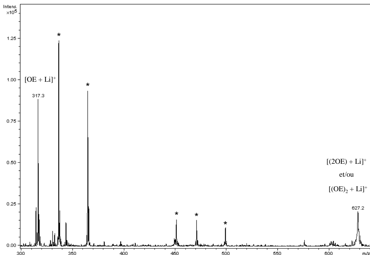
Figure 38 : Spectre MS de l'oléate d'éthyle après chauffage (* : contaminants)
