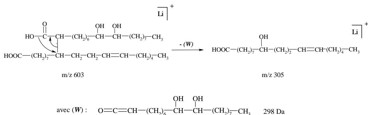
Figure 46 : Mécanisme d'obtention de l'ion à m/z 305
