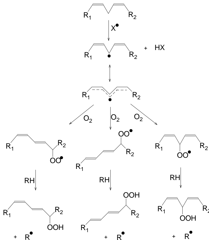
Figure 3 : mécanisme de formation d'hydroperoxydes
