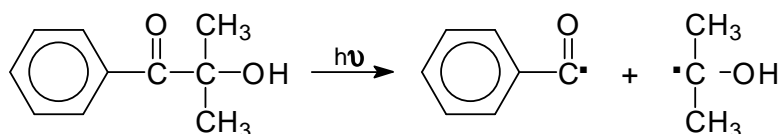
Figure 2 : décomposition du Darocur 1173 ® sous rayonnement UV
