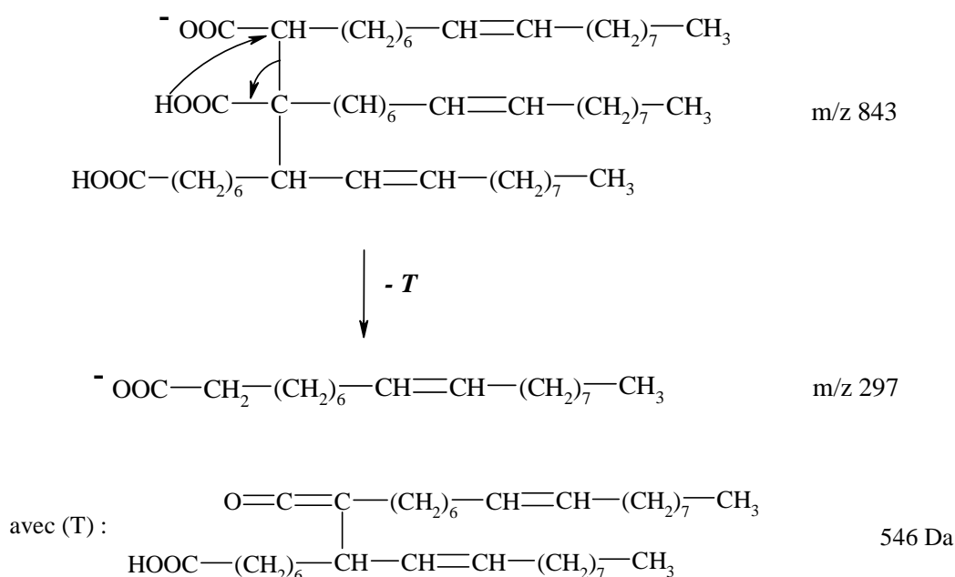
Figure 35 : Mécanisme de réarrangement à quatre centres permettant d'obtenir l'ion à m/z 297 à partir d'une espèce issue d'une réaction d'addition radicalaire suivie d'un couplage
