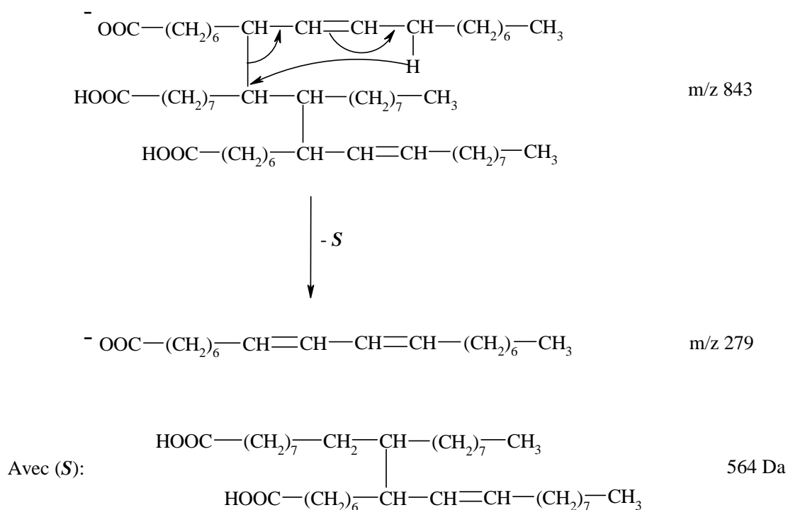
Figure 37 : Mécanisme de réarrangement à six centres permettant d'obtenir l'ion à m/z 279 à partir d'une espèce issue d'une addition radicalaire suivie d'un couplage
