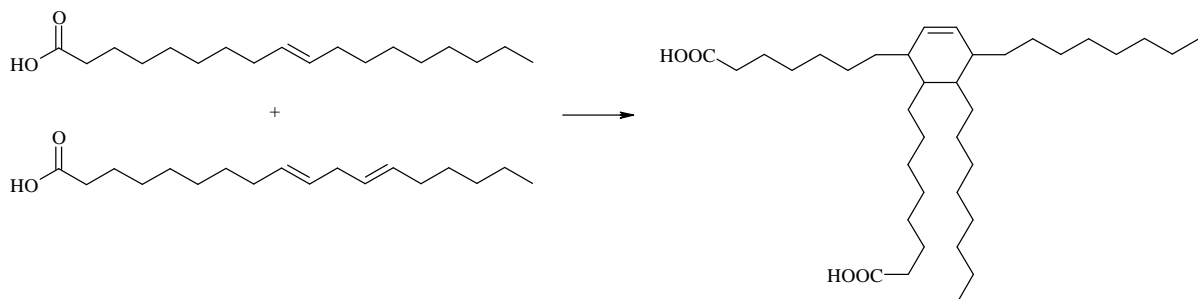
Figure 24 : Formation de dimères par réaction d'addition de Diels-Alder
