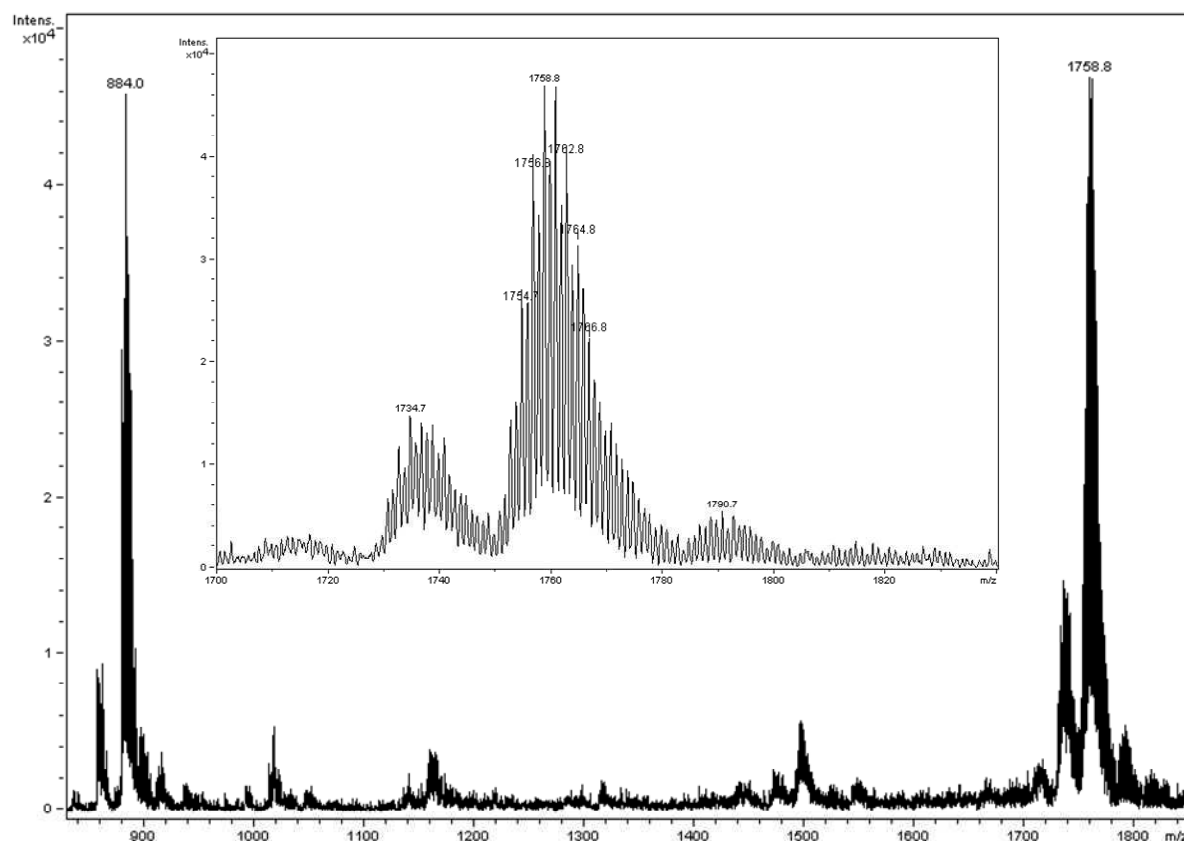
Figure 18 : Spectre MS de la solution lithiée l'huile de lin standolisée à 30 % de conversion en doubles liaisons
