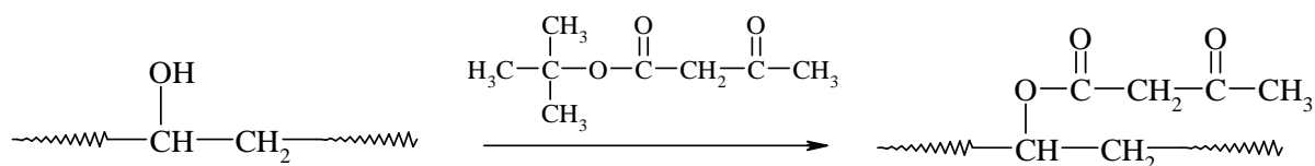
Figure 32 : Acétoacétylation de l'huile de ricin
