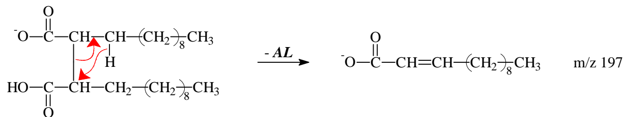
Figure 23 : Mécanisme d'obtention de l'ion à m/z 197
