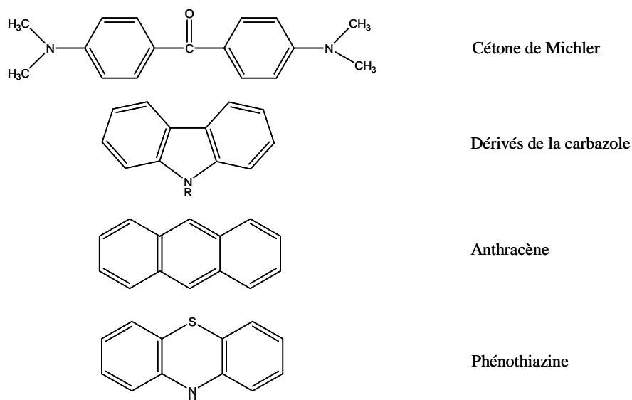
Figure 46: Exemples de photosensibilisateurs
