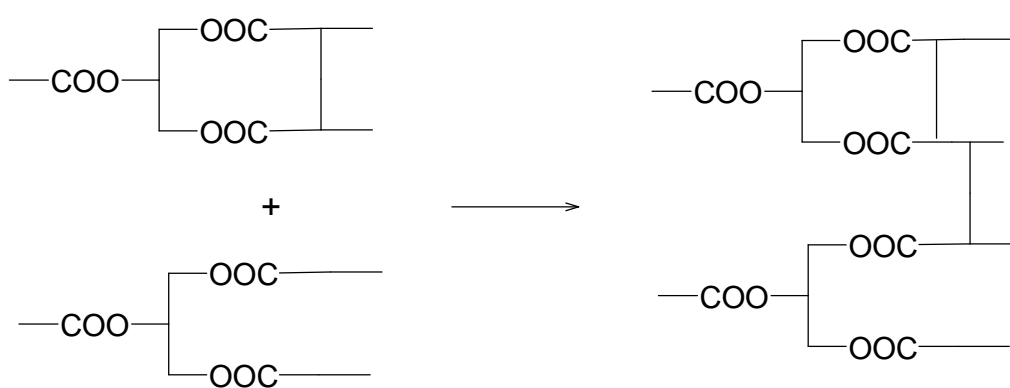
Figure 8 : Mécanisme réactionnel proposé par Pestemer et Tschinkel
