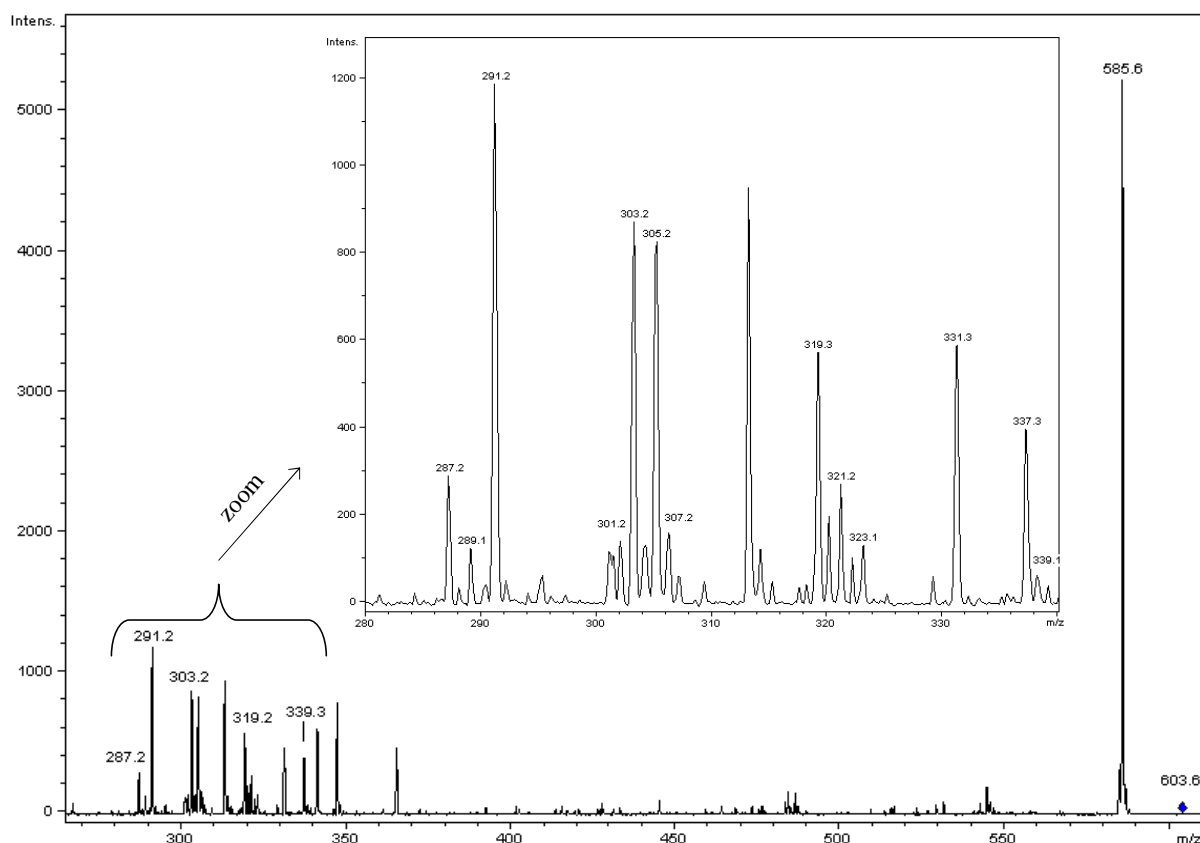
Figure 42 : Spectre MS^2 de l'ion à m/z 603
