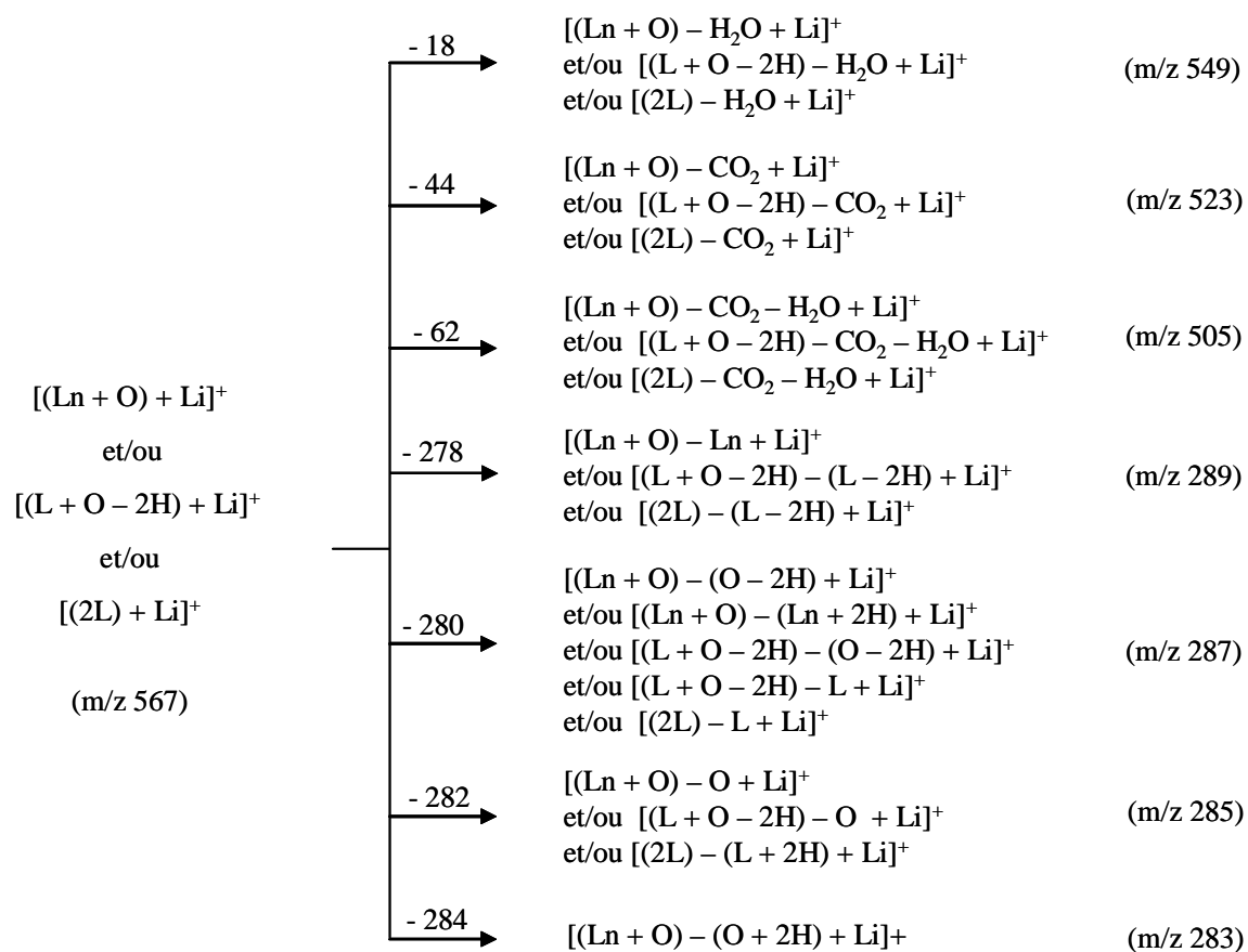
Figure 53 : Spectre MS 2 de l'ion à m/z 567
