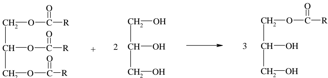
Figure 28 : Réaction de glycérolyse des huiles végétales
