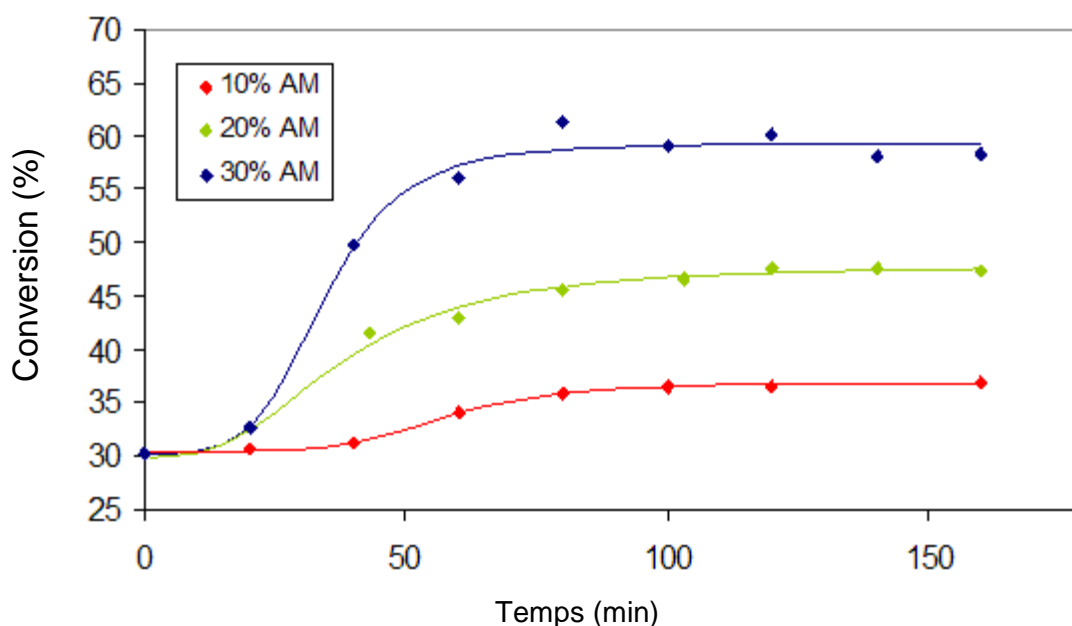
Figure 15 : Cinétique de modification de l'huile de lin standolisée à 30,3 % par l'anhydride maléique
