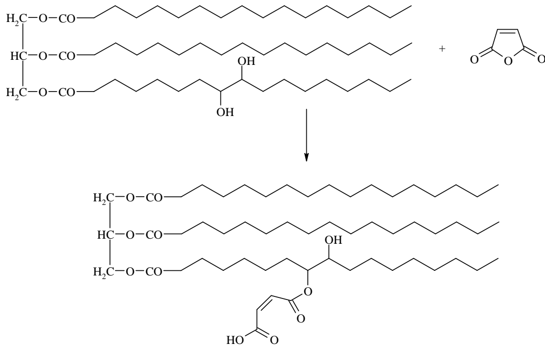
Figure 34 : Estérification des huiles hydroxylées par l'anhydride maléique
