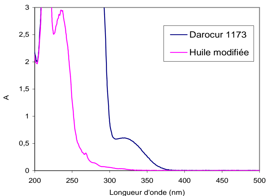
Figure 3 : spectres UV-visible du Darocur 1173 ® et de l'huile de lin modifiée dans l'acétonitrile
