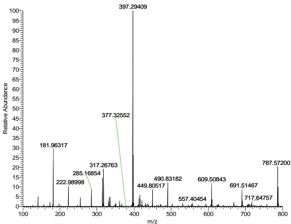
Figure 8 : Spectre HRMS du mélange réactionnel (LM + AM)
