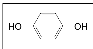
Figure 25 : Formule de l'hydroquinone
