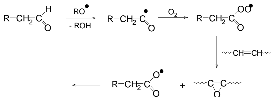
Figure 6 : Formation d'époxydes
