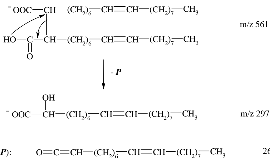
Figure 27 : Mécanisme de réarrangement à quatre centres permettant l'obtention de l'ion à m/z 297 à partir d'une espèce issue d'une réaction de couplage
