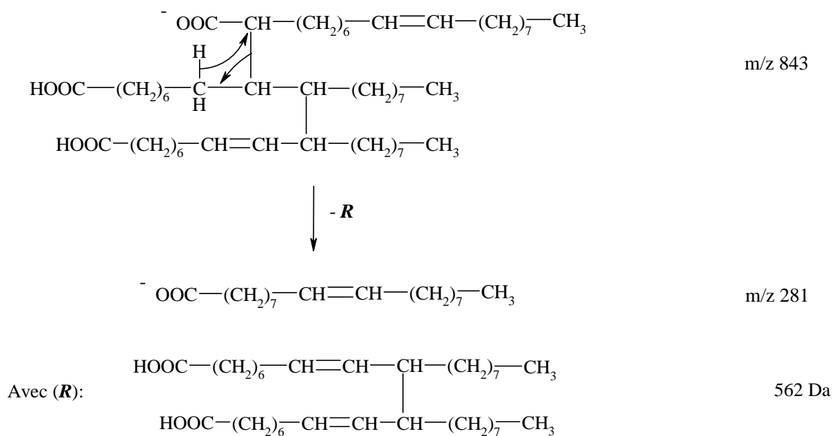
Figure 36 : Mécanisme de réarrangement à quatre centres permettant d'obtenir l'ion à m/z 281 à partir d'une espèce issue d'une addition radicalaire suivie d'une élimination
