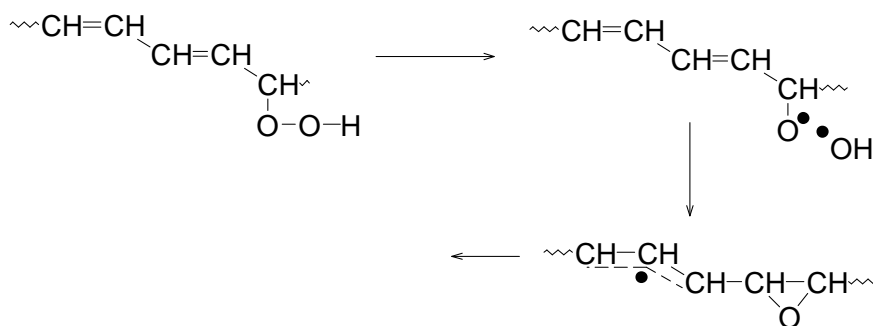
Figure 4 : Formation d'époxydes par réaction des hydroperoxydes sur les doubles liaisons
