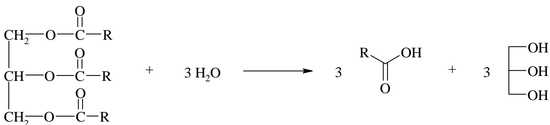
Figure 29 : Hydrolyse des triglycérides
