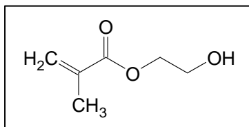
Figure 20 : Formule du méthacrylate d'hydroxyéthyle
