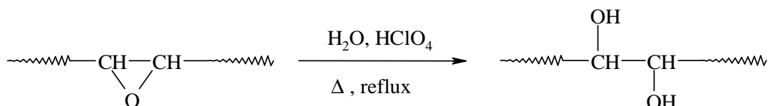
Figure 35 : Formation de deux fonctions hydroxyle par ouverture du cycle époxyde
