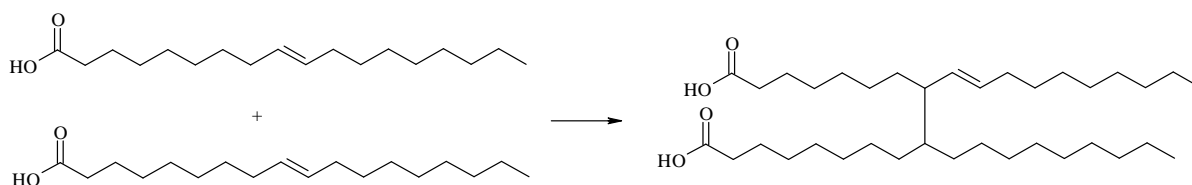
Figure 25 : Formation de dimères par réaction d'addition radicalaire
