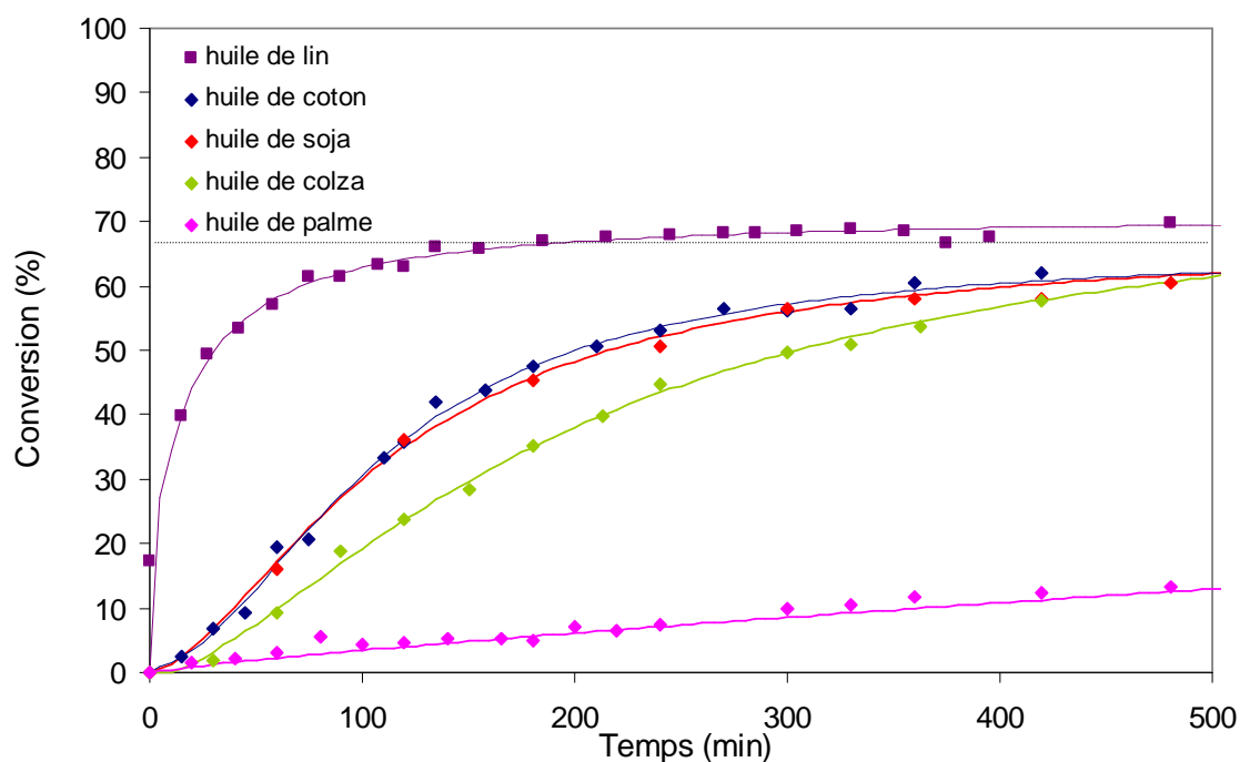
Figure 2 : Cinétique de standolisation des différentes huiles à 330°C
