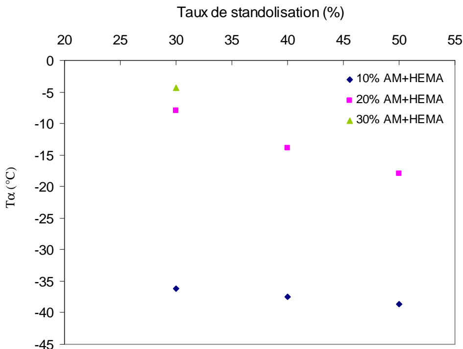
Figure 14 : Evolution de T_{\alpha} en fonction du taux de standolisation et du taux de modification de l'huile de lin
