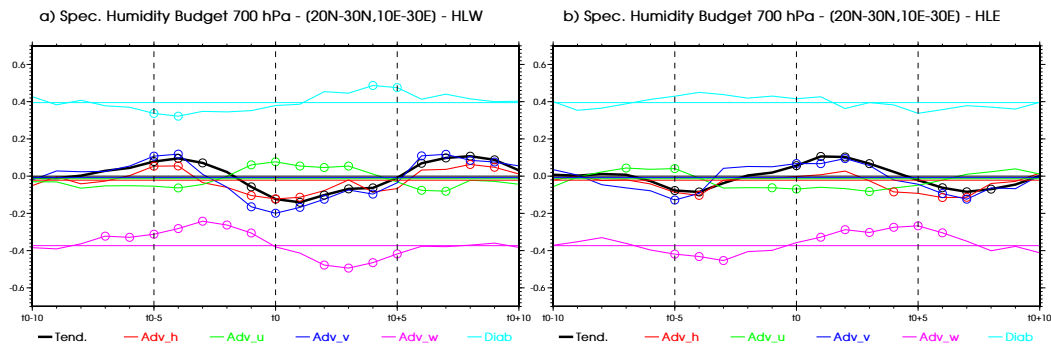
Figure 4.43 – Idem Fig. 4.42, mais pour le bilan composite de l’humidité spécifique à 700 hPa (en \text{g kg}^{-1} \text{ jour}^{-1} ), pour les évènements a) HLW et b) HLE.
