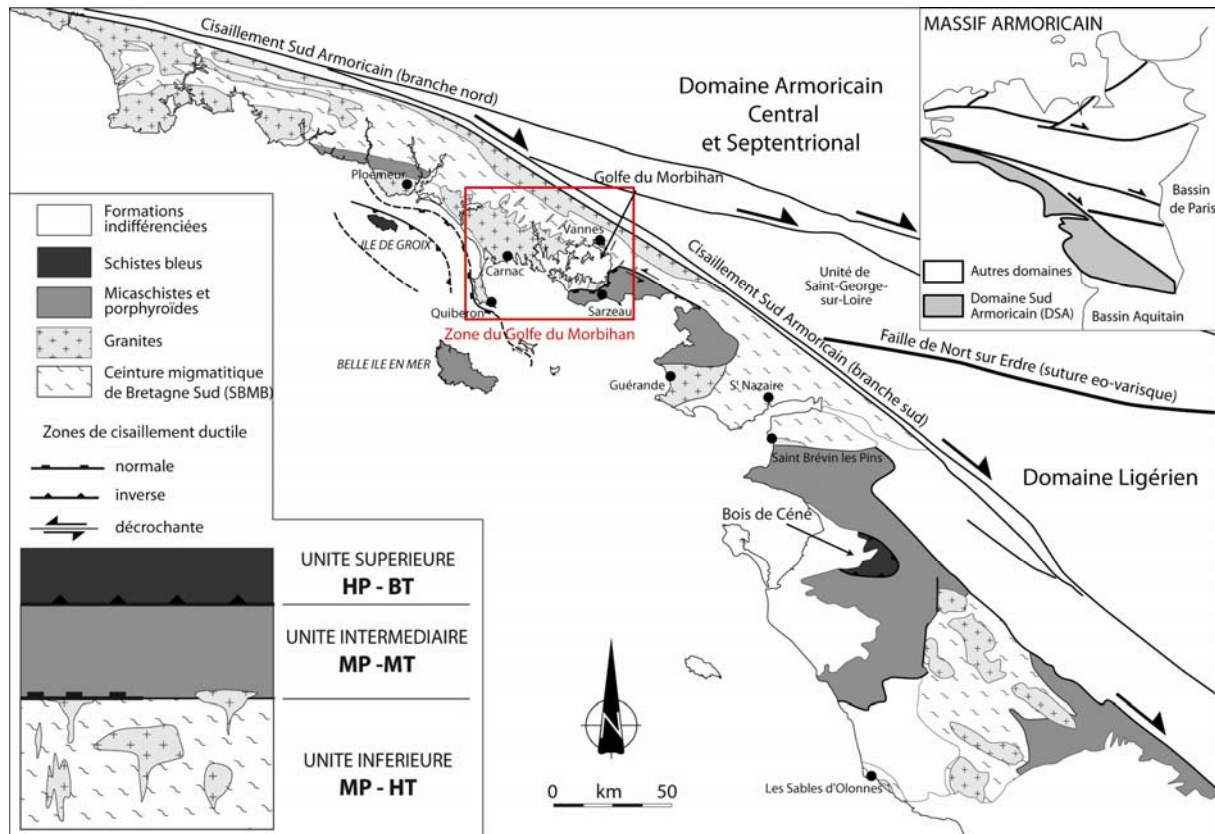
Figure II.1 : Localisation de la zone du Golfe du Morbihan (carte structurale du Domaine Sud Armoricaire modifiée d'après Gapais et al. (2009)).
