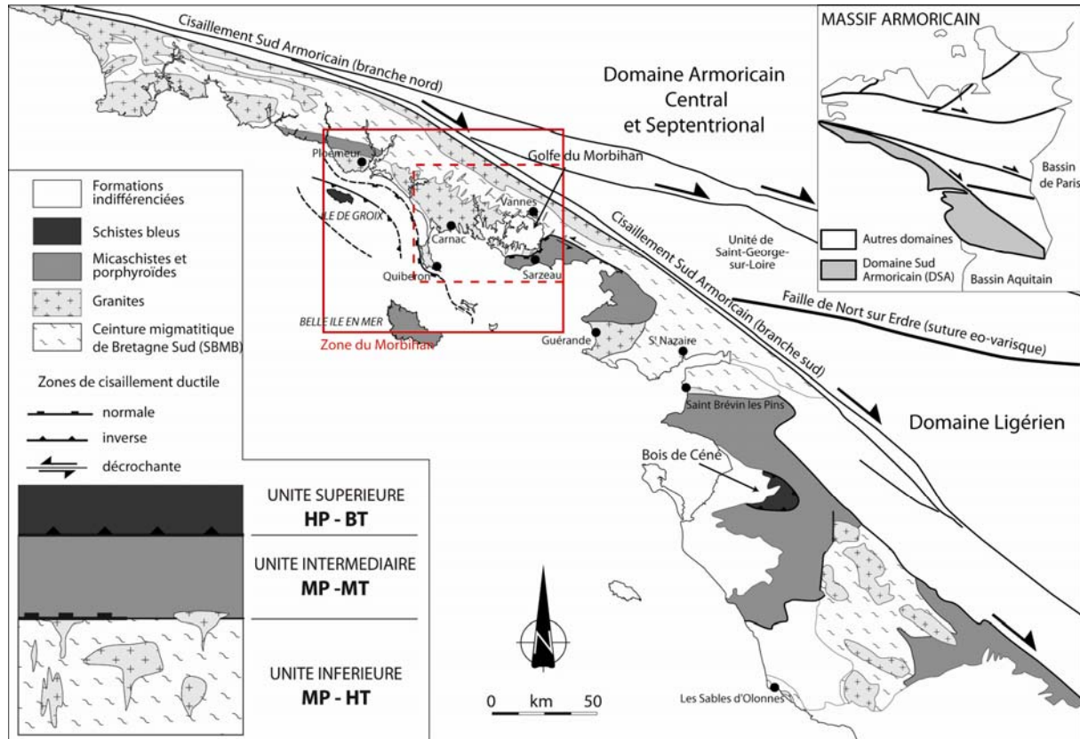
Figure IV.1 : Localisation de la zone du Morbihan (carte structurale du Domaine Sud Armoricaïn modifiée d'après Gapais et al. (2009)).
