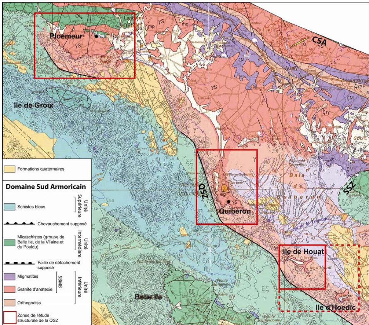
Figure IV.4 : Carte géologique à 1/250000 de la Marge continentale de Lorient (Thinon et al., 2008). Cette carte montre la trace présumée de la QSZ (d'après Thinon et al. (2008)) et la localisation des trois zones de notre étude structurale.
