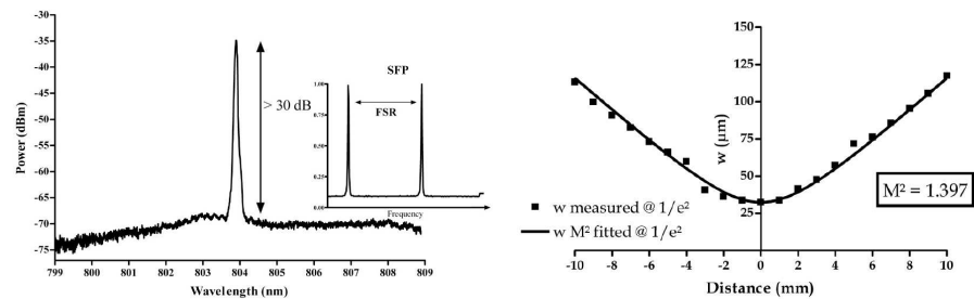
Fig. 3.21. Spectre d'une source à diode laser évasée montée en cavité auto-organisable. La puissance de sortie est de 1,2 W. Encart : spectre mesuré à l'aide d'un Fabry-Perot confocal à balayage. Mesure du facteur M_x^2 pour une puissance de sortie de 1,2 W.
