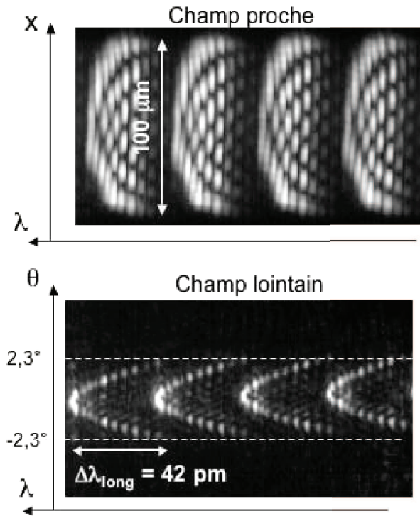
Fig. 3.10. Distributions d'intensité, résolues en longueur d'onde, en champ proche (image du haut) de la face de sortie d'une diode laser à ruban large de 100\ \mu\text{m} et en champ lointain (image du bas). La direction horizontale indique la longueur d'onde pour chaque mode. La direction verticale correspond à la direction latérale de la diode laser.
