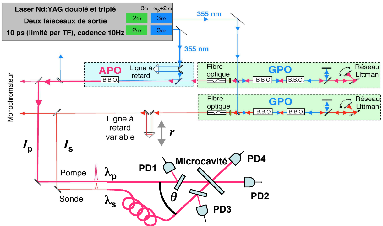
Fig. 6.14. Schéma du montage de type pompe-sonde en régime ps utilisé pour caractériser la transmission en régime non linéaire d'une microcavité doublement résonnante pour les faisceaux pompe et Stokes. Chaque faisceau est généré à partir d'une ligne de génération paramétrique. Les deux sources paramétriques sont pompées par un laser Nd :YAG pompé par flash, émettant des impulsions de durée voisine de 10 ps, dont le faisceau est doublé puis triplé en fréquence.
