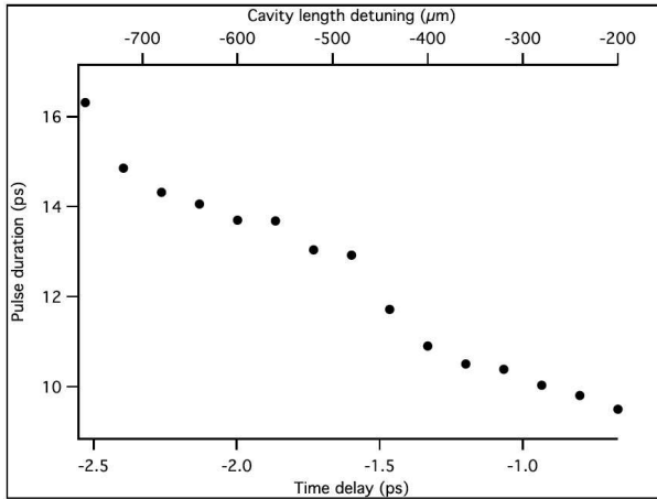
Fig. 6.3. Evolution des durées d'impulsion signal en fonction du désaccord de la longueur de la cavité OPO.
