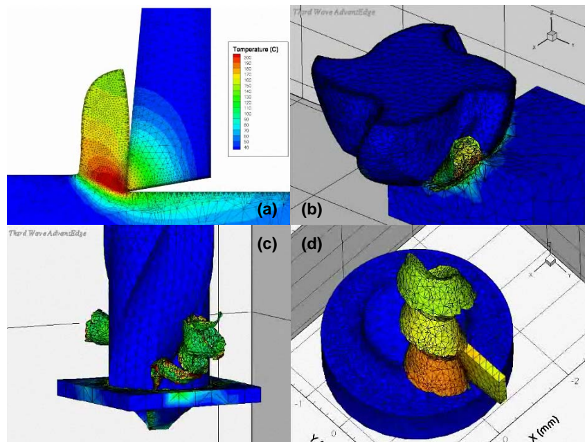
FIG. 1.11 – Quelques exemples de simulations avec le logiciel AdvantEdge TM .
