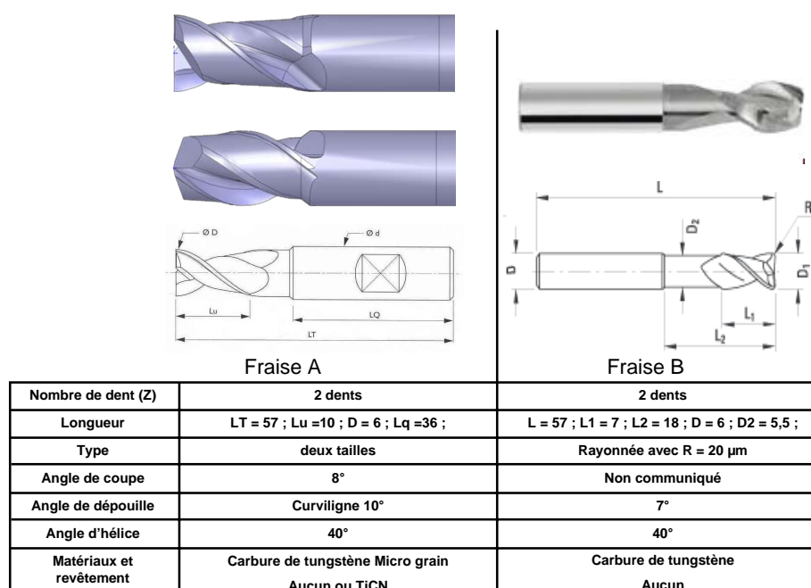
FIG. 3.2 – Descriptif des fraises utilisées pour les essais de fraisage.
