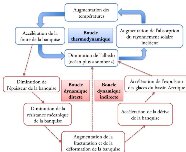
FIG. 1.4: Boucle de rétroaction de l'albédo illustrant les interactions entre les processus thermodynamiques (bleu) et les processus mécaniques (rouge) (Rampal, 2008).
