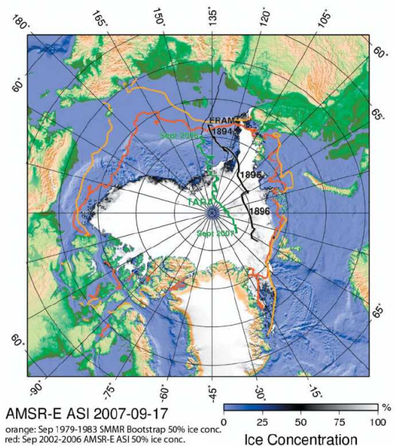
FIG. 1.3: Trajectoires de dérive du voilier Tara (de sept. 2006 à sept. 2007) et du Fram (1894-1896), superposées à la concentration de glace minimale de septembre 2007 estimée à partir de données AMSR-E (Gascard et al. , 2008).
