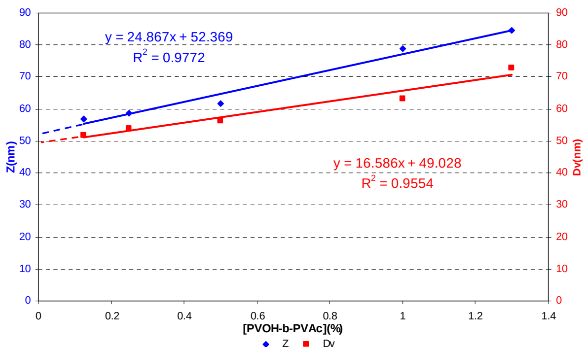
Figure VI-16 : Extrapolation à concentration nulle de la valeur Z et du diamètre hydrodynamique D_v des micelles de copolymère diblocs PVOH_{350}\text{-}b\text{-}PVAc_{60}
