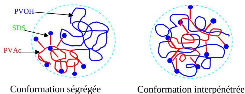
Figure VI-19 : Représentation schématique des conformation limites des copolymères PVOH- b -PVAc dont la séquence PVAc est complexée par le SDS
