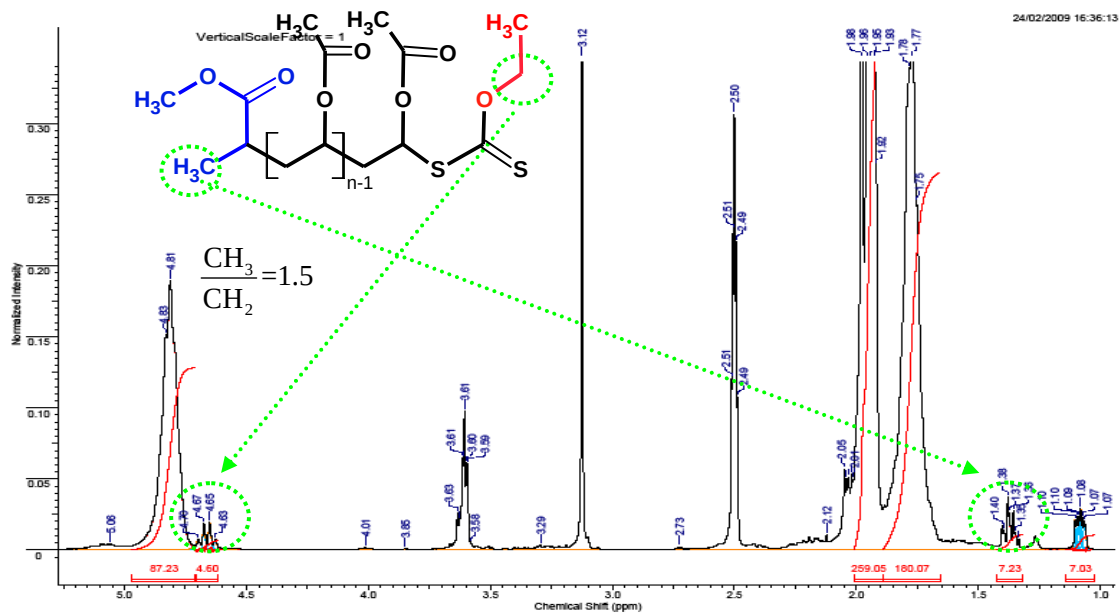
Figure A-VI-1 : Spectre RMN ^1\text{H} d'un PVAc fonctionnnalisé xanthate
