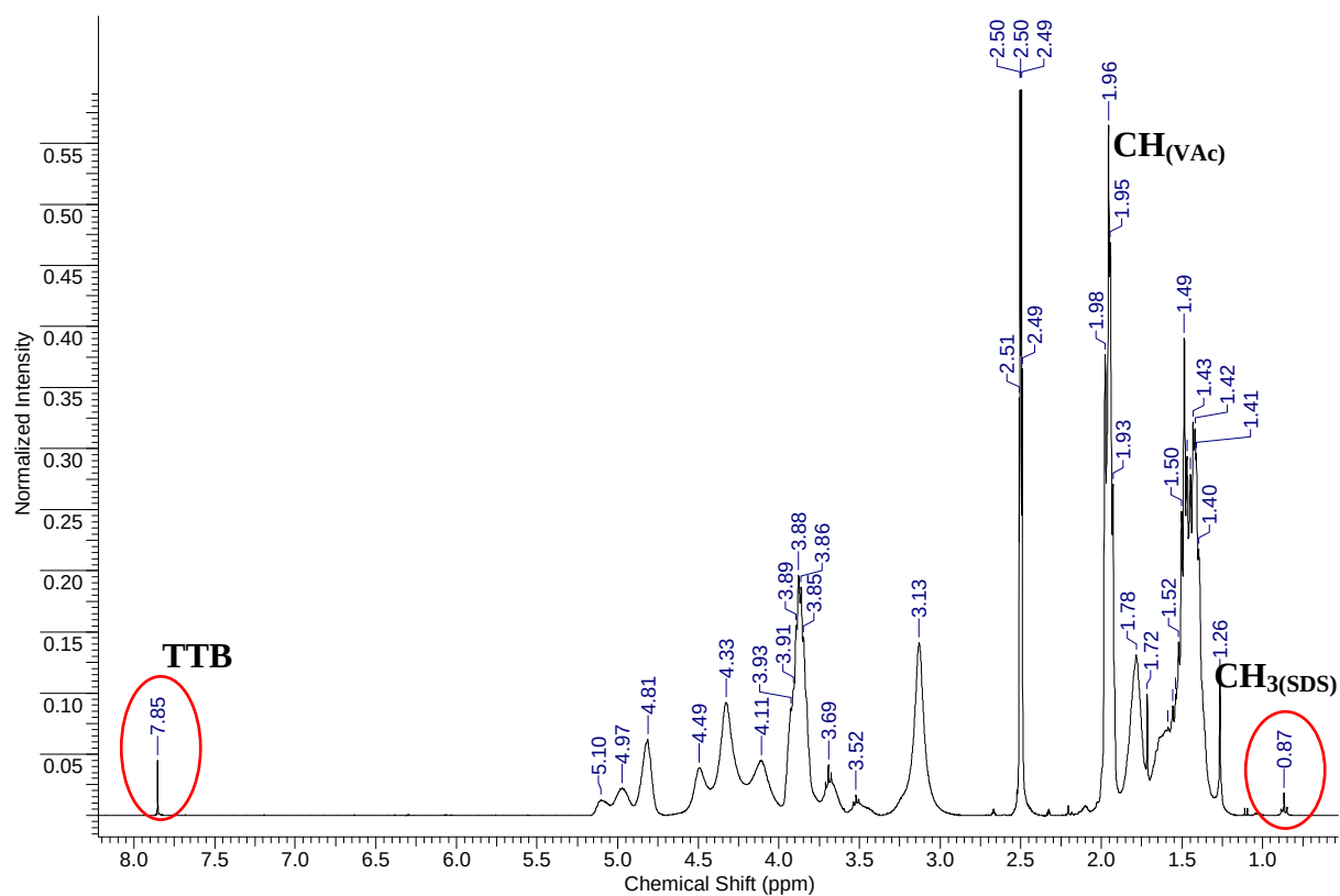
Figure A-V-1 : Spectre RMN ^1\text{H} de la fraction \text{FC}_3 du PVA-73-685 en présence de la référence TTB :
