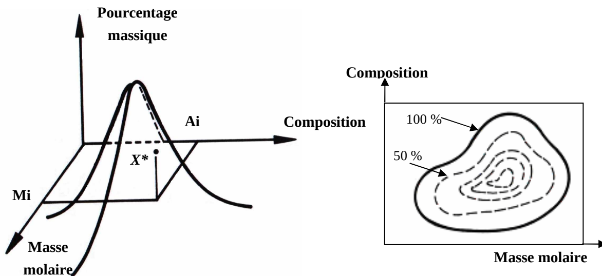
Figure I-3a : Surface de distribution en 3 dimensions
