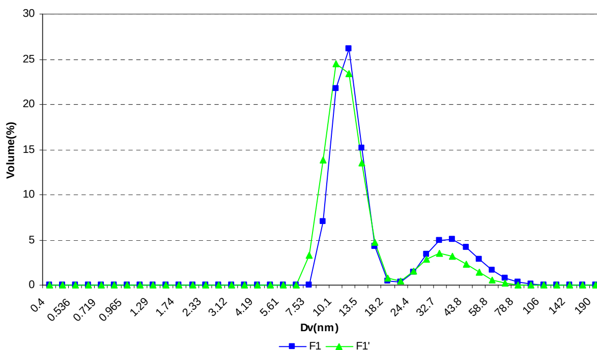
Figure V-7 : Courbes de distribution des tailles en volume par DLS pour le coacervat F_1 et le surnageant F_1' , issus du PVA-73-685 à une concentration massique de 1 % à 20°C
