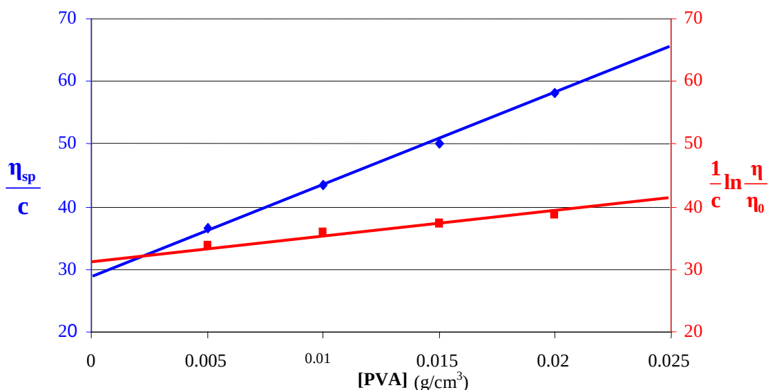
Figure II-5: Détermination de [\eta] du KP08 en milieu aqueux à partir des relations de Huggins et de Kraemer
