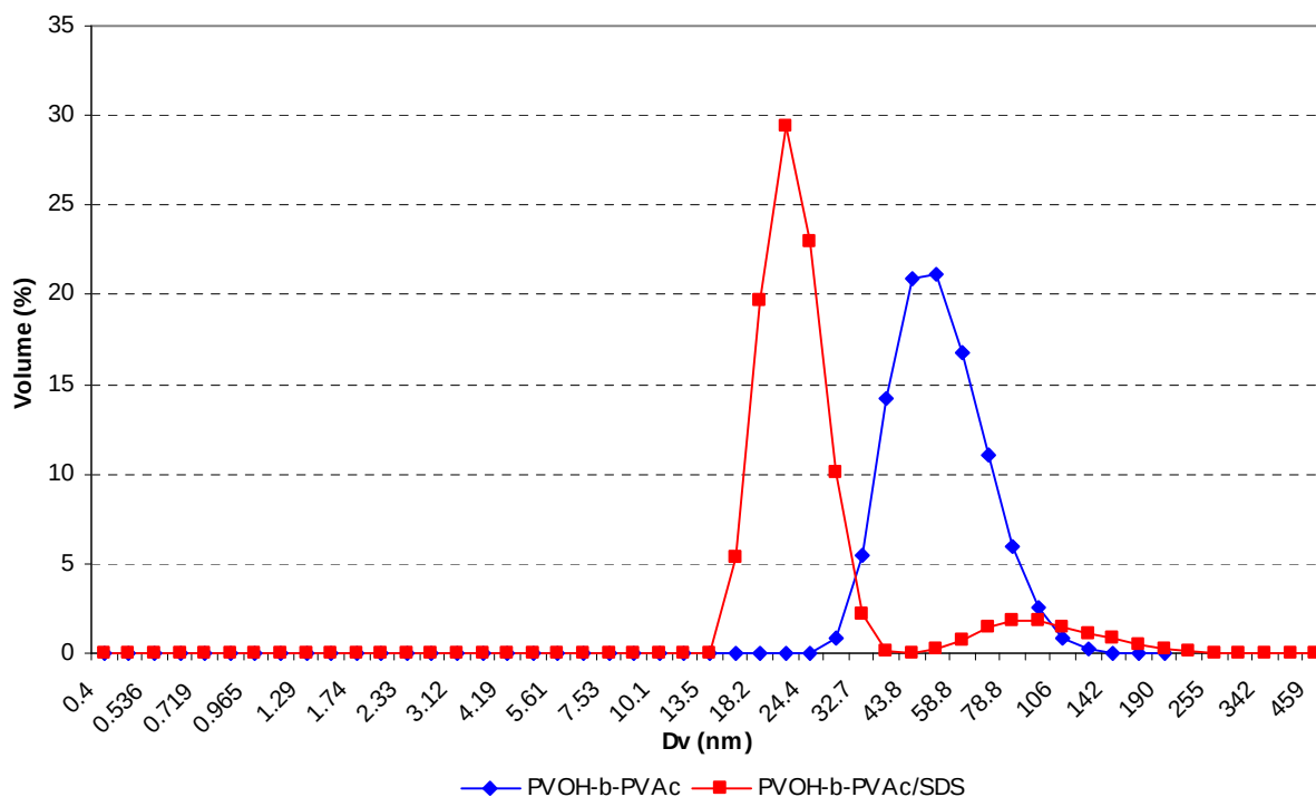
Figure A-VI-3 : Courbes de distribution des tailles en volume pour les micelles de copolymère PVOH_{350} - b - PVAc_{60} en absence et en présence de SDS à une concentration massique de 1 % par rapport au copolymère
