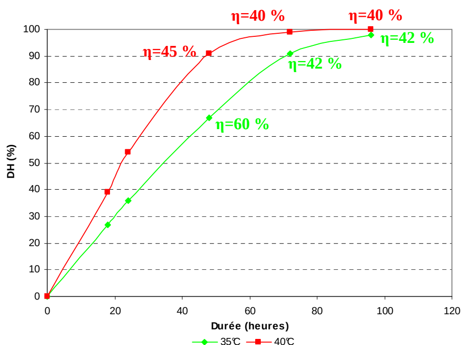
Figure VI-9 : Evolution du taux de fonctionnalisation xanthate \eta en fonction du DH et de la durée de l'hydrolyse
