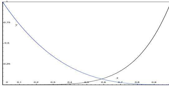
FIGURE 1.1 – k_1(s_1) perméabilité de la phase 1(croissante) k_2(s_1) perméabilité de la phase 2 (décroissante)
