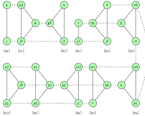
FIG. 7.1 – Le programme de référence, son graphe d'interférence-affinité et son graphe éclaté. Le graphe éclaté donne une bonne représentation du flot de données du programme.
