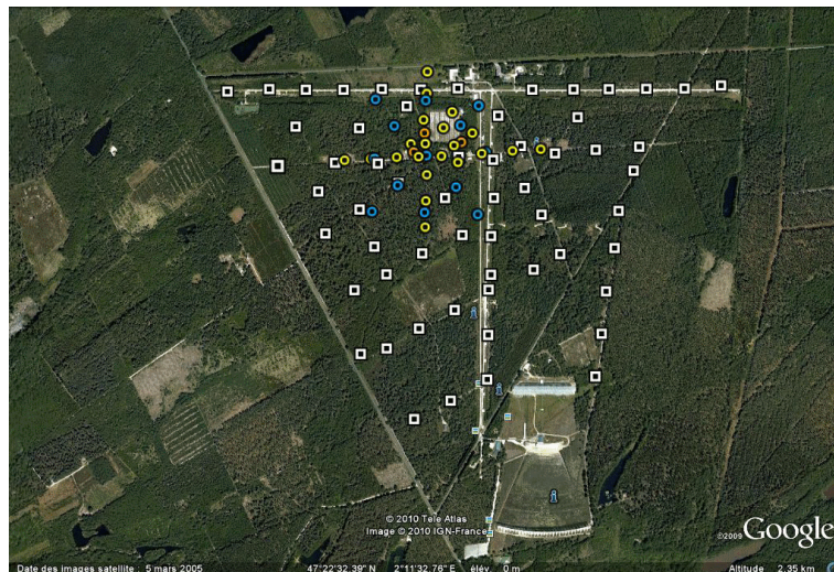
FIGURE 4.49 – Emplacement des 60 futures stations autonomes (carrés blanc) sur l'Observatoire de Nançay. Les scintillateurs sont indiqués par des cercles rouge.
