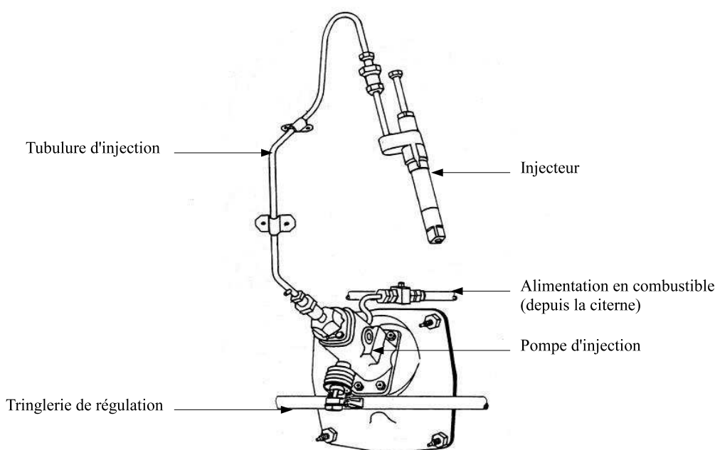
Figure 2.7 – Système d'injection.
