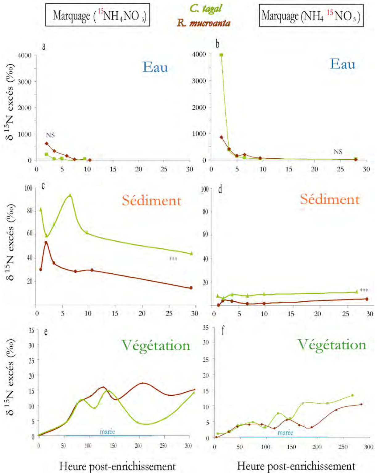
• Figure 4.28 : Résultats du traçage isotopique dans les compartiments eau, sédiments et végétation dans les faciès à C. tagal et R. mucronata . Delta ^{15}\text{N}_{\text{excès}} (‰) moyen calculé à partir des mesures d'abondance isotopique effectuées sur les échantillons d'eau, de sédiment et de feuilles en fonction du temps post enrichissement au ^{15}\text{NH}_4\text{NO}_3 et \text{NH}_4^{15}\text{NO}_3 .
