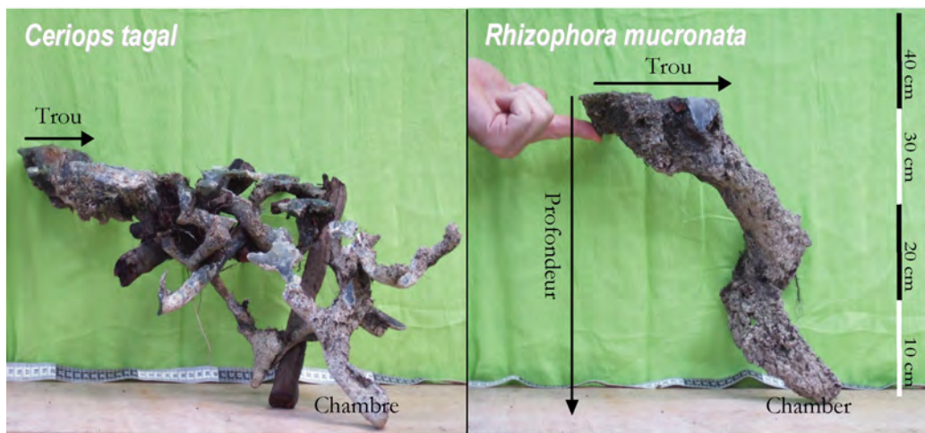
Figure 6.7: Moulage en résine polyester montrant l'architecture typiques et les caractéristiques (largeur du trou, profondeur et surface) des terriers de crabes dans les faciès C et R (photo : avril 2007)
