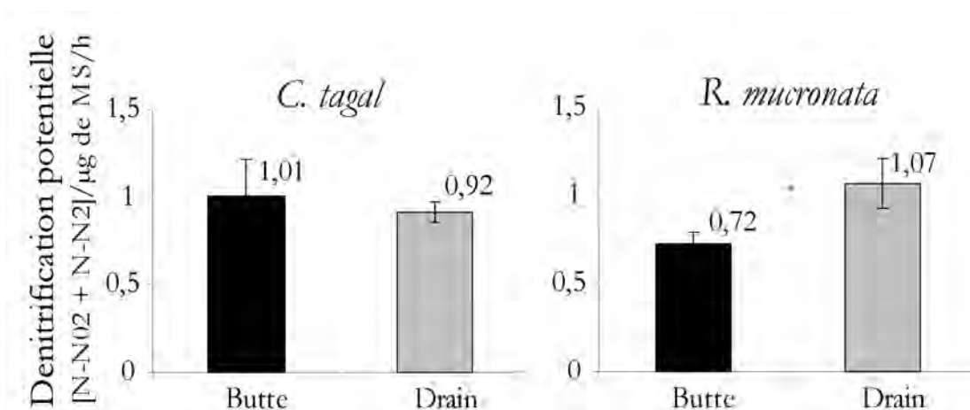
Figure 4.25 : Dénitrification potentielle en fonction de la microtopographie du sol (butte en gris et drain en noir) à de 0-5 cm de profondeur, dans les faciès à C. tagal et R. mucronata . (Avril 2008, n=6 , * p \leq 0,01 ).
