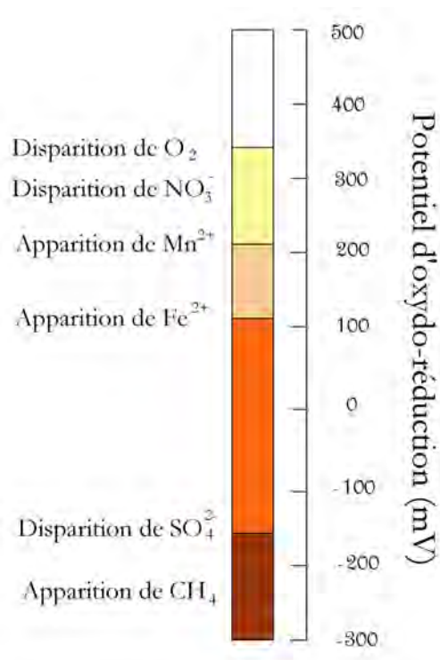
Figure 4.33 : Changement chimiques dans le sédiment selon les différents niveaux du potentiel d'oxydoréduction du sédiment. (Eh, corrigé à pH7). (D'après Delaune et al. , 1976, redessiné par Youssef, 1995).
