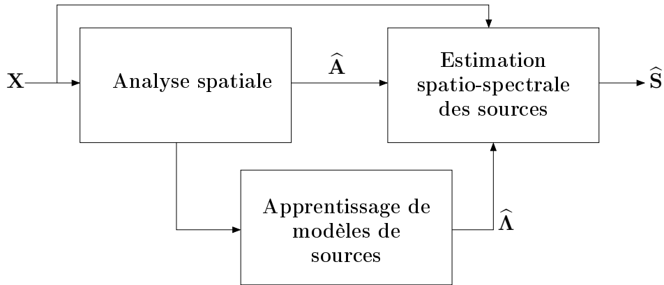
FIG. 14 – Architecture de la méthode de séparation spatio-spectrale que nous proposons. \mathbf{X} est le mélange multicanal, \hat{\mathbf{A}} est l'estimation de la matrice de mélange, \hat{\mathbf{\Lambda}} est l'estimation des modèles de sources, \hat{\mathbf{S}} est l'estimation des sources.
