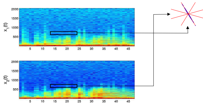
FIG. 8 – Approche locale de Deville. les directions sont estimées à partir du diagramme de dispersion des points contenus dans une région temps-fréquence où une seule source est active.
