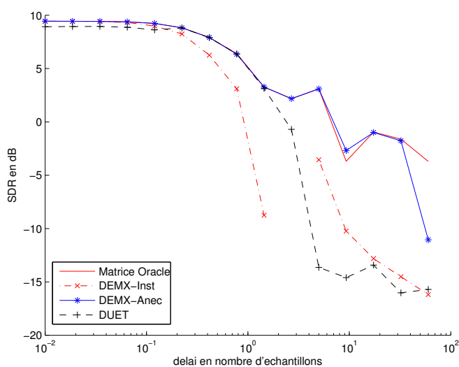
FIG. 7.4 – SDR en fonction de la valeur absolue du délai \delta des deux sources latérales
