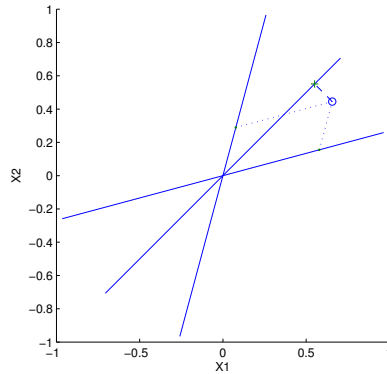
FIG. 10 – Estimation des coefficients des sources par la méthode DUET, pour un point temps-fréquence donné. Le coefficient du mélange (o) est projeté orthogonalement sur la direction la plus proche (ici la direction du milieu correspondant à la source S_2 ). La distance du point projeté (+) à l’origine est la valeur attribuée à la source S_2 , alors qu’une valeur nulle est attribuée aux autres sources. Les valeurs estimées par cette méthode sont les plus vraisemblables si l’on suppose qu’une seule source au plus est active (a une valeur non nulle). Or dans l’exemple ci-dessus, les sources S_1 et S_3 sont actives, tandis que la source S_2 est inactive.
