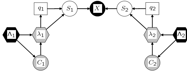
FIG. 8.1 – Réseau bayésien représentant l'adaptation contrainte. Formes des nœuds : processus continus (ronds), processus discrets (carrés), modèles (hexagones). Coloration des nœuds : nœuds observés (noir), nœuds cachés estimés (gris), autres nœuds cachés (blanc).
