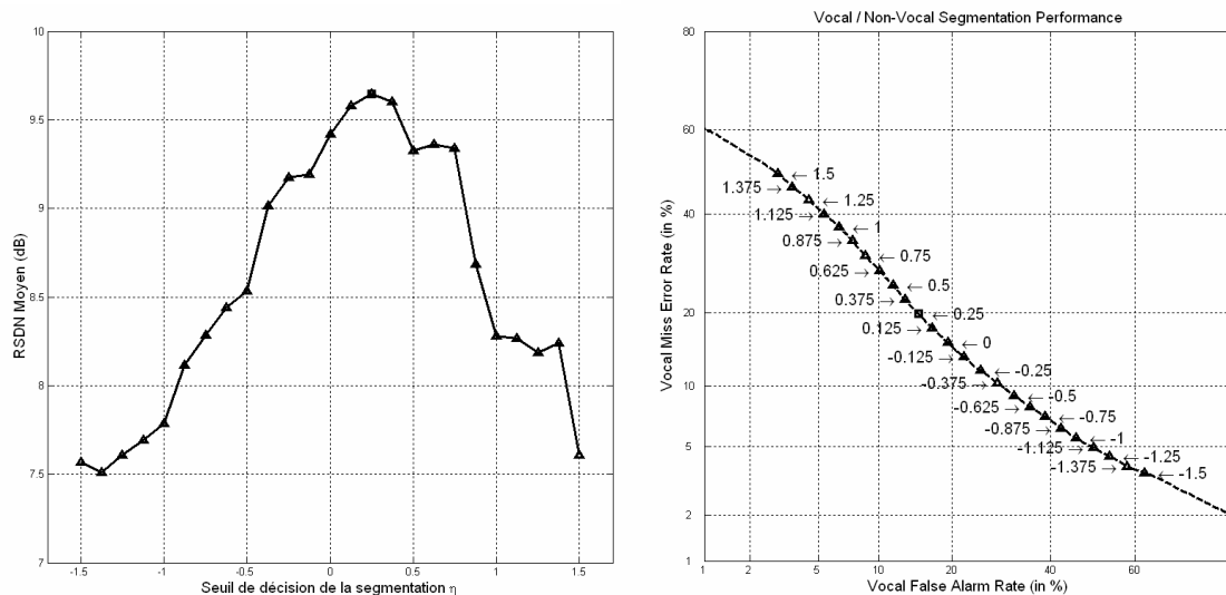
FIG. 12.1 – Performances de séparation en fonction du seuil de décision de la segmentation automatique. A gauche : RSDN moyen en fonction du seuil \eta . A droite : points de fonctionnement sur la courbe DET correspondants aux seuils de décision testés.
