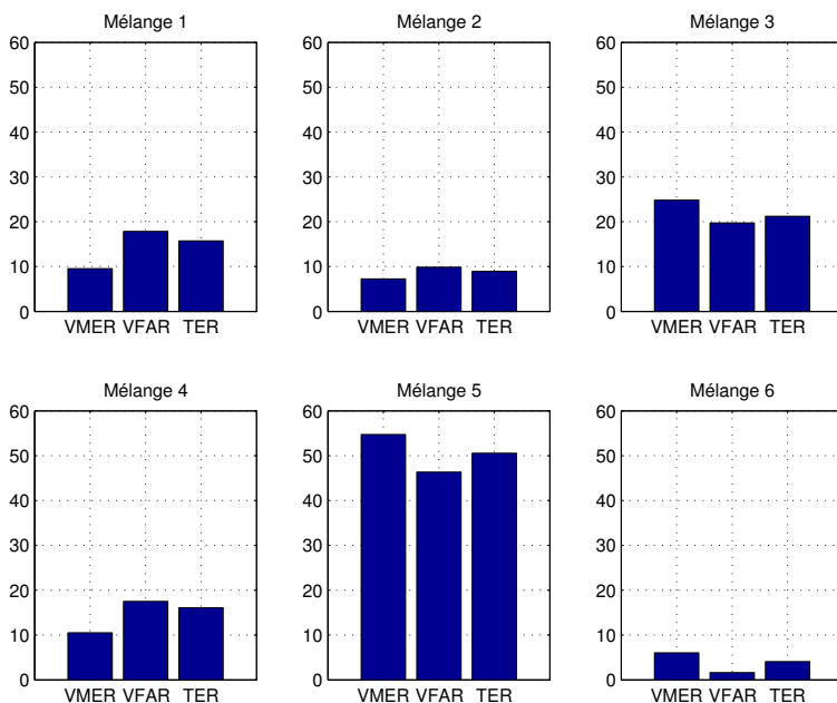
FIG. 12.4 – Performances de segmentation en parties vocales et non vocales pour chaque chanson de test : VMER ( Vocal Miss Error Rate ), VFAR ( Vocal False Alarm Rate ) et TER ( Total Error Rate ).
