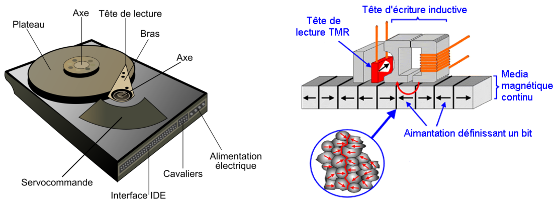
FIGURE 1.19 – Schéma d'un disque dur (Source : Wikipedia) et zoom au niveau de la tête de lecture/écriture (Source : E. Grochowski et R. E. Fontana, Nanofilms in Giant Magnetoresistance Heads, Dekker Encyclopedia of Nanoscience and Nanotechnology).
