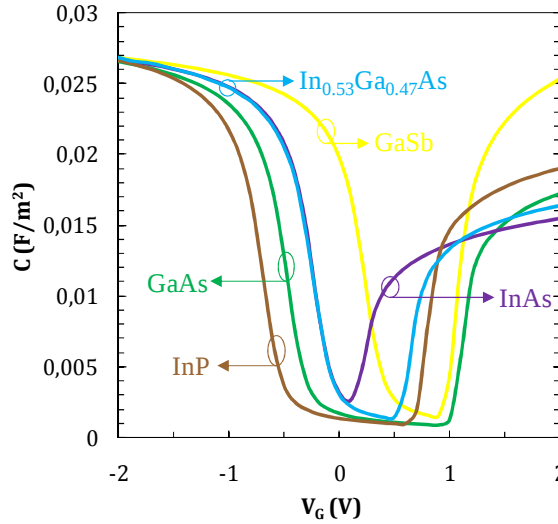
Figure 2.14 : Caractéristiques C-V simulées (Poisson-Schrödinger) pour différents semiconducteurs III-V (GaAs en vert, \text{In}_{0.53}\text{Ga}_{0.47}\text{As} en bleu, InAs en violet, GaSb en jaune et InP en marron) dopés de type p ( N_A = 1 \times 10^{17} \text{ cm}^{-3} ) avec une couche d'oxyde [ T_{\text{Al}_2\text{O}_3} = 2.3 \text{ nm} ( \text{EOT} \sim 1 \text{ nm} )] et un travail de sortie fixe pour toutes les structures ( \Phi_M = 5.0 \text{ eV} ).
