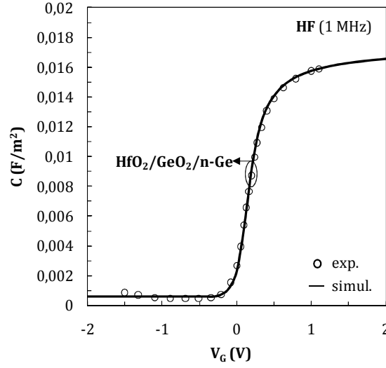
Figure 2.13 : Caractéristiques C-V expérimentales (ronds) [Xie] et simulées (Poisson-Schrödinger) d'une capacité \text{HfO}_2/\text{GeO}_2/\text{Ge} à haute fréquence (1 MHz) avec : T_{\text{HfO}_2} = 4.5 \text{ nm} , T_{\text{GeO}_2} = 2.0 \text{ nm} , N_A = 1 \times 10^{16} \text{ cm}^{-3} .
