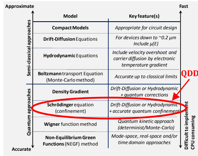
Figure 3.1 : Classification hiérarchique des modèles de transport [Vasileska].
