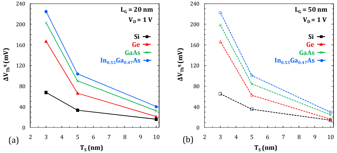
Figure 3.16 : Comparaison des différents matériaux semiconducteurs (même code couleur que la figure 3.13) en termes d'écart entre les tensions de seuil classique et quantique \Delta V_{Th}^q (extraites à V_D = 1 V) en fonction de l'épaisseur du film semiconducteur T_s dans les transistors MOS DG avec (a) L_G = 20 nm et (b) L_G = 50 nm.
