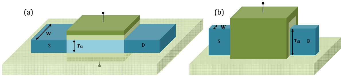
Figure 1.6 : Représentation schématique (a) du transistor MOSFET en architecture Double-Grille plane et (b) du transistor FinFET (dispositif Triple-Grille non-planaire) où sont représentées les largeurs W et les épaisseurs du film semiconducteur T_{Si} (avec S pour région de source et D pour région de drain).
