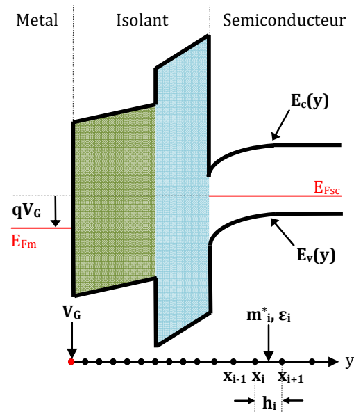
Figure 2.9 : Diagramme de bande schématisant une structure MIS (semiconducteur dopé de type p) pour V_G > 0 et représentation du maillage 1D (uniforme dans les oxydes et non-uniforme dans le semiconducteur).
