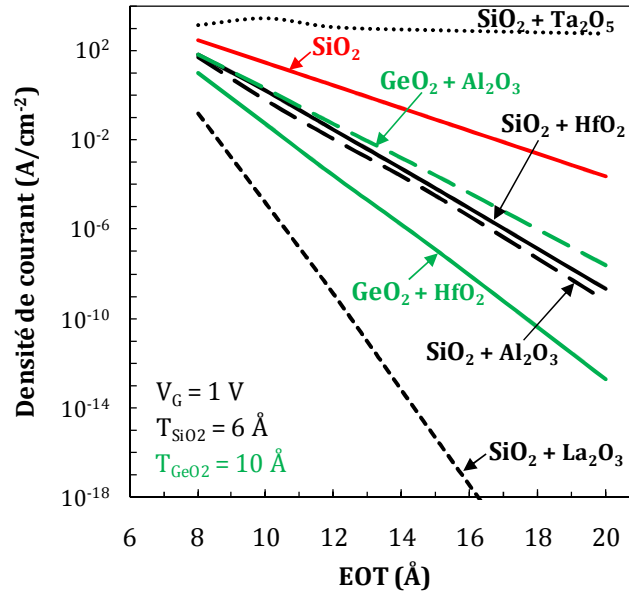
Figure 2.28 : Comparaison de la densité de courant de fuite en fonction de l'EOT (à V_G = 1 V) dans différentes capacités MIM avec les empilement de grille suivants : \text{SiO}_2 (rouge), \text{SiO}_2 + \text{HfO}_2 (traits continus noirs), \text{SiO}_2 + \text{Al}_2\text{O}_3 (pointillés larges noirs), \text{SiO}_2 + \text{La}_2\text{O}_3 (pointillés courts), \text{SiO}_2 + \text{Ta}_2\text{O}_5 (points), \text{GeO}_2 + \text{HfO}_2 (traits continus verts), \text{GeO}_2 + \text{Al}_2\text{O}_3 (pointillés larges verts) ( T_{\text{SiO}_2} = 6 Å et T_{\text{GeO}_2} = 10 Å pour les structures à deux couches).
