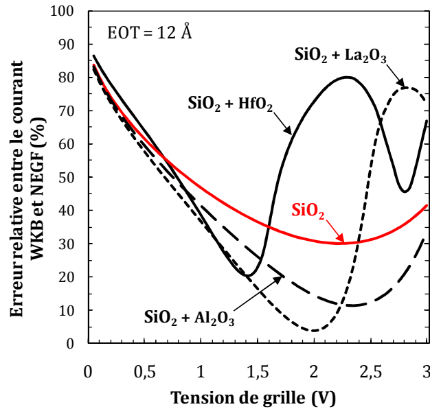
Figure 2.24 : Erreur relative entre le calcul du courant avec la transparence WKB et NEGF en fonction de la tension de grille dans des capacités MIM à deux couches ( T_{\text{SiO}_2} = 6 \text{ \AA} et \text{EOT} = 1.2 \text{ nm} ) avec différents matériaux high- \kappa : \text{HfO}_2 (traits continus), \text{Al}_2\text{O}_3 (pointillés larges) et \text{La}_2\text{O}_3 (pointillés courts). La structure de référence (simple couche de \text{SiO}_2 ) est également représentée en rouge.
