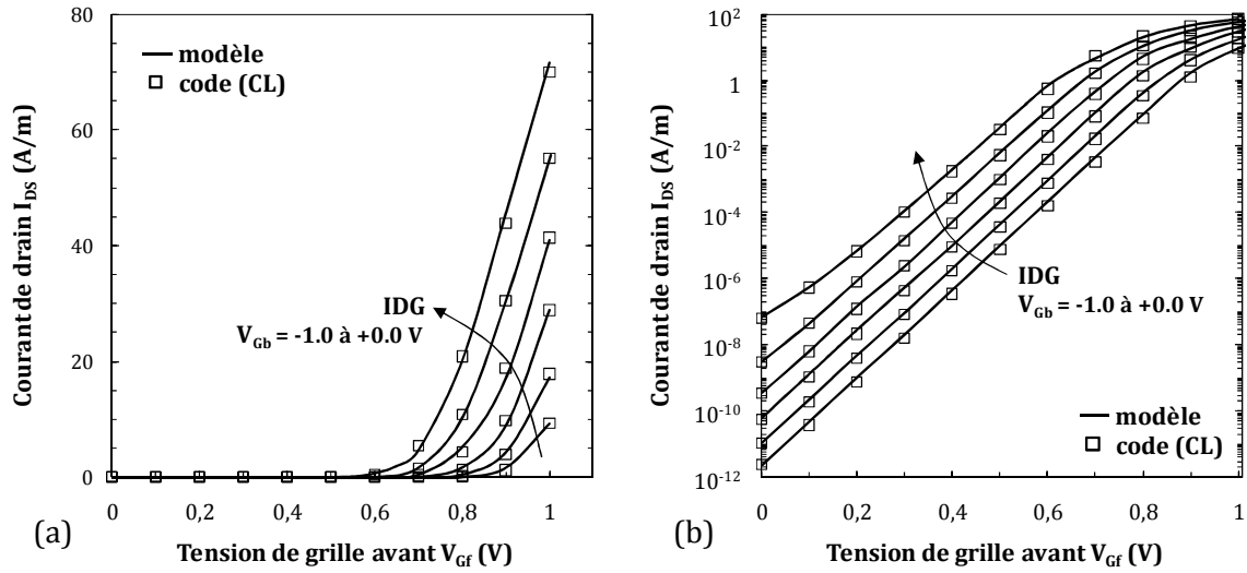
Figure 4.3 : Modèle compact (traits continus) versus simulation numérique (symboles) : caractéristiques I_{DS}(V_{Gf}) à V_D=0.1 V pour différentes valeurs négatives de la tension de la grille arrière ( V_{Gb} varie de -1 à 0 V par de pas de 0.2 V) (a) en échelle linéaire et (b) en échelle logarithmique dans le cas de transistors MOS IDG avec L_G = 200 nm, T_{Si} = 10 nm, T_{oxf} = T_{oxb} = 1 nm, N_A = n_i , N_{SD} = 3 \times 10^{20} cm -3 .
