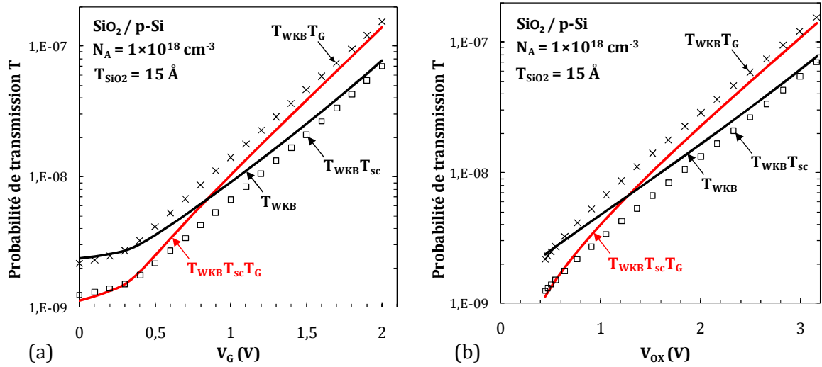
Figure 2.16 : Probabilité de transmission T des électrons du premier niveau d'énergie ( E^0 ) dans une structure M/SiO_2/p-Si avec \Phi_M = 4.05 eV, T_{SiO_2} = 15 Å, N_A = 1 \times 10^{18} cm -3 calculée selon différentes approximations : WKB [ T = T_{WKB} (trait noir)] ; WKB avec prise en compte du terme de correction côté grille [ T = T_{WKB} \times T_G (croix)] ; WKB avec prise en compte du terme de correction côté semiconducteur [ T = T_{WKB} \times T_{sc} (carrés)] ; WKB avec prise en compte des deux termes de correction [ T = T_{WKB} \times T_G \times T_{sc} (trait rouge)].
