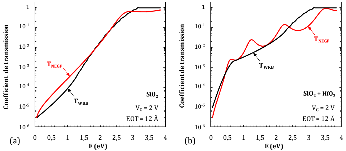
Figure 2.21 : Coefficient de transmission calculé selon l'approche WKB (noir) ou NEGF (rouge) en fonction de l'énergie des électrons à V_G = 2 \text{ V} dans des capacités MIM ( \text{EOT} = 1.2 \text{ nm} ) avec (a) une couche de \text{SiO}_2 et (b) une couche de \text{SiO}_2 ( T_{\text{SiO}_2} = 6 \text{ \AA} ) + une couche d' \text{HfO}_2 ( T_{\text{HfO}_2} = 30.8 \text{ \AA} ).
