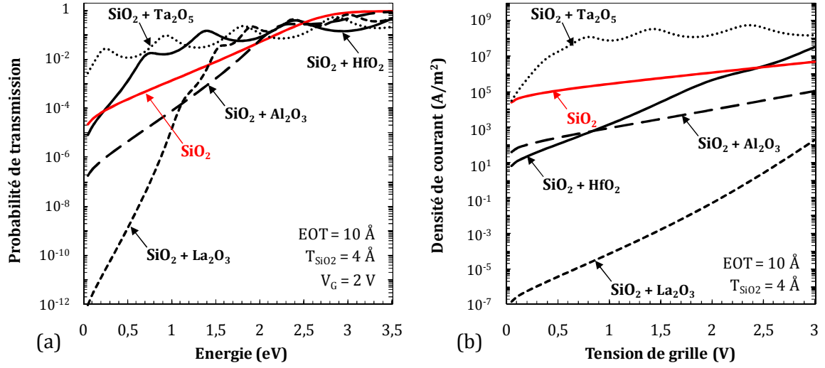
Figure 2.26 : Comparaison de capacités MIM avec différents empilements de grille [ SiO_2 ( T_{SiO_2} = EOT , rouge), SiO_2 + HfO_2 ( T_{HfO_2} = 30.8 \text{ \AA} , traits continus), SiO_2 + Al_2O_3 ( T_{Al_2O_3} = 13.9 \text{ \AA} , pointillés larges), SiO_2 + La_2O_3 ( T_{La_2O_3} = 43.1 \text{ \AA} , pointillés courts), SiO_2 + Ta_2O_5 ( T_{Ta_2O_5} = 40.0 \text{ \AA} , points)] et le même EOT = 10 \text{ \AA} ( T_{SiO_2} = 4 \text{ \AA} pour les structures à deux couches,) en terme de (a) coefficient de transmission des électrons vs énergie à V_G = 2 \text{ V} et (b) densité de courant de fuite vs tension de grille (calcul avec la transparence NEGF).
