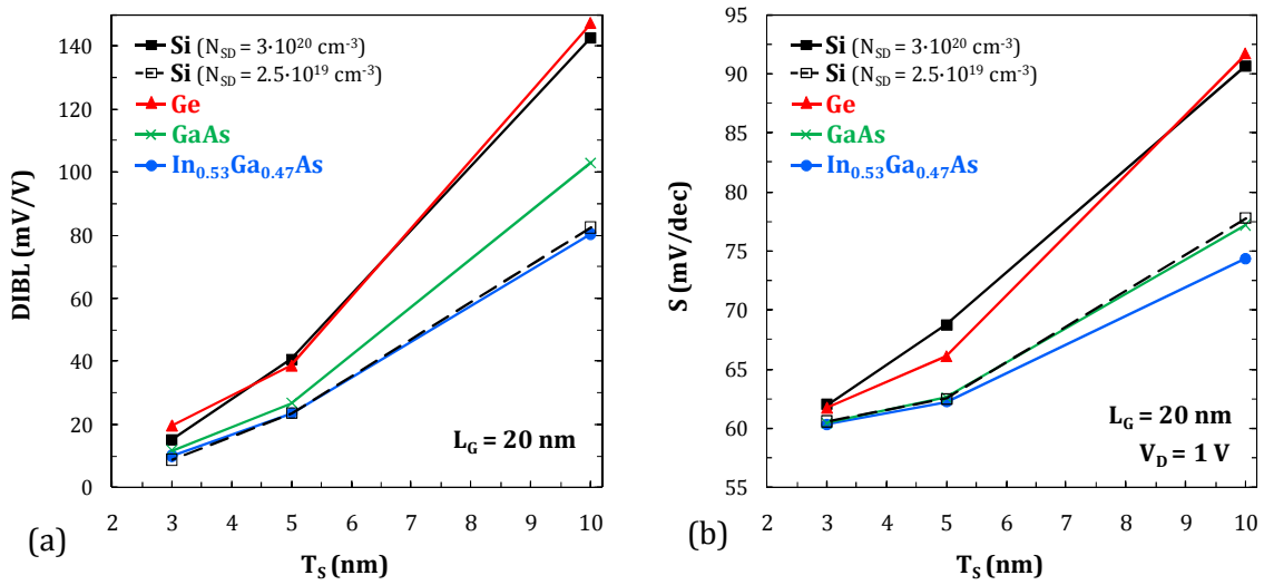
Figure 3.14 : Représentation (a) de l'effet de canal court DIBL et (b) de la pente sous le seuil SS en fonction de l'épaisseur de film T_S dans les transistors MOS DG ( L_G = 20 nm et simulation quantique ) avec différents matériaux semiconducteurs (même code couleur que la figure 3.13). Le cas d'un transistor MOS DG à base de Si avec des régions S/D moins dopées ( N_{SD} = 2.5 \cdot 10^{19} \text{ cm}^{-3} ) est également représenté en pointillés.
