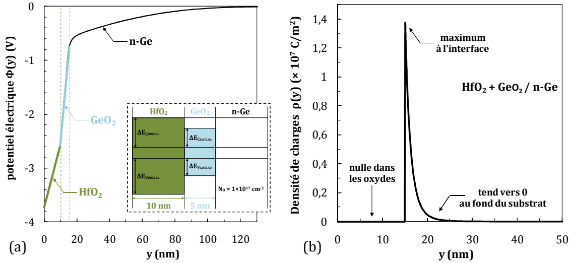
Figure 2.6 : (a) Potentiel électrique \Phi(y) et (b) densité de charges \rho(y) d'une structure \text{HfO}_2+\text{GeO}_2/\text{n-Ge} [avec T_{\text{HfO}_2} = 10 nm, T_{\text{GeO}_2} = 5 nm, N_D = 10^{17} \text{ cm}^{-3} , voir encart de la figure (a)] dans le régime d'inversion forte ( V_G \ll 0 V). L'origine de l'axe horizontal est prise au contact métal/oxyde.
