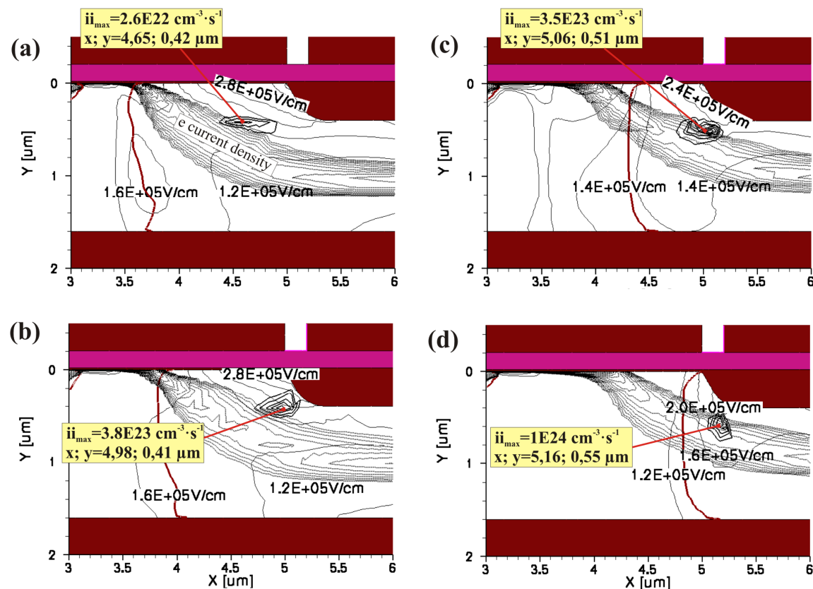
Figure II-24 : Densité de courant d'électrons, contour du champ électrique et de la concentration de porteurs ionisés dans la structure STI-LDMOS à V_{\text{GS}} = 2 \text{ V} et V_{\text{DS}} = 60 \text{ V} pour \Delta\text{Wells} égal à (a) 0, (b) 0,5, (c) 1 et (d) 1,5 \mu\text{m}
