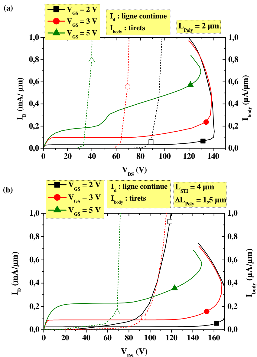
Figure II-25 : Comparaison des caractéristiques de sortie des (a) transistor LDMOS avec L_{\text{Poly}} = 2 \mu\text{m} et (b) STI-LDMOS avec L_{\text{STI}} = 4 \mu\text{m} et \Delta L_{\text{Poly}} = 1,5 \mu\text{m}
