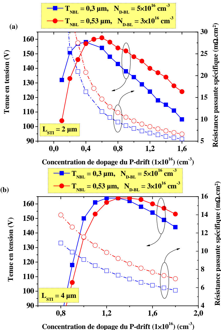
Figure III-8 : Tenue en tension et résistance passante spécifique du transistor RESURF-PLDMOS avec (a) L_{STI} = 2 \mu\text{m} et (b) L_{STI} = 4 \mu\text{m}
