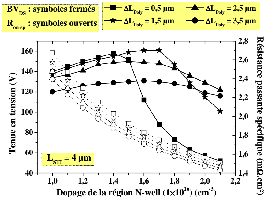
Figure II-5 : Tenue en tension et résistance passante spécifique du transistor STI-LDMOS avec L_{STI} = 4 \mu\text{m} pour plusieurs valeurs de \Delta L_{Poly}
