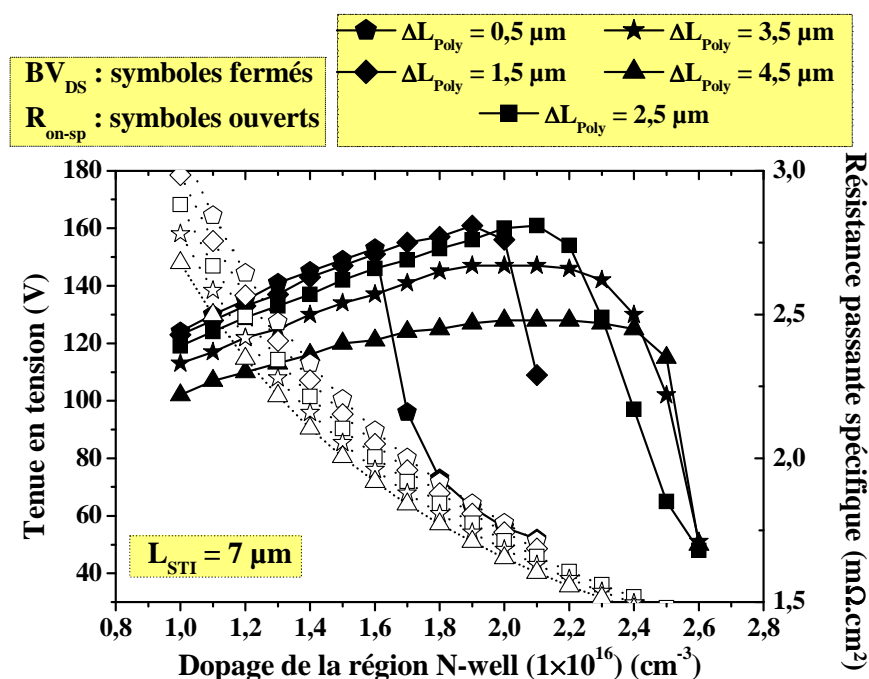
Figure II-6 : Tenue en tension et résistance passante spécifique du transistor STI-LDMOS avec L_{STI} = 7 \mu\text{m} pour plusieurs valeurs de \Delta L_{Poly}
