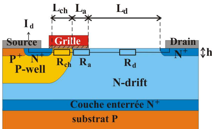
Figure I-11 : Coupe schématique du transistor LDMOS
