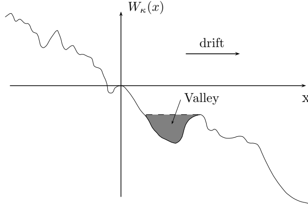
Figure 1.3: Une vallée.
