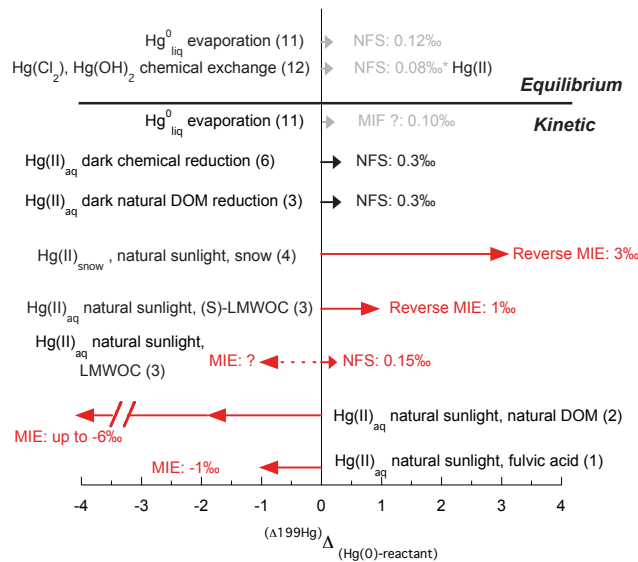
Figure 27: Variation de l'amplitude du facteur de fractionnement isotopique des anomalies en ^{199}\text{Hg} exprimé en (\Delta^{199}\text{Hg})_{\Delta(\text{Hg}(0)\text{-reactant})} mesuré dans les différents travaux expérimentaux pour les réactions cinétiques et équilibres: les références de la littérature sont identiques à celle de la figure 26
