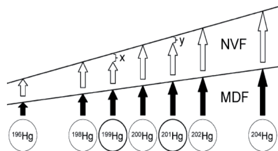
Figure 20: Représentation schématique des mécanismes de fractionnement isotopique du mercure. MDF représente le fractionnement dépendant de la masse et NVF représente le fractionnement dû au NFS. x et y dans le NFS sont deux quantités mesurables permettant d'identifier le fractionnement NFS par rapport au MDF. (Extrait de Wiederhold et al., 2010).
