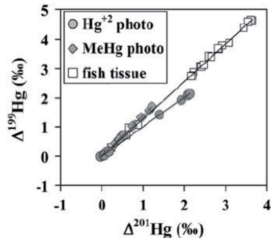
Figure 31: \Delta^{199}\text{Hg} (‰) en fonction de \Delta^{201}\text{Hg} (‰) pour les expériences de photoréduction du Hg(II) et du MeHg. Dans ce diagramme, la pente des anomalies \Delta^{199}\text{Hg}/\Delta^{201}\text{Hg} est de 1 pour la photoréduction du Hg(II) et de 1.3 pour le MeHg (Extrait de Bergquist and Blum, 2007).
