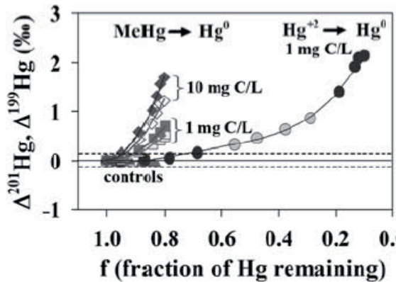
Figure 30: \Delta^{201}\text{Hg} (‰) et \Delta^{199}\text{Hg} (‰) en fonction de la fraction de mercure restant en solution pour les expériences de photoréduction du Hg(II) et du MeHg (Extrait de Bergquist and Blum, 2007).
