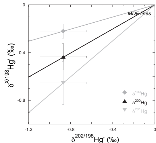
Figure 16 : Diagramme tri-isotopique présentant les \delta^{xxx/198}\text{Hg} en fonction du \delta^{202/198}\text{Hg} . Dans ce diagramme, les droites représentées sont les droites de fractionnement de masse calculées avec l'équation [8].
