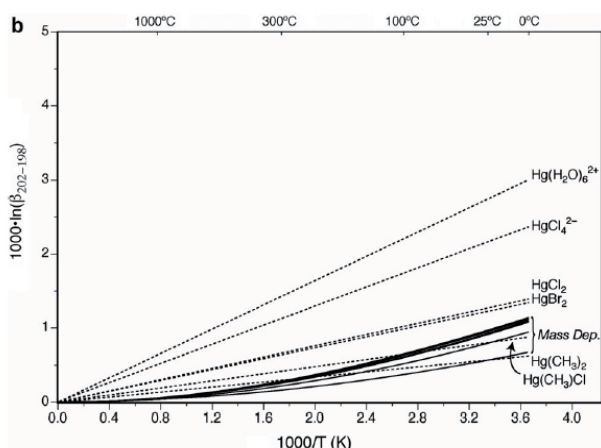
Figure 22: Dans ce diagramme le facteur de fractionnement entre le Hg(0) et les différents composés du mercure ( ^{202/198}\Delta_{\text{Hg}(0)\text{-HgX}} (en ‰), équivalent à 1000\ln(\beta_{202-198}) ) est tracé en fonction de 1000/T . L'amplitude des fractionnements dépendants de la masse pour chacune des espèces est en trait plein noir. L'amplitude des fractionnements dus au NFS sont tracés en trait pointillés noir. Ce diagramme montre par exemple que, à 25°C l'amplitude de fractionnement due au NFS est au moins égale à celle du fractionnement dépendant de la masse pour les espèces \text{Hg}(\text{CH}_3)_2 et \text{Hg}(\text{CH}_3)\text{Cl} et qu'elle est plus importante pour les autres espèces. (Extrait de Schauble 2007)
