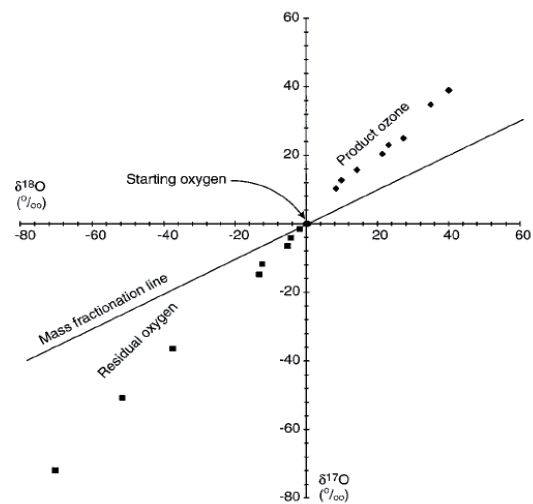
Figure 17 : Diagramme tri-isotopique de l'oxygène avec \delta^{17}O en fonction de \delta^{18}O pour la réaction de formation de l'ozone. Dans ce diagramme, la droite de fractionnement de masse (mass fractionation line) est représentée. Les compositions isotopiques de l'ozone produit et de l'oxygène restant à la fin de la réaction montrent des déviations significatives de cette droite de fractionnement de masse indiquant des fractionnements indépendants de la masse (MIF). (Extrait de Thiemens, 1999).
