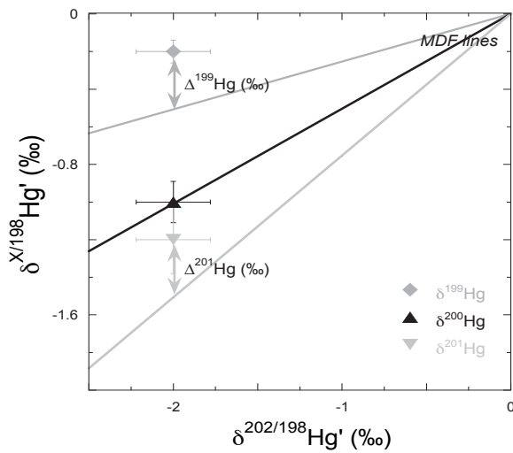
Figure 18: Diagramme tri-isotopique dans lequel est représenté le \delta^{XXX}\text{Hg} en fonction du \delta^{202}\text{Hg} ainsi que les droites de fractionnement de masse. Dans ce diagramme les \delta^{199}\text{Hg} et \delta^{201}\text{Hg} présentent des déviations significatives de leur droite de fractionnement de masse respective contrairement au \delta^{200}\text{Hg} . Ces déviations indiquent des fractionnements indépendants de la masse (MIF) sur les isotopes ^{199}\text{Hg} et ^{201}\text{Hg} . La grandeur de mesure de ces MIF est le \Delta^{XXX}\text{Hg} (où XXX est ^{199}\text{Hg} ou ^{201}\text{Hg} ) et représente la différence entre le \delta^{XXX}\text{Hg} mesuré et le même \delta^{XXX}\text{Hg} s'il était dépendant de la masse (voir calcul dans le texte).
