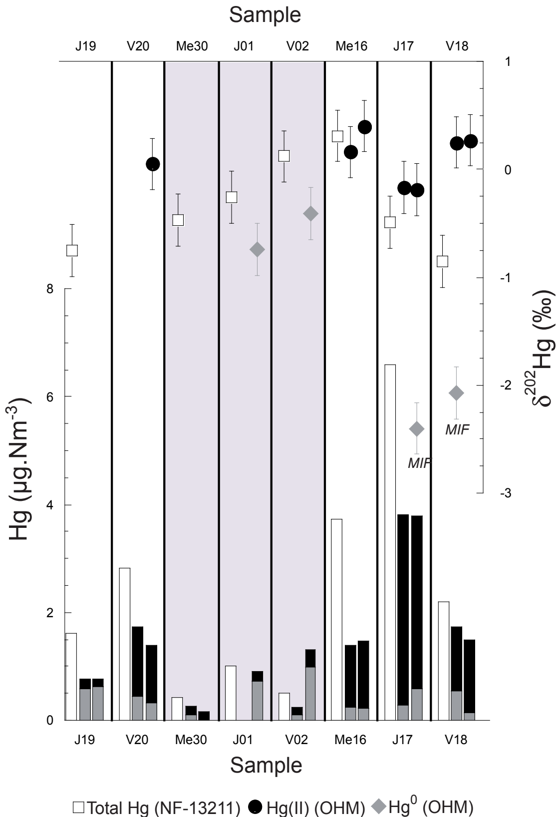
Figure 6: En bas , Concentration en Hg total, Hg(II) et Hg 0 en \mu\text{g}\cdot\text{Nm}^{-3} pour les méthodes NF-13211, OHM-1&2 pour les 3 campagnes d'échantillonnage: mai 2009 (J19, V20), octobre 2009 (Me30, J01, V02), décembre 2009 (Me16, J17, V18). Dans les méthodes OHM, la somme Hg(II) + Hg 0 représente le Hg total. En haut , les compositions isotopiques ( \delta^{202}\text{Hg} ) du Hg total et des formes Hg(II) et Hg 0 pour les 3 campagnes d'échantillonnage (MIF signifie «mass independent fractionation»).
