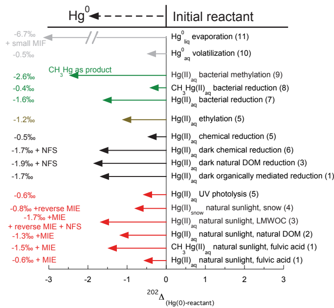
Figure 26: Variation de l'amplitude du facteur de fractionnement isotopique sur le rapport ^{202/198}\text{Hg} exprimé en ^{202}\Delta_{(\text{Hg}(0)\text{-reactant})} mesuré dans les différents travaux expérimentaux pour les réactions cinétiques: (1) Bergquist and Blum (2007) (2) Zheng and Hintelmann (2009), (3) Zheng et Hintelmann (2010a), (4) Sherman et al. (2010), (5) Yang and Sturgeon (2008), (6) Zheng and Hintelmann (2010), (7) Kritee et al. (2007, 2008), (8) Kritee et al., (2009), (9) Rodriguez et al., (2009), (10) Zheng et al., (2007), (11) Estrade et al., (2009). Dans le cas où des fractionnements indépendants de la masse ont été mis en évidence, le type MIE ou NFS est reporté. Mise à jour de Bergquist and Blum, (2009)
