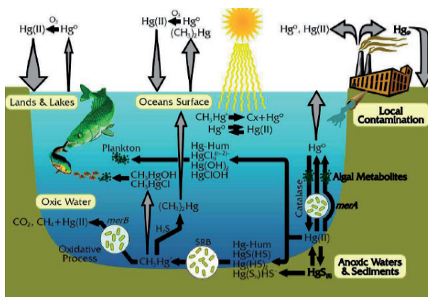
Figure 2: Cycle biogéochimique axé sur les transformations du mercure inorganique ( Hg(0) , Hg(II) ) en méthylmercure ( CH_3Hg et ses autres composés) dans les systèmes aquatiques (Extrait de Scheafer et al., 2002)
