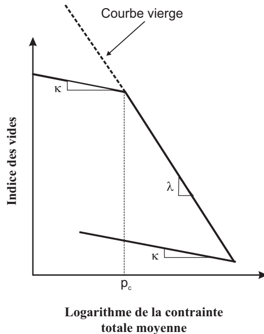
FIG. 7.2 – Consolidation mécanique.
