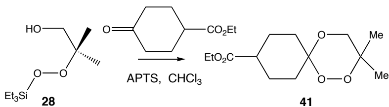
Figure 20 : synthèse du diméthyltrioxane 41 .
