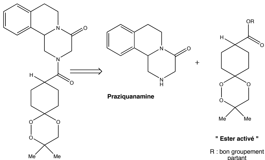
Figure 19 : Rétrosynthèse du diméthyltrioxaquantel acylé en position 2.
