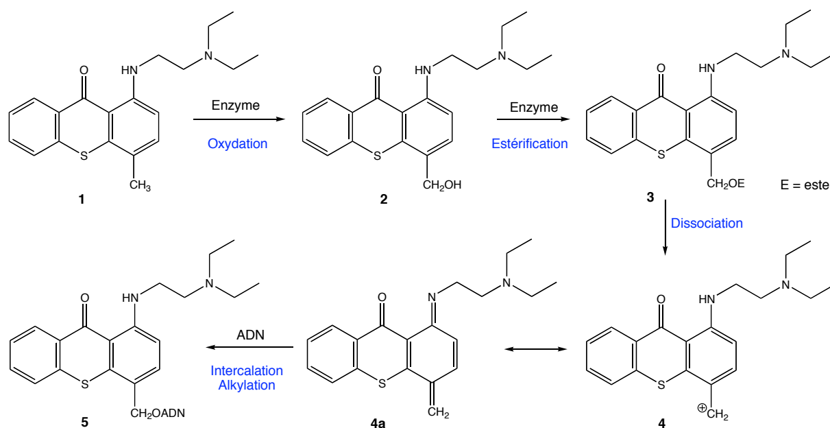
Figure 4 : Proposition d'un mécanisme d'action pour l'hycanthonne et la lucanthonne [38].
