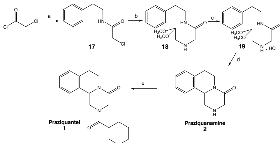
Figure 8 : Synthèse du praziquantel 1 selon la méthode de Kim et al. [7] : a) phényléthylamine, NaHCO 3 , CH 2 Cl 2 , TA, 2h, 92% ; b) aminoacétaldéhyde diméthylacétal, toluène, reflux, 2h ; c) HCl gaz, rendement des étapes b et c 67% ; d) H 2 SO 4 concentré, TA, 3,5h, 98% ; e) C 6 H 11 CHCl, Na 2 CO 3 , DCM, TA, 2h, 85%.
