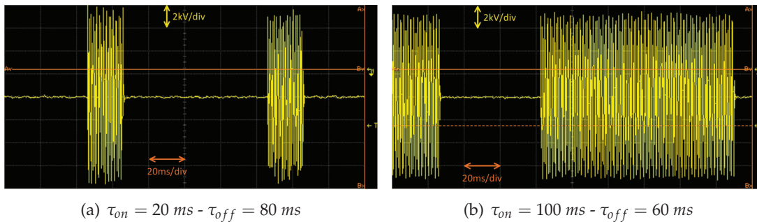
FIGURE 3.14 – Oscillogrammes de tension typiques obtenus avec le G2000 pour différents temps de maintien et de relaxation
