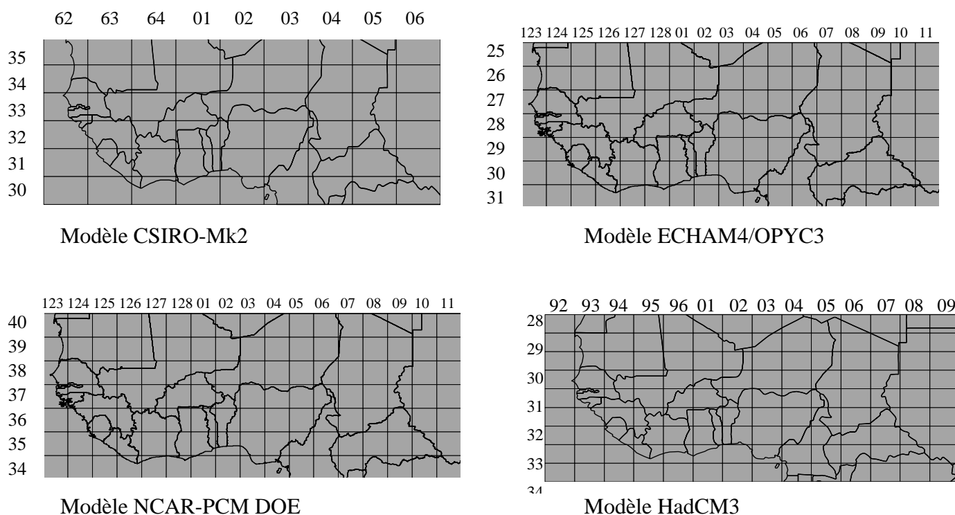
Figure 4.12 – Superposition des grilles propres à chaque modèle climatique sur la fenêtre étudiée.
