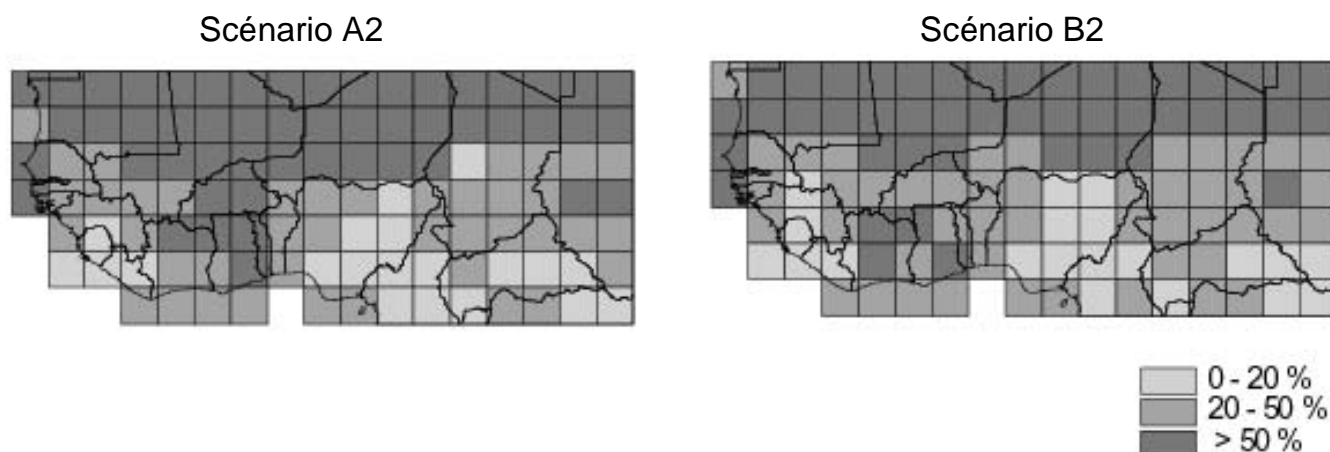
Figure 4.15 – Exemple de cartes d'erreurs relatives sur les précipitations moyennes annuelles entre 1990-1998, pour le modèle ECHAM4 avec les scénarii A2 et B2.
