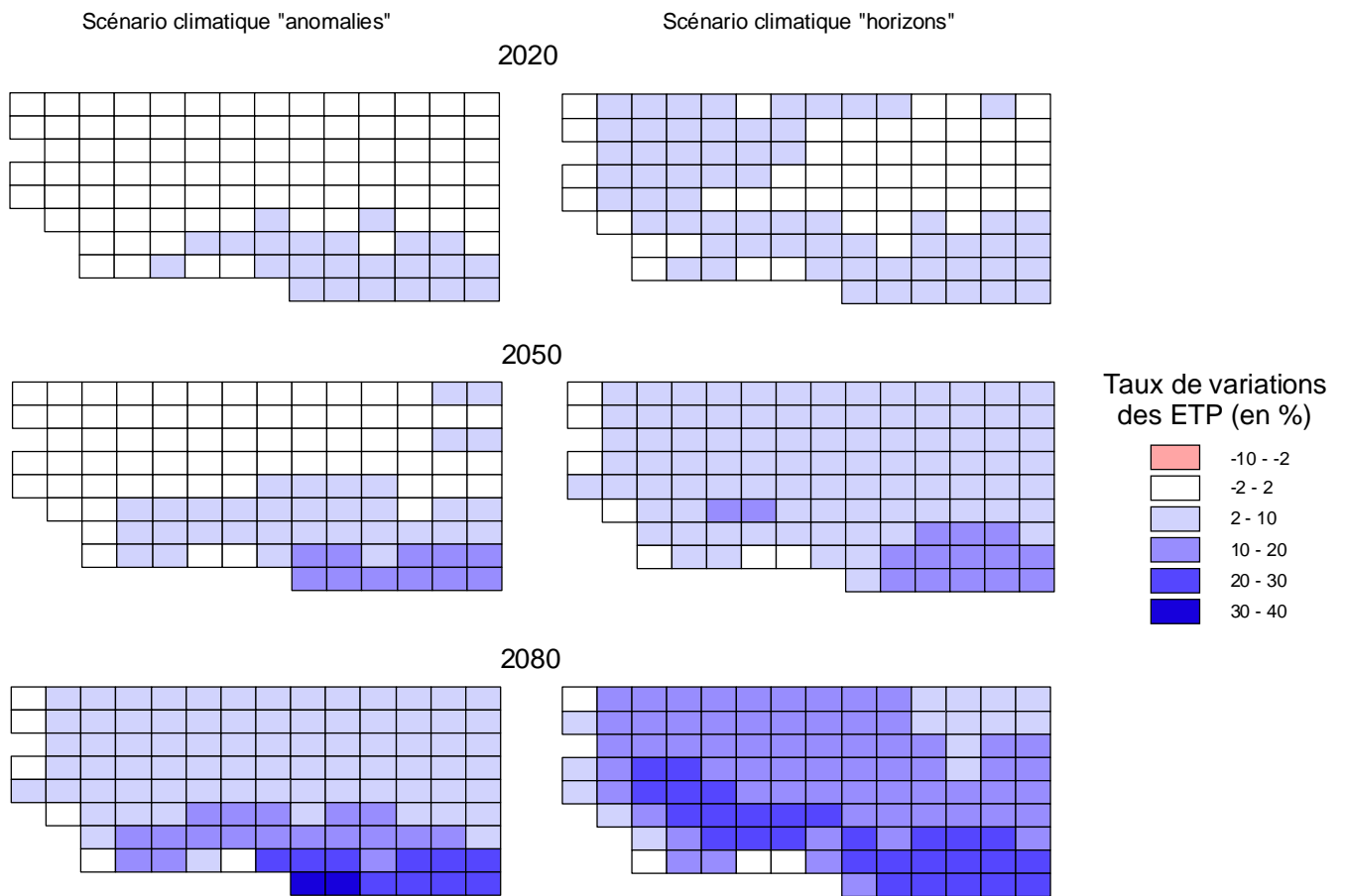
Figure 5.1 – Variations des ETP Ano (à gauche) et ETP Horiz (à droite) pour les horizons 2020, 2050 et 2080 par rapport à la moyenne 1966-1995 observée.
