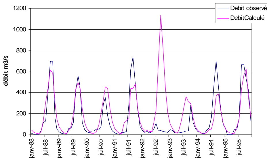
Figure 3.33 – Comparaison des hydrogrammes observés et calculés par le modèle GR2M en validation sur la période 1988-1995, pour Batafango (Chari).
