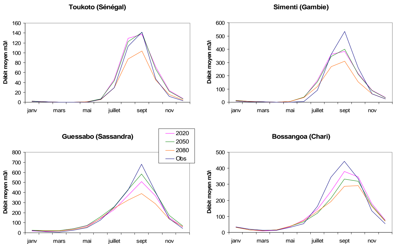
Figure 5.22 – Hydrogrammes moyens aux horizons 2020, 2050 et 2080, comparés à celui de référence (1971-1955), des séries GR2M_Ano pour quatre bassins versants représentatifs de chaque unité hydrographique étudiée pour le cas 1.
