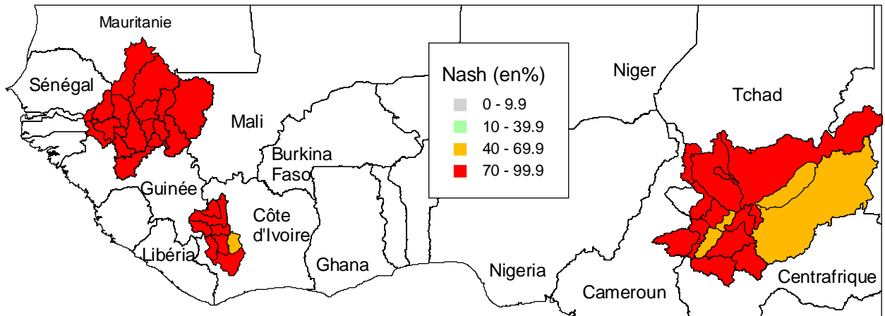
Figure 3.29 – Cartographie des critères de Nash obtenus en calage avec le modèle GR2M
