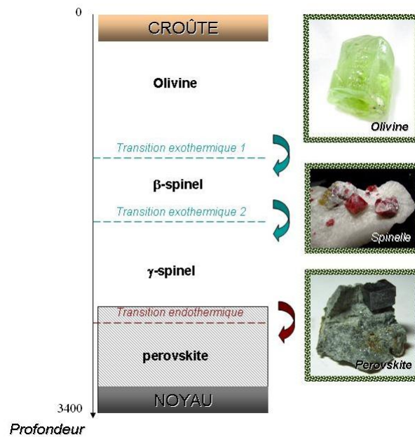
FIGURE 1.13 – Structure interne de Mars schématisée, avec les minéraux suivants illustrés : l’Olivine, la Spinnelle et la Perovskite. Les transitions de phase sont indiquées approximativement dans le manteau car leurs positions ne sont pas connues précisément, et celle de la transition endothermique dépend de la taille du noyau. Les modèles de structure interne employés dans les simulations numériques seront décrits dans le chapitre 3.
