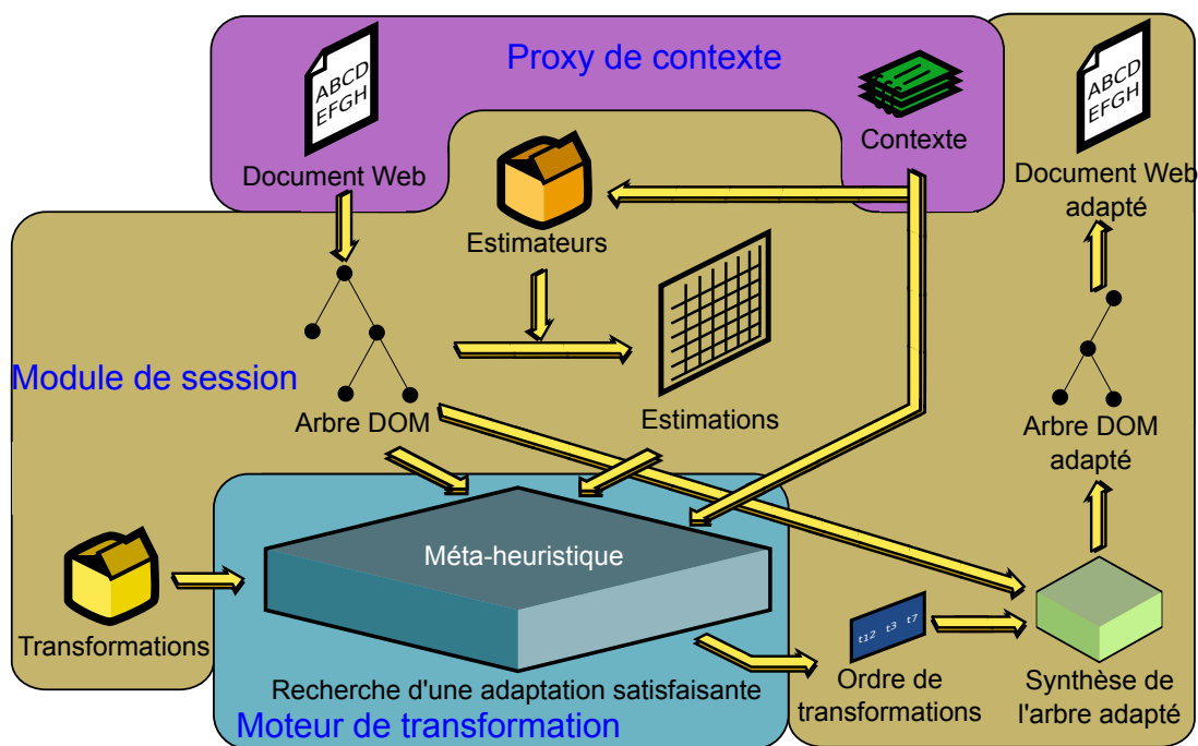
FIG. II.3 – Blocs de notre système au niveau du processus d'adaptation.
