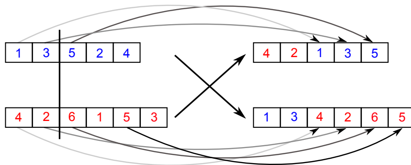
FIG. II.10 – Croisement d'individus avec locus = 2.
