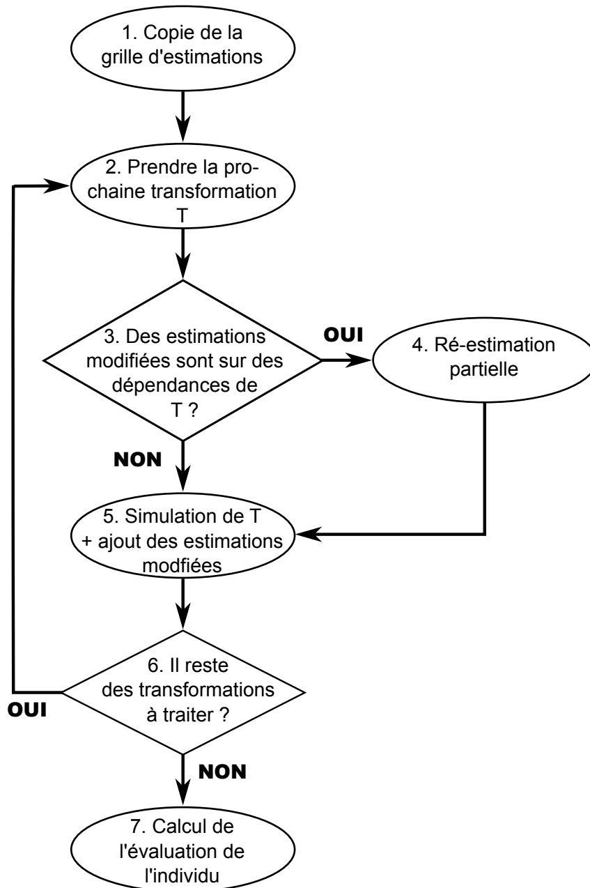
FIG. II.11 – Processus d'évaluation d'un individu.
