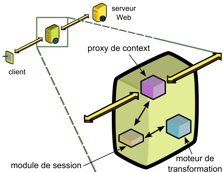
FIG. II.2 – Schéma bloc de notre système.
