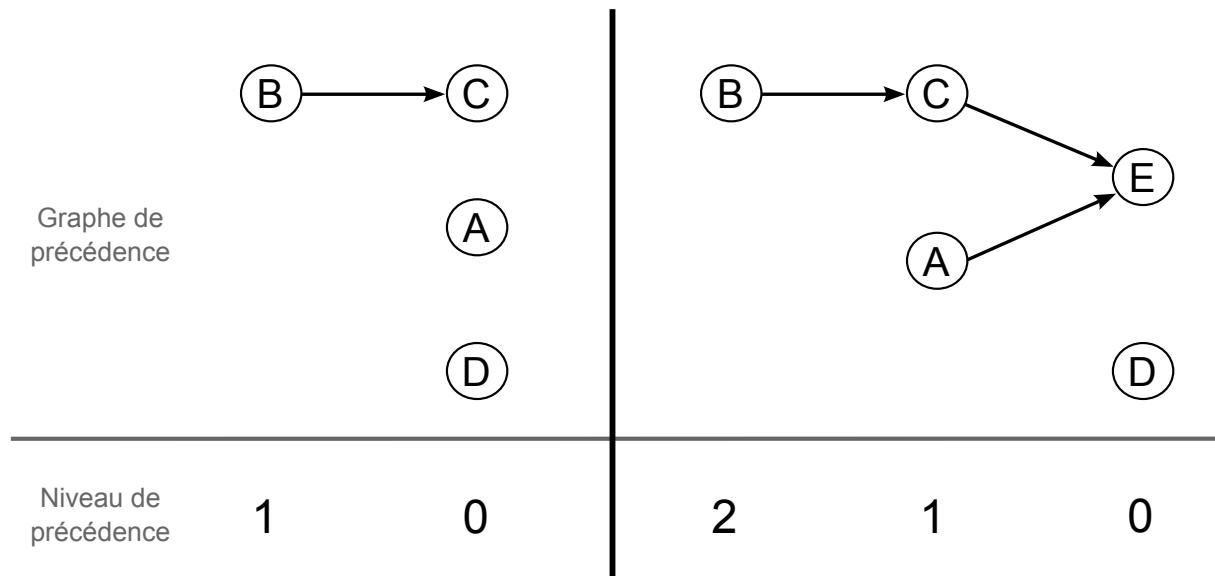
FIG. II.7 – Graphe de précedence avant (à gauche) et après (à droite) l'ajout de l'estimateur E dépendant de A et C.
