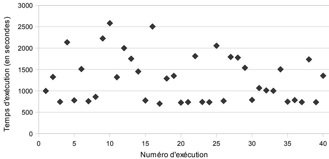
FIG. III.6 – Temps d'exécution de l'algorithme génétique pour les exécutions de la première expérimentation.
