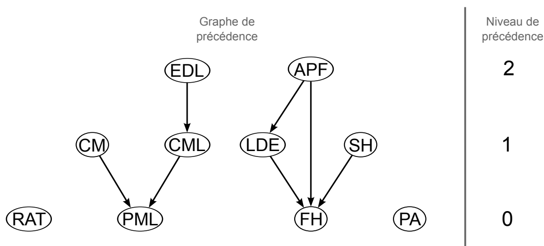
FIG. III.1 – Graphe de précédence des estimateurs développés avec niveau de précédence.
