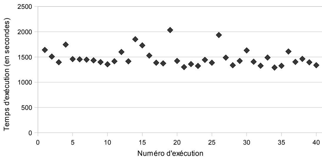
FIG. III.7 – Temps d'exécution de l'algorithme génétique pour les exécutions de la seconde expérimentation.
