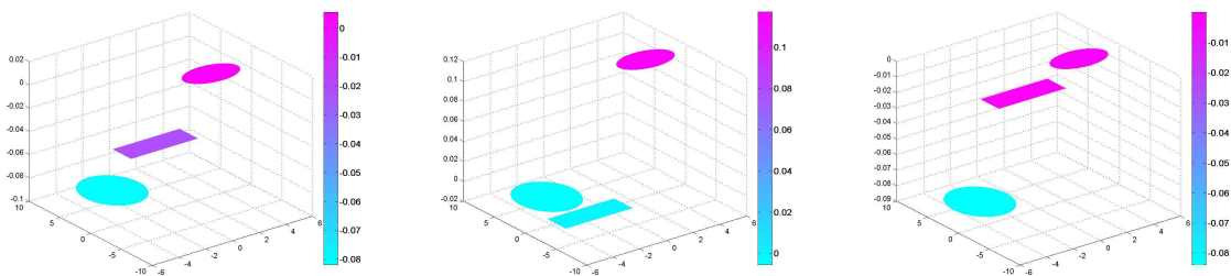
(d) Premier vecteur propre de A (e) Deuxième vecteur propre de A (f) Troisième vecteur propre de A
