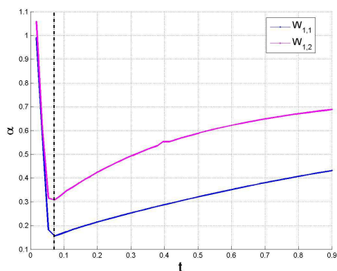
(b) Norme \alpha en fonction de t
