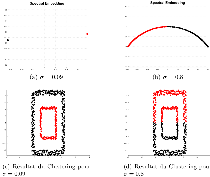
FIGURE 1.2 – Influence du paramètre dans l'espace de projection spectrale
