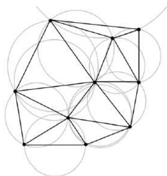
(a) Triangulation de Delaunay et cercles circonscrits
