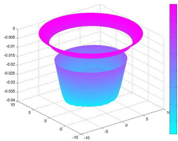
(d) Produit (A + \mathbb{I}_N)MV_{1,1}
