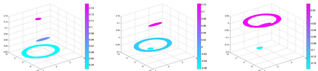
(a) Première fonction propre de (\mathcal{P}_\Omega^N) (b) Deuxième fonction propre de (\mathcal{P}_\Omega^N) (c) Troisième fonction propre de (\mathcal{P}_\Omega^N)
