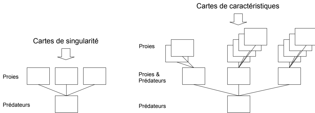
FIGURE 7.4.1: Prise en compte des cartes de caractéristiques dans le modèle proies / prédateurs. A gauche : la hiérarchie utilisée actuellement par notre modèle ; les proies sont associées aux cartes de singularité. A droite : une hiérarchie basée sur les cartes de caractéristiques ; on ajoute un étage au système proies / prédateurs, les cartes de singularité sont remplacées par les proies du niveau central (également prédatrices des proies du niveau supérieur).
