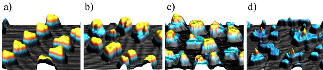
FIGURE 3.9 – Images STM 30 \times 30 \text{ nm}^2 , les teintes bleutées correspondent à la 1 re couche et le jaune à la 2 e couche. (a) Cobalt pur (b) Co 81 Pt 19 (c) Co 58 Pt 42 (d) Platine pur .
