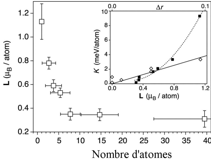
FIGURE 1.21 – Moment magnétique orbital en fonction du nombre moyen d'atomes composant des agrégats de cobalt déposés sur une surface de platine (111). En encart, évolution de l'anisotropie magnétique en fonction du moment orbital (axe du bas et carrés pleins) ou d'une quantité proportionnelle à l'anisotropie du moment orbital (axe du haut et losanges vides). L'évolution en fonction de l'anisotropie du moment se fait linéairement (courbe en trait plein), en accord avec l'équation (1.10) (figure extraite de [Gambardella, 2003]).
