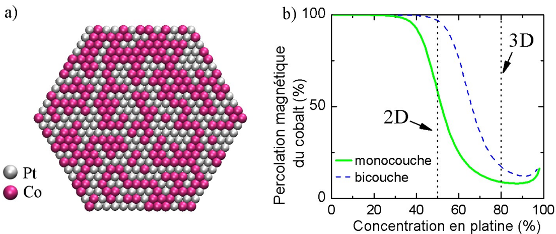
FIGURE 5.11 – (a) Îlot monocouche Co_{50}Pt_{50} avec 469 atomes (233 atomes de cobalt et 236 de platine) répartis aléatoirement. (b) Taux de percolation des atomes de cobalt en fonction de la composition en platine pour des îlots de configuration monocouche (469 atomes, ligne pleine) et bicouche (409 atomes dont 217 en première couche, ligne discontinue). L'ordonnée représente la proportion moyenne d'atomes de cobalt appartenant au plus gros agrégat de cobalt. Les cas infinis 2D et 3D sont rappelés par les droites en pointillé.
