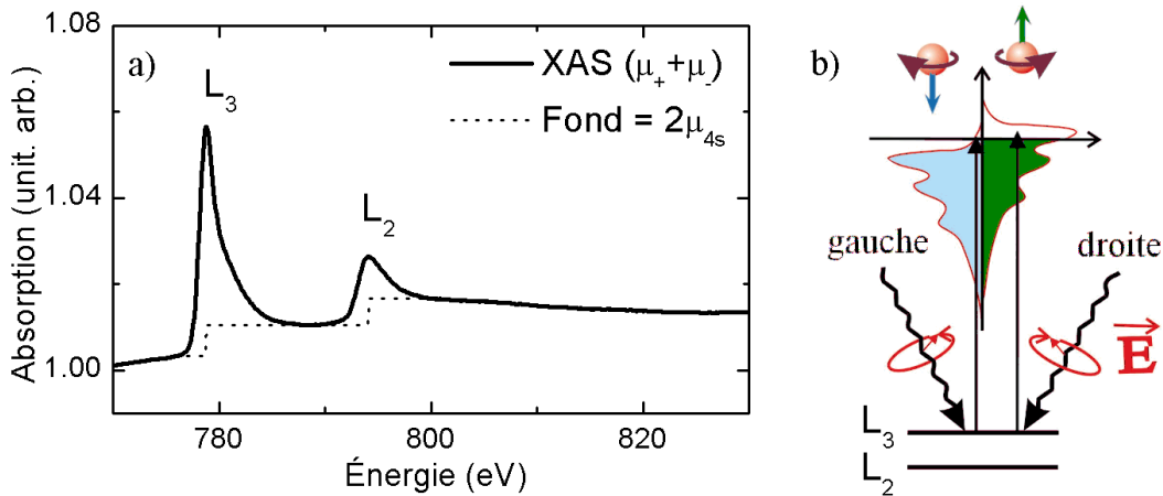
FIGURE 2.5 – (a) Spectre d'absorption d'un faisceau non polarisé (moyenne des faisceaux polarisés) obtenu sur des nanostructures Co_{84}Pt_{16} avec \theta = 0,31 MC à 150K. (b) Schéma du principe de l'absorption de photons polarisés par un niveau 2p_{3/2} vers des états vides 3d .
