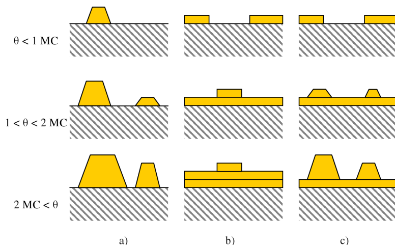
FIGURE 1.5 – Représentation schématique des différents modes de croissance à l'équilibre d'un adsorbant sur une surface en fonction du taux de couverture : (a) Croissance tridimensionnelle ou « Volmer - Weber », (b) Croissance bidimensionnelle ou « Frank - van der Merwe », (c) Croissance « Stranski - Krastanov ».
