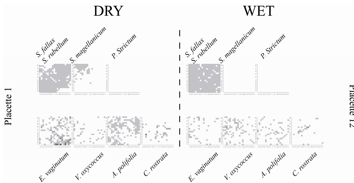
Figure 1.5 : Composition végétale des placettes en conditions DRY (placette 1) et WET (placette 12). Relevé floristique effectué en 2008 (Buttler 2008)
