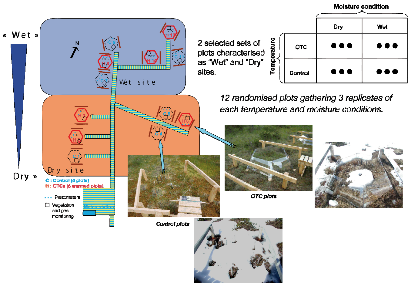
Figure I.4 : Dispositif expérimental et vues des placettes-témoins et les placettes équipées d'OTCs (Laggoun-Déforge 2008)
