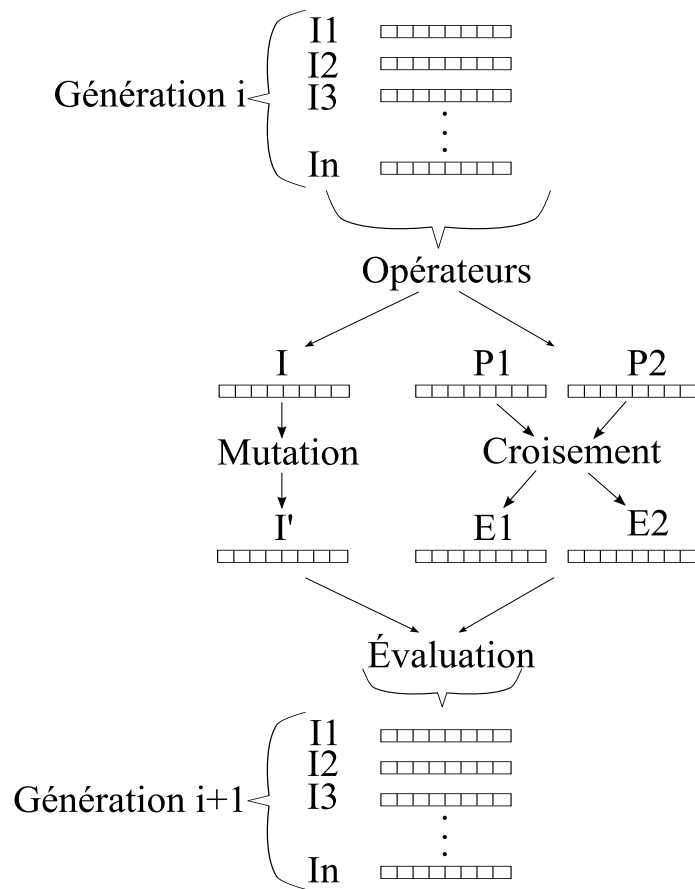
FIGURE 2.1 – Principe général d'un algorithme génétique
