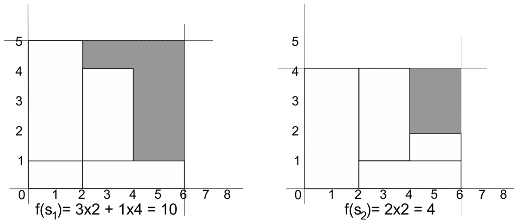
FIGURE 2.6 – Fonctions d’évaluation reposant sur le critère d’aire gaspillée
