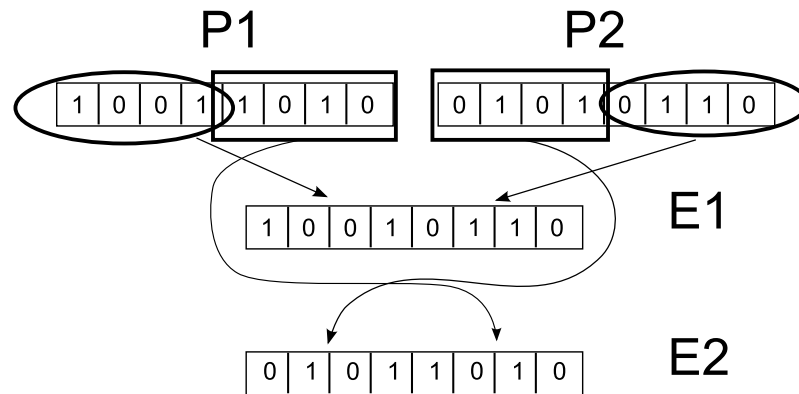
FIGURE 2.3 – Exemple de l’opérateur de croisement créé par Holland
