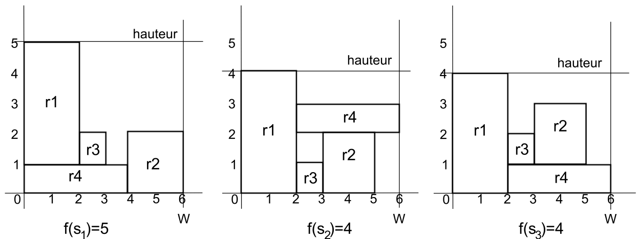
FIGURE 2.5 – Fonctions d'évaluation reposant sur le critère de hauteur
