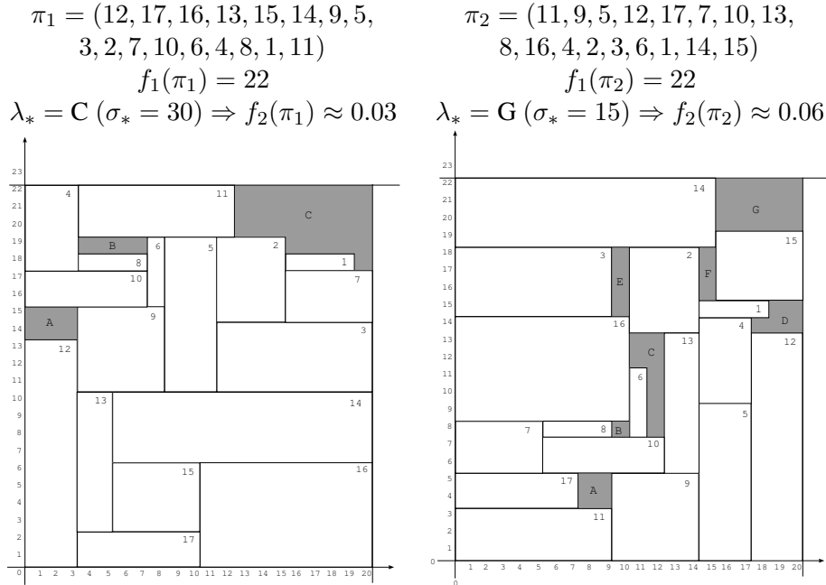
FIGURE 2.12 – Pour deux individus \pi_1 (à gauche) et \pi_2 (à droite) tels que f_1(\pi_1) = f_1(\pi_2) , f_1 n’est pas capable de faire la différence, donc si nous appliquons f_2 , \pi_1 est meilleur que \pi_2 ( f_2(\pi_1) < f_2(\pi_2) ).
