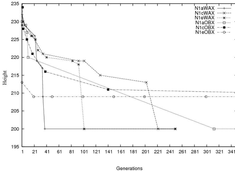
FIGURE 2.14 – Comparaison entre les croisements WAX et OBX
