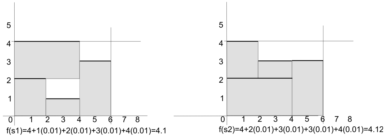
FIGURE 2.7 – Fonctions d’évaluation reposant sur la distribution des rectangles
