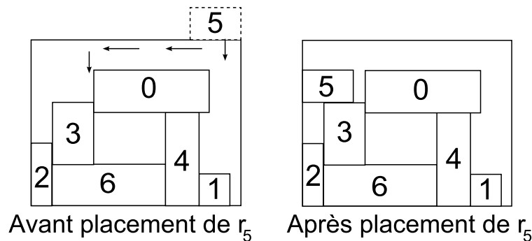
FIGURE 1.10 – Un exemple d'exécution de BL
