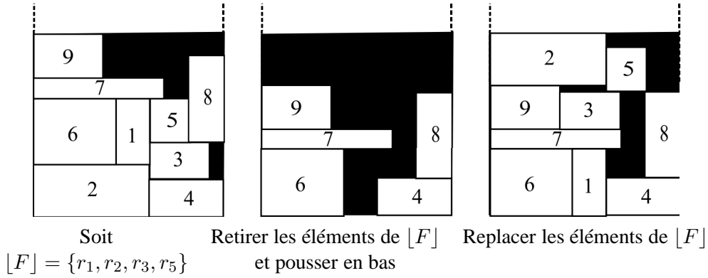
FIGURE 4.2 – La diversification D_T . Les expériences ont montré que presque tous les rectangles de basses fréquences ( F_i ) se situent dans le bas de la bande.
