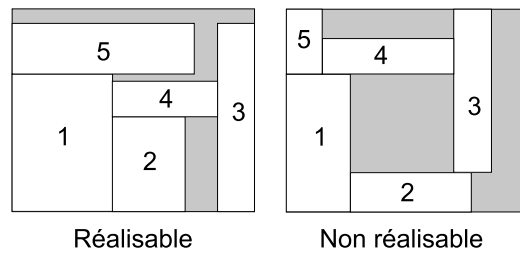
FIGURE 1.3 – La contrainte de découpe guillotine
