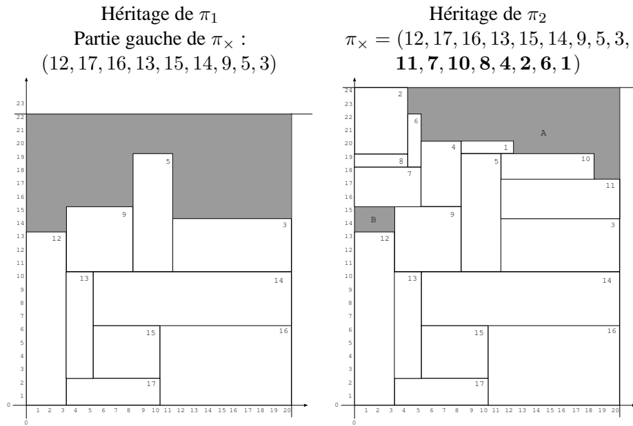
FIGURE 2.13 – WAX : un exemple (avec les parents de la figure 2.12).
