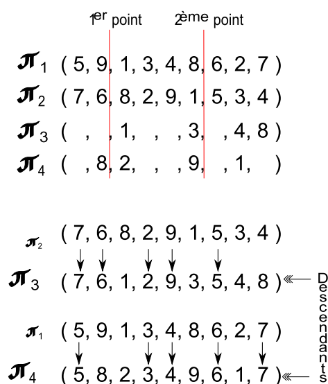
FIGURE 2.9 – Une illustration du croisement OBX
