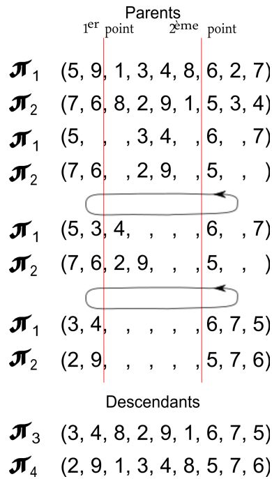
FIGURE 2.8 – Une illustration du croisement OX
