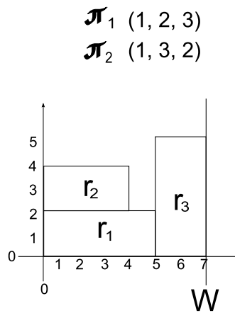
FIGURE 2.4 – Deux permutations avec le même patron de placement selon BL
