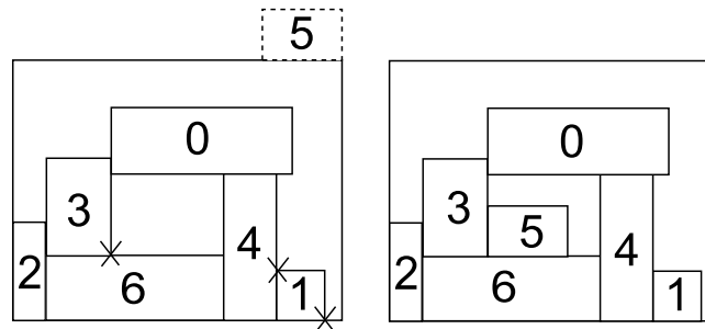
FIGURE 1.11 – Un exemple d’exécution de BLF
