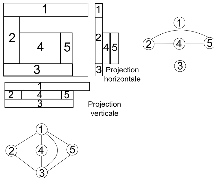
FIGURE 1.8 – Représentation par graphes d’intervalles
