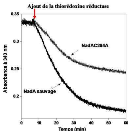
Figure 76 : Dosage des ponts disulfure dans NadA E. coli par le système Trx/Trr/NADPH. Mesure réalisée à 340 nm dans une cuve de 1 mm en incubant les protéines NadA (145 \mu M) avec du NADPH (0.3 mM), de la Trx (1 \mu M) dans du Tampon H. Après 8 minutes, la Trr (0.23 \mu M) est ajoutée et la réaction suivie sur 50 minutes. La trace inférieure représente les résultats obtenus avec la protéine NadA sauvage, la trace supérieure représente le résultat obtenu pour la protéine mutée NadAC294A, des tracés similaires ont été obtenus pour les protéines NadAC291A et NadAC291A-C294A.
