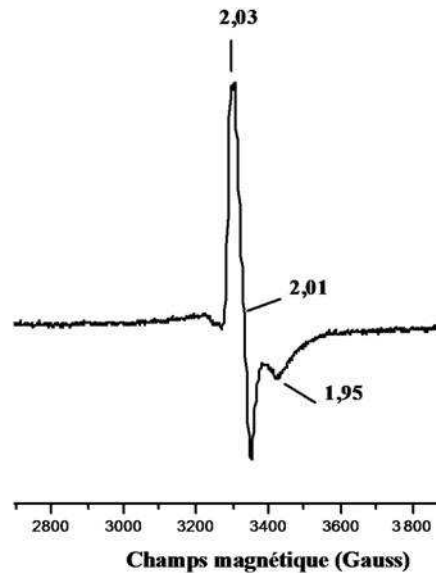
Figure 52 : Spectre RPE de NadA d' E. coli (260 \mu\text{M} ) exposée pendant 10 min à l'oxygène. Enregistré à 10 K, puissance 0.1 mW, amplitude de modulation 10 Gauss, gain 2 \cdot 10^5 .
