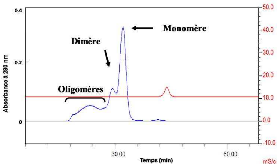
Figure 49 : Détermination de l'état oligomérique de la NadA d' E. coli . Profil d'élution obtenu sur Superdex-200 de la NadA d' E. coli (200 \mu M) réalisé à 0.5 mL/min dans du Tampon Tris -HCl 100 mM pH 7.5, NaCl 100 mM.
