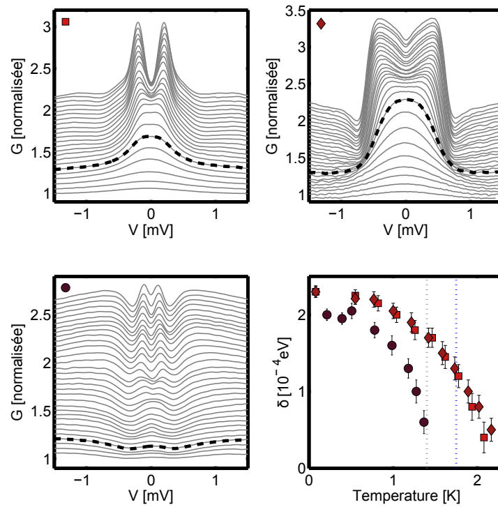
Figure 7.9 Dépendance en température de la conductance différentielle G obtenue à différentes positions sur les échantillons \text{InO}_{x-2} ( \circ ) et \text{InO}_{x-3} ( \square, \diamond ). Les spectres sont décalés verticalement d'une valeur constante par souci de clarté. Les spectres obtenus à T = T_c sont représentés en pointillés noirs. En bas à droite : évolution de l'énergie d'Andreev \delta(T) . Les lignes pointillées verticales indiquent les températures critiques respectives 1.4 K et 1.75 K des deux échantillons. Les barres d'erreurs correspondent à l'indétermination sur les valeurs de \delta extraites à partir des ajustements théoriques. Celles-ci augmentent avec la température à cause de l'élargissement thermique.
